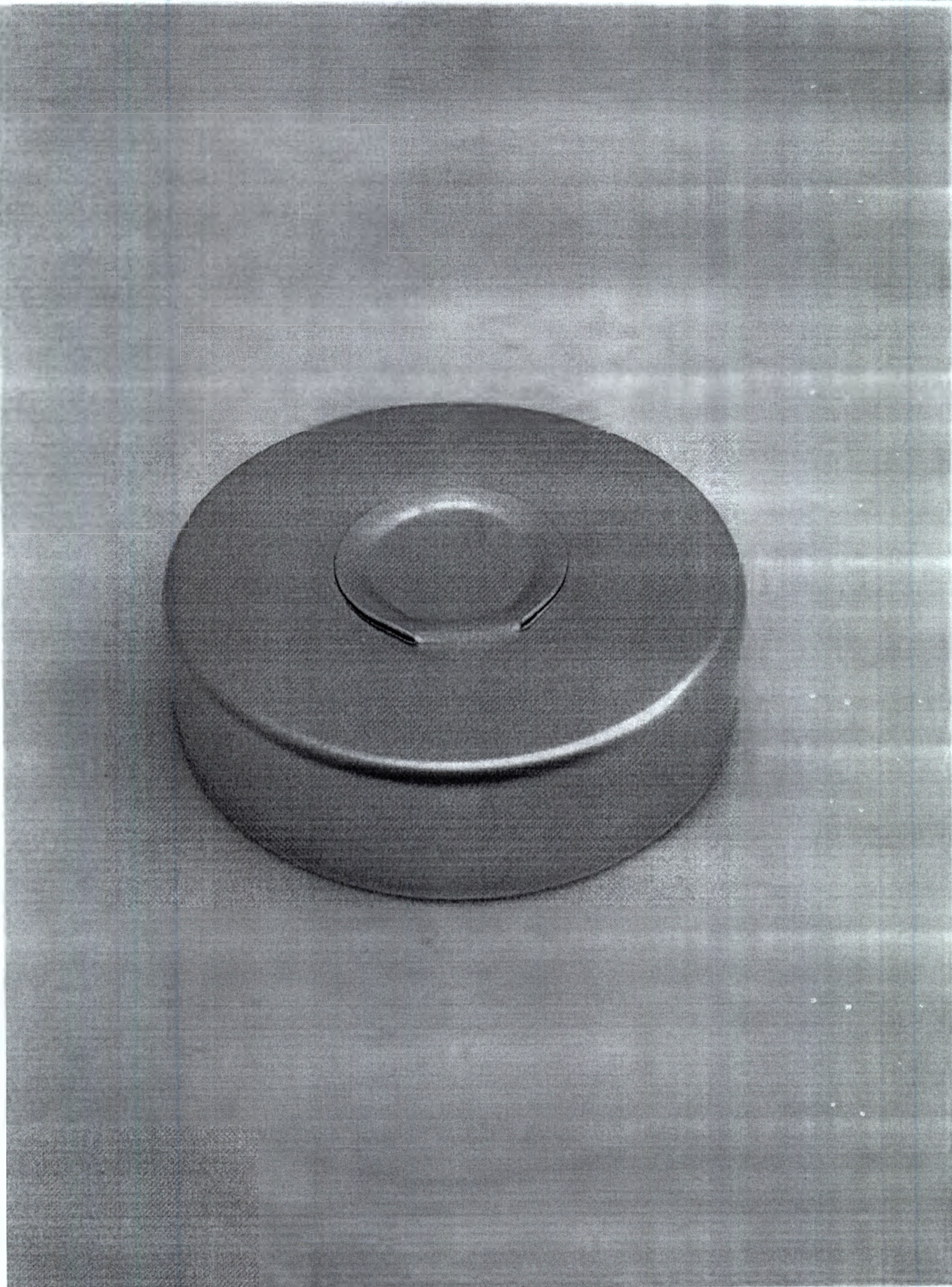
Общий вид колпачка алюминиевого гладкого, с надрезами (просечками) в дне колпачка, лепестком для отгиба. Исполнение 1.
