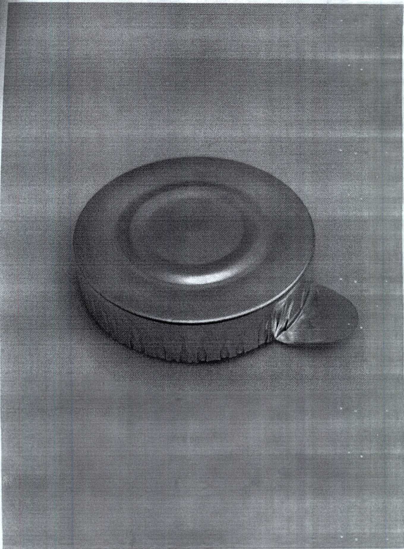
Общий вид колпачка алюминиевого гладкого с боковым отрываемым лепестком, с линиями ослабленного сечения.
