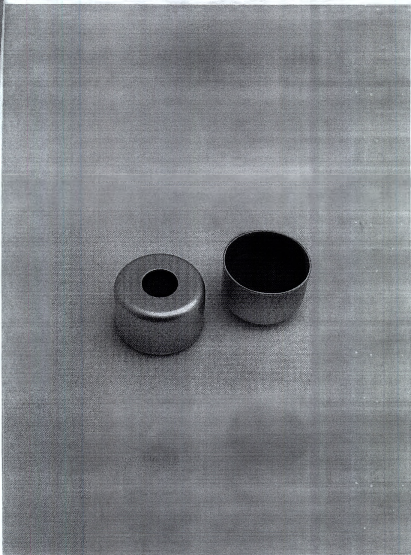
Общий вид колпачка алюминиевого с центральным отверстием в дне колпачка, с прокладкой (септой). Исполнение 2.
