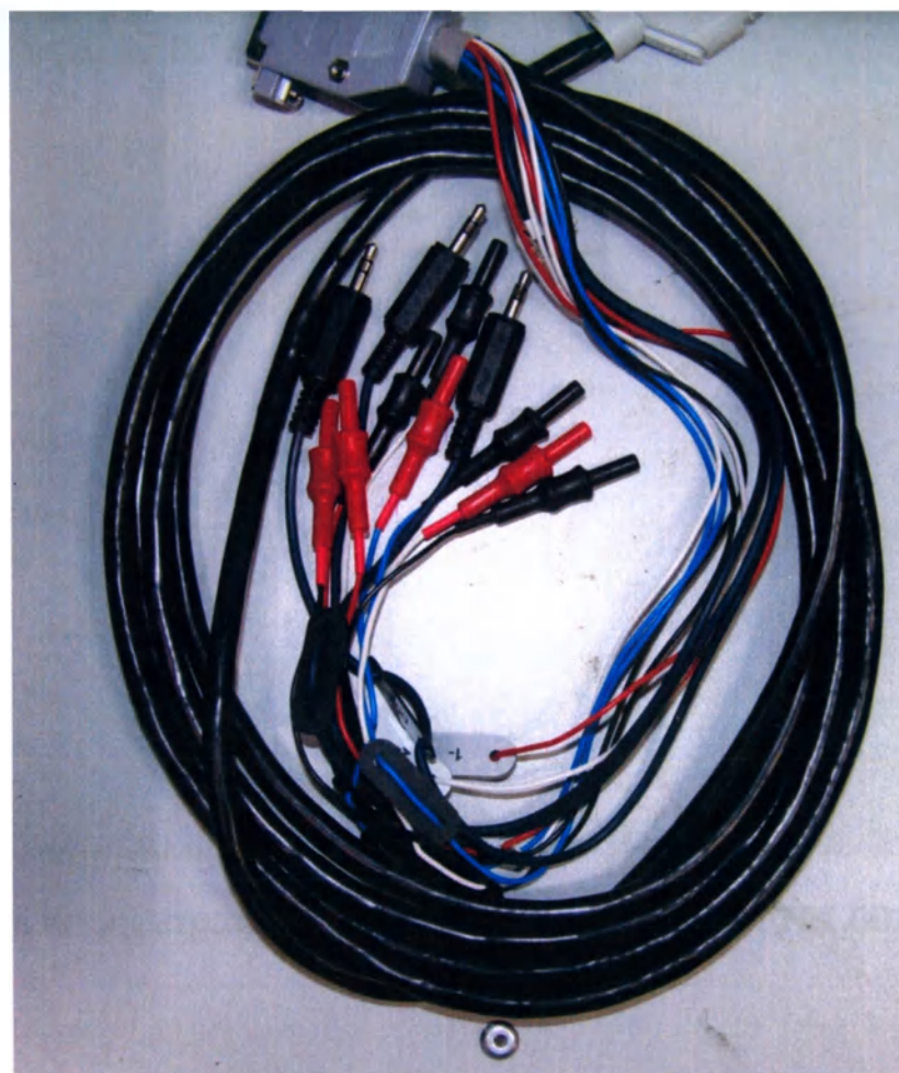
Кабель для подключения блока пациента «К-4П», NS055103.002
