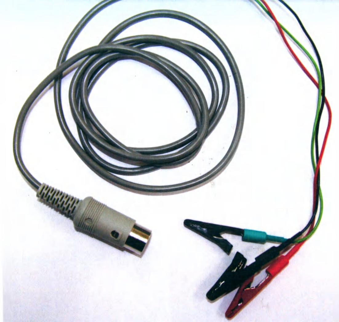
Кабель для подключения одноразовых электродов с коннектором «аллигатор», DIN240 NS990103.050
