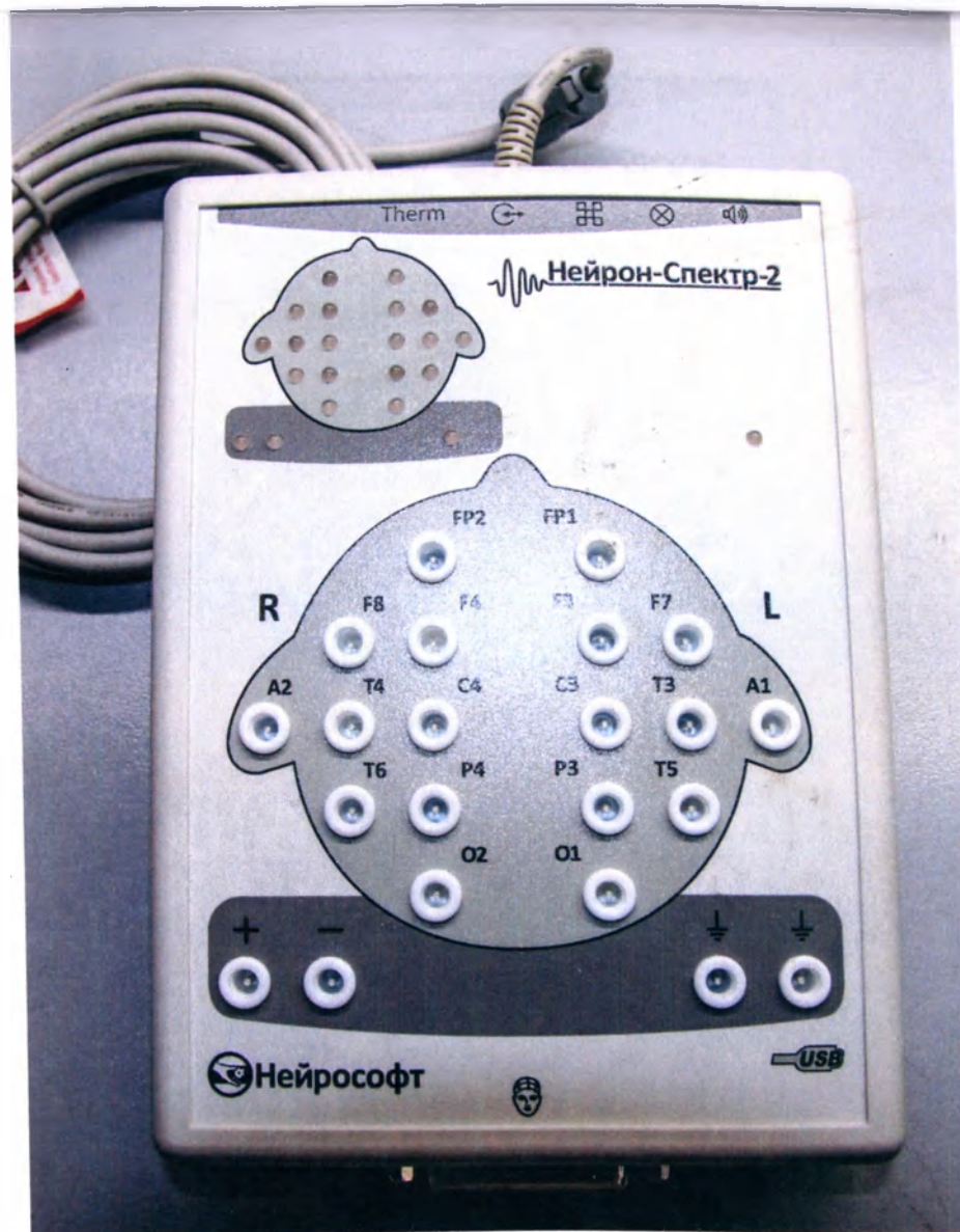
Электронный блок «Нейрон-Спектр-2» NS015201.042-010
