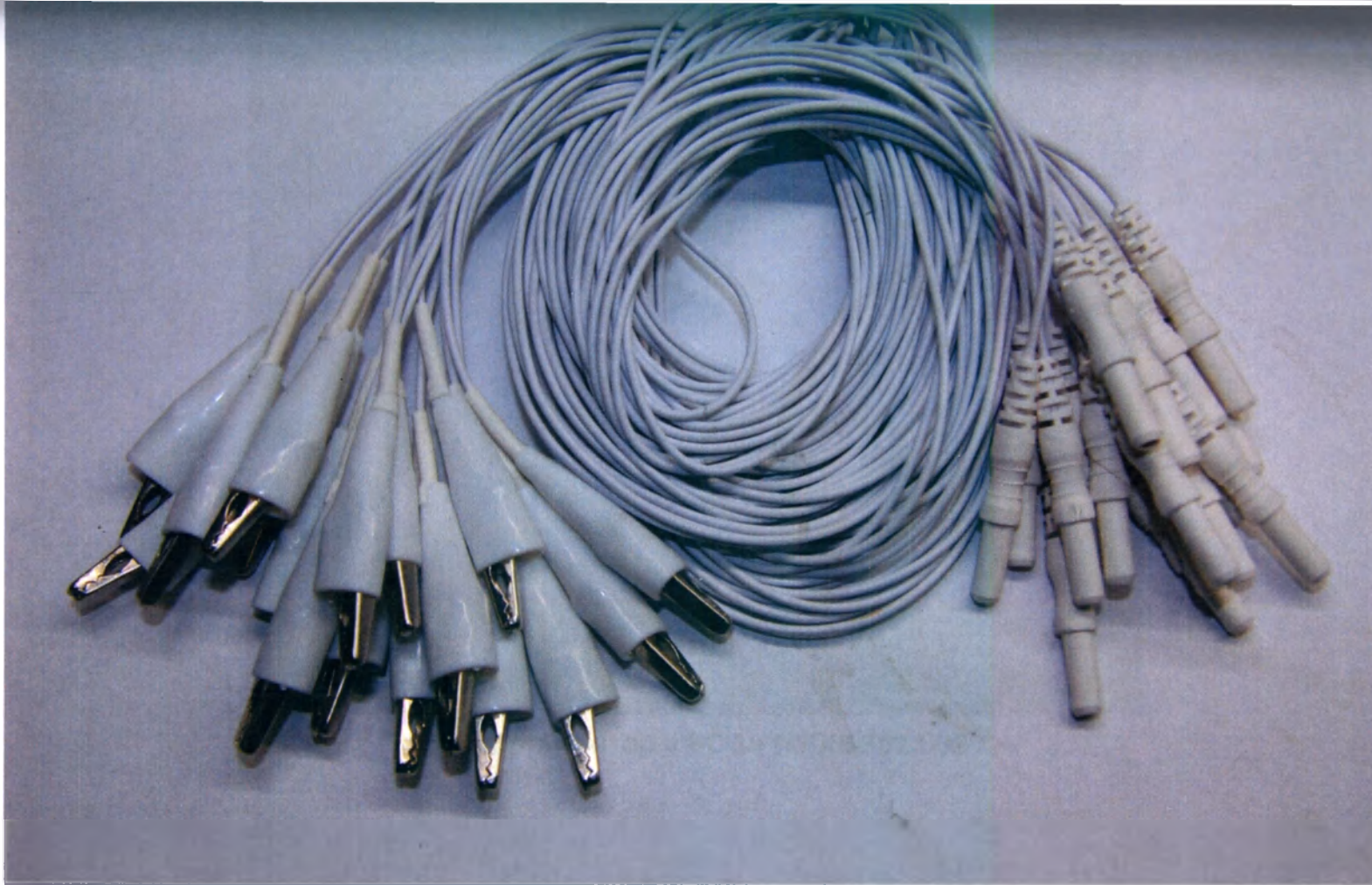
Кабель отведения для мостикового и ушного электрода ЭЭГ белый, 1 м NS990103.036-01.10
