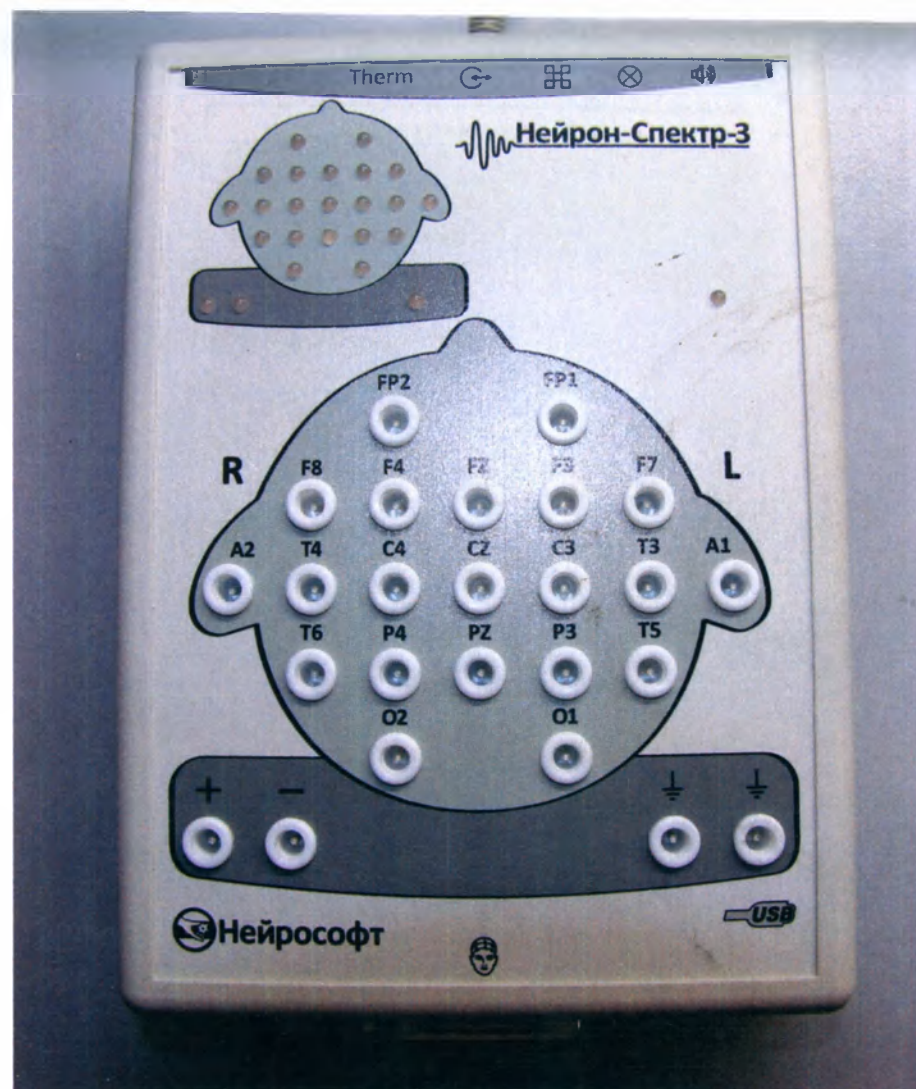
Электронный блок «Нейрон-Спектр-3» NS015201.043-010
