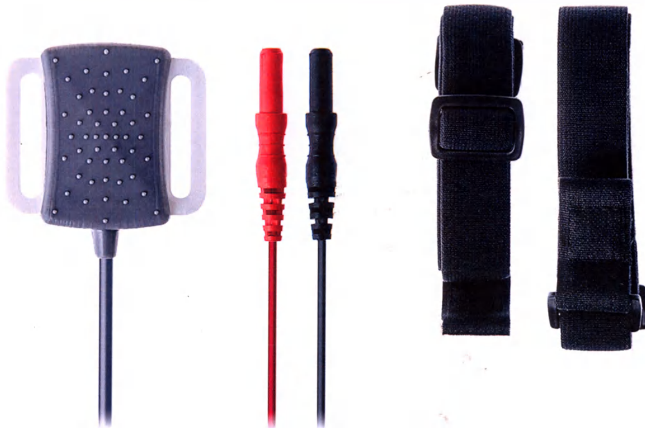
Датчик экскурсии грудной клетки и брюшной стенки «ДДП-4-22» с комплектом ремней NS990998.020
