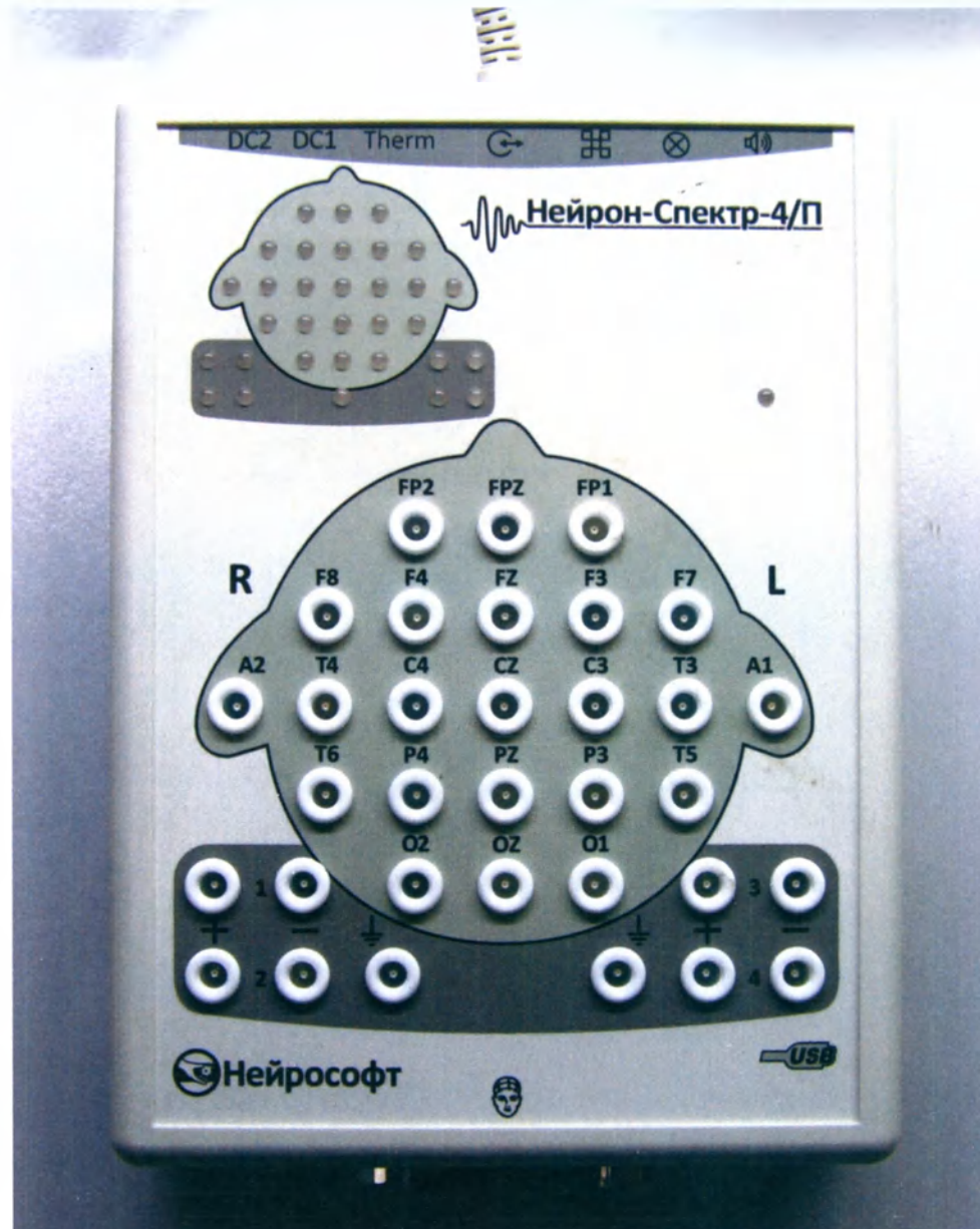
Электронный блок «Нейрон-Спектр-4/П» NS015201.045-010
