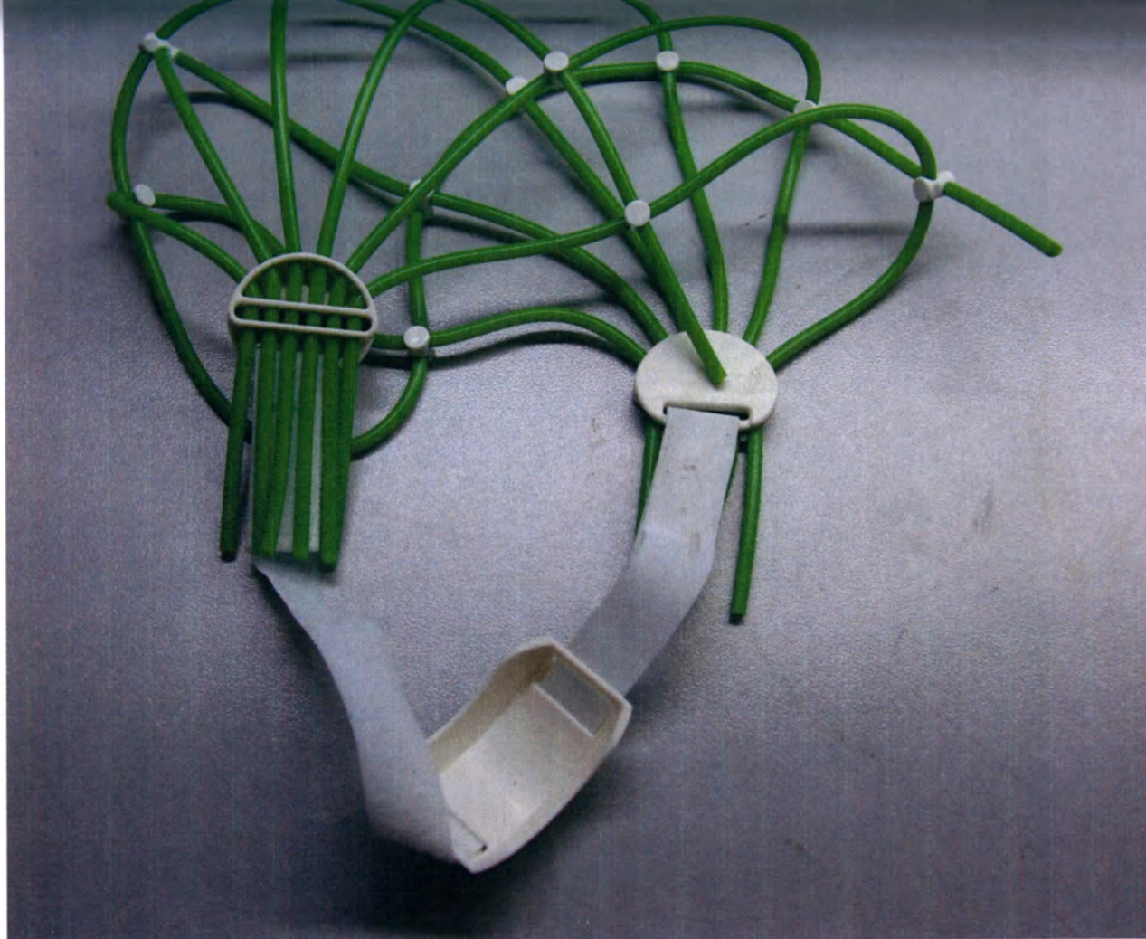
Шлем для крепления электродов ЭЭГ (48-54) NS023211.007-01
