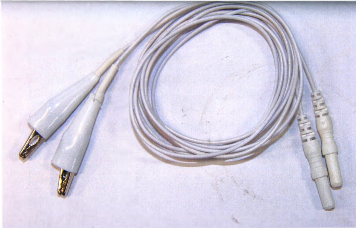
Кабель отведения для мостикового или ушного электрода ЭЭГ NS990103.036-01.10
