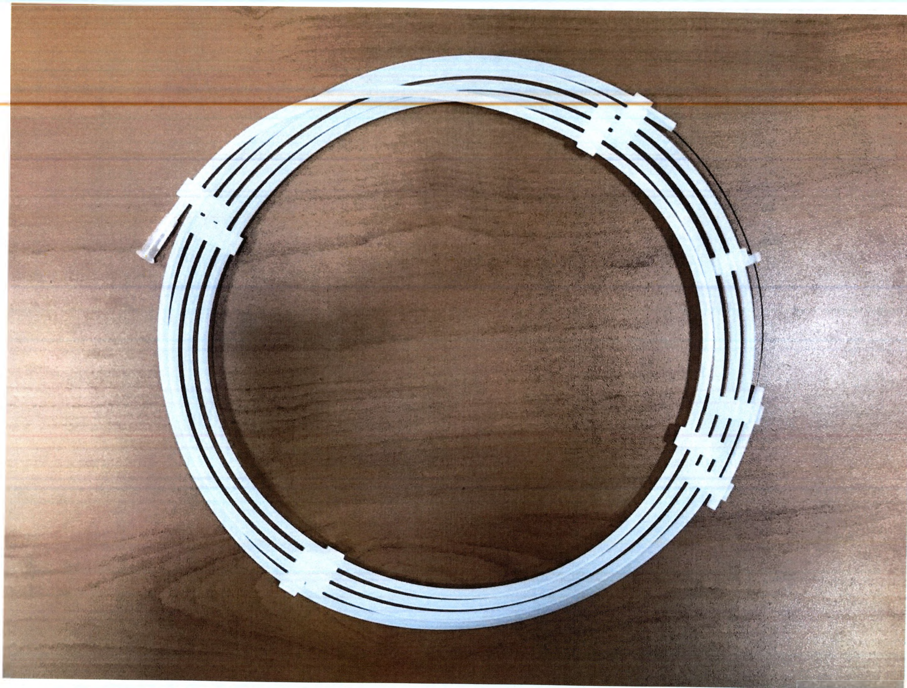
Защитная трубка для проводников длиной 300 см в сборке
