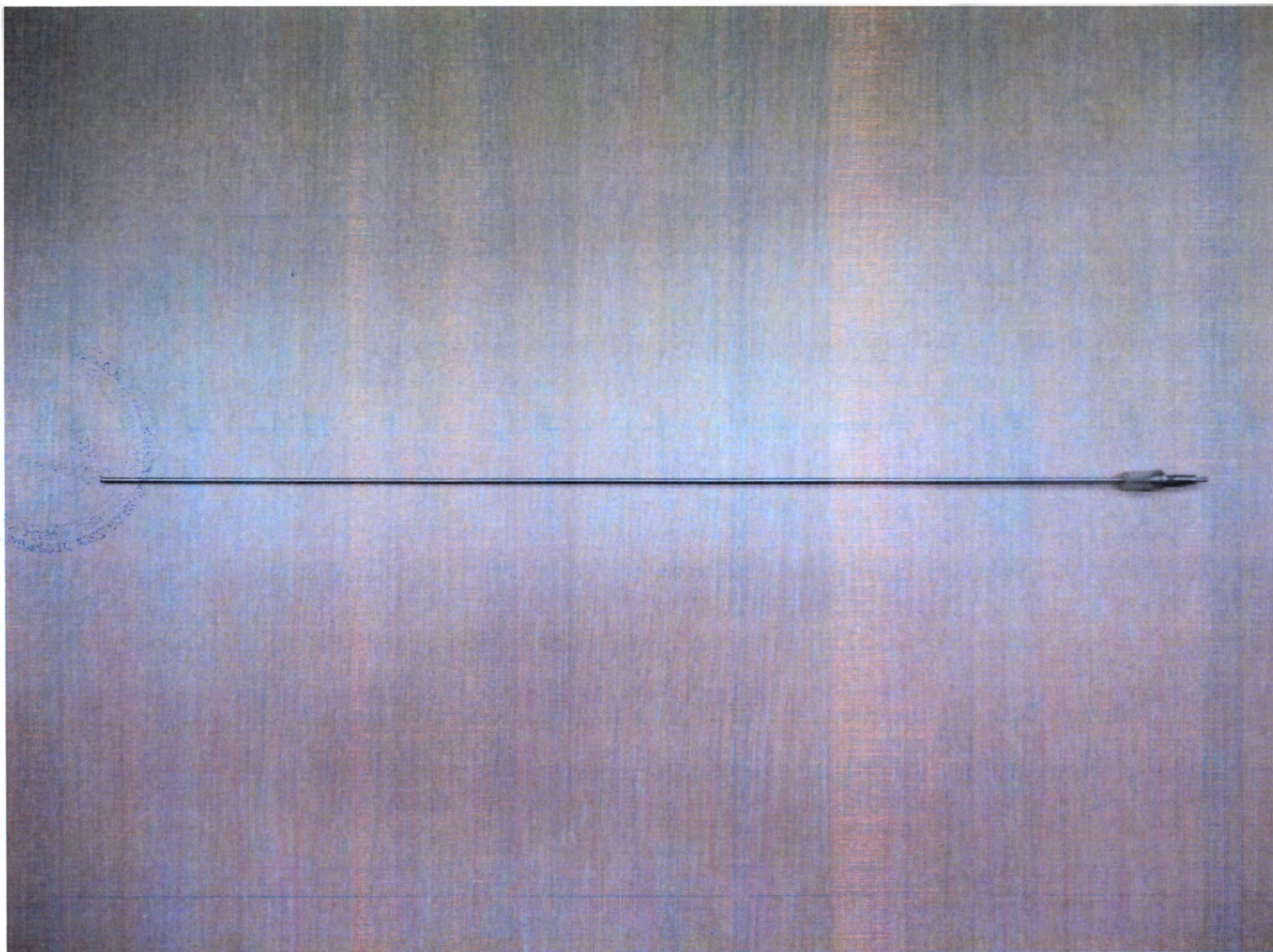
Зонд сплошной Ø 2,0 мм, длина 395 мм, рабочая длина 375 мм
