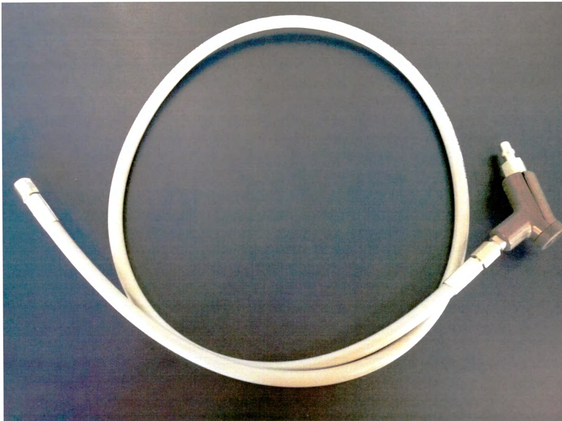
Шланг низкого давления, для системы централизованной подачи CO 2 , длина 150 см
