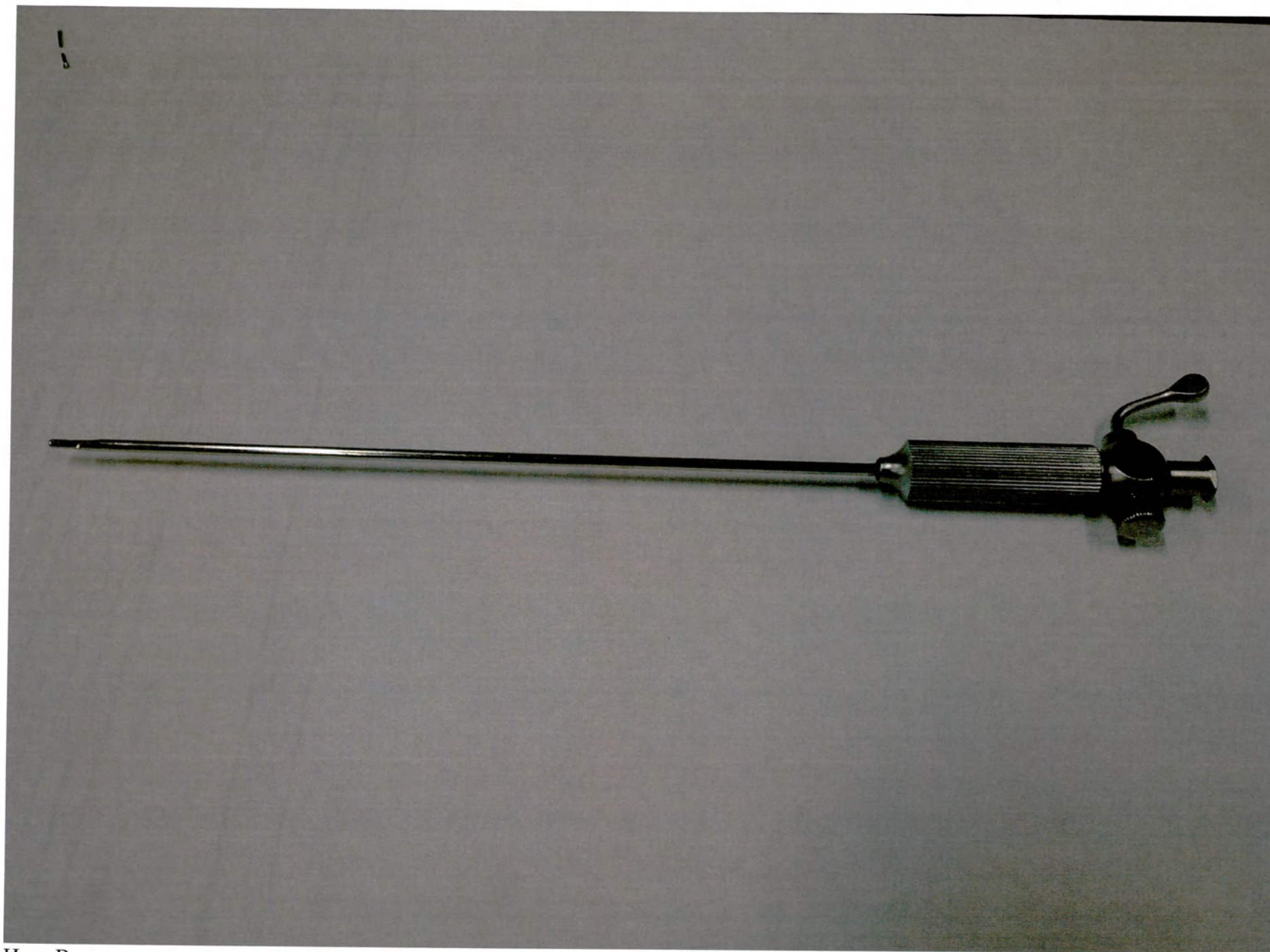
Игла Редена для пневмоперитонеума с тупоконечной внутренней канюлей на пружине, замок LUER, длина 12 см
