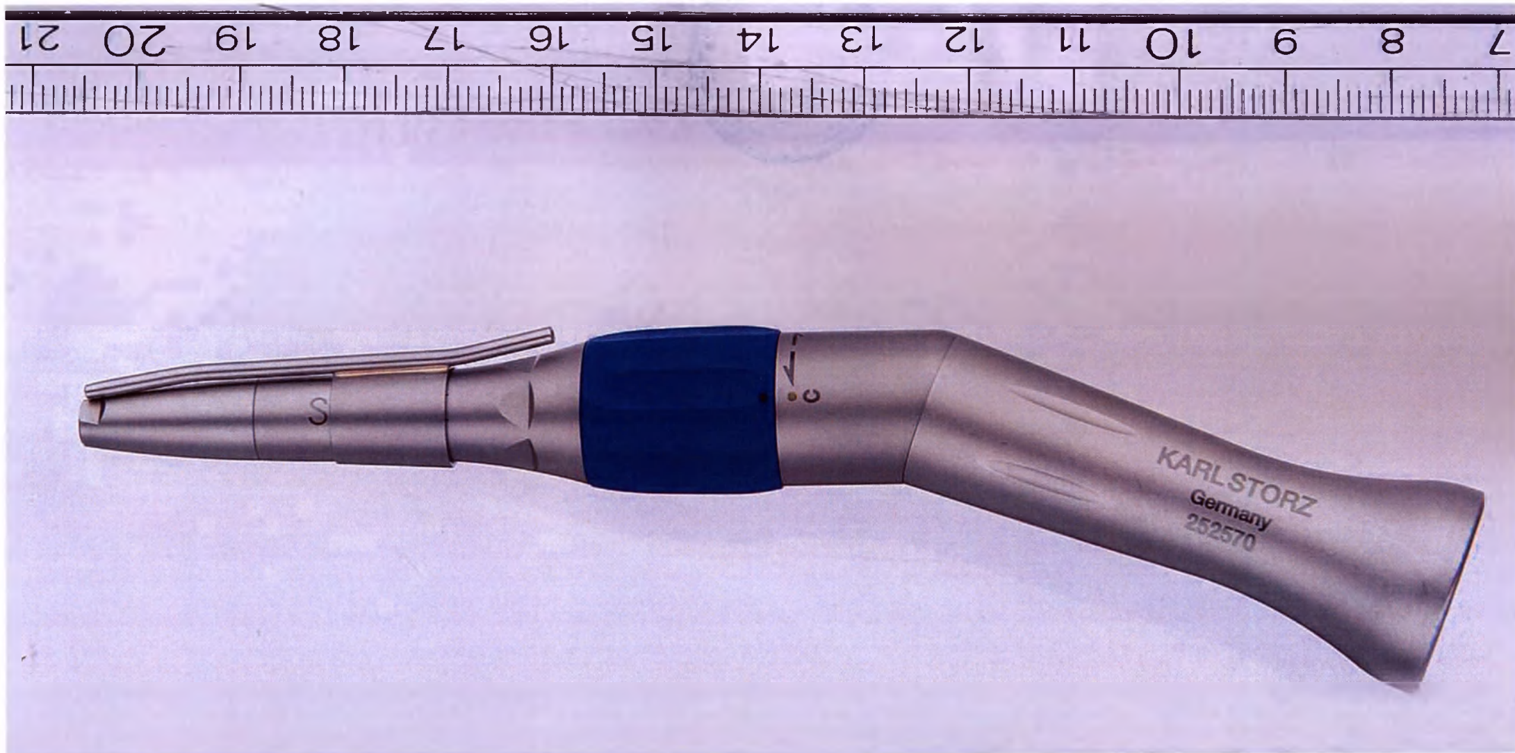
Хирургический наконечник INTRA, угловой, 12,5 см
