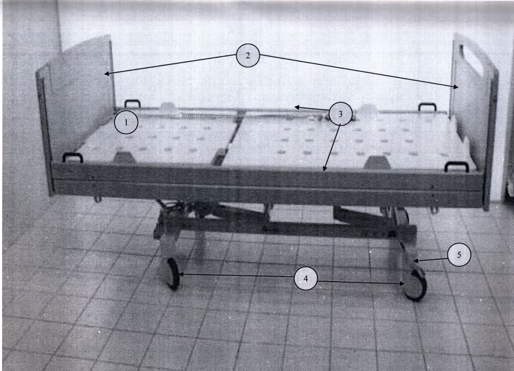
Кровать Salli H с регулируемой спинной секцией (1), установленными деревянными торцами (2) и боковыми ограждениями с механизмом защелкивания (3), колеса с центральной блокировкой (4) (5 – педаль тормоза на колесах с центральной блокировкой)
