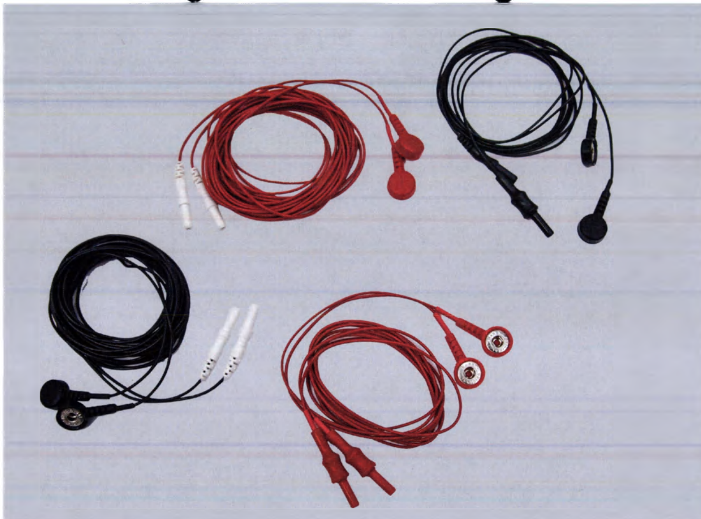
Кабель для подключения одноразовых электродов с коннектором «кнопка», разъем «touch-proff»: красный, 1.5 м (NS990103.037-03.15); черный, 1.5 м (NS990103.037-04.15); красный, 1 м (NS990103.037-03.10); черный, 1 м(NS990103.037-04.10).
