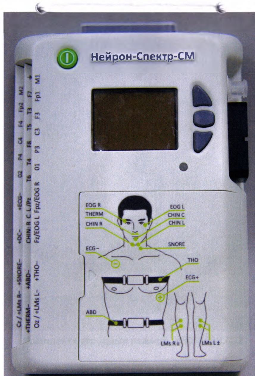
Блок регистрации «Нейрон-Спектр-СМ», NS053201.004
