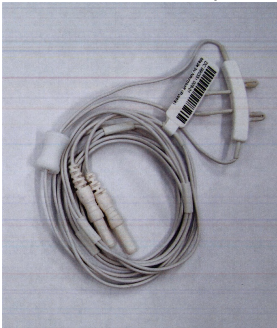
Датчик дыхания ДДТ-8/В-10 (детский) NS990351.009-01
