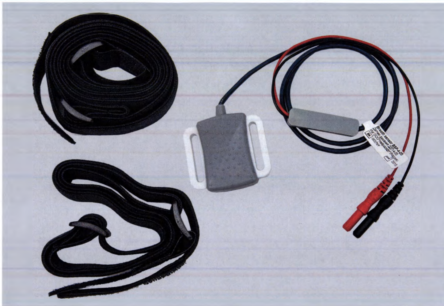
Датчик экскурсии грудной клетки и брюшной полости NS990998.020-02 в составе: датчик дыхания пьезокерамический «ДДП-4-05» с комплектом ремней
