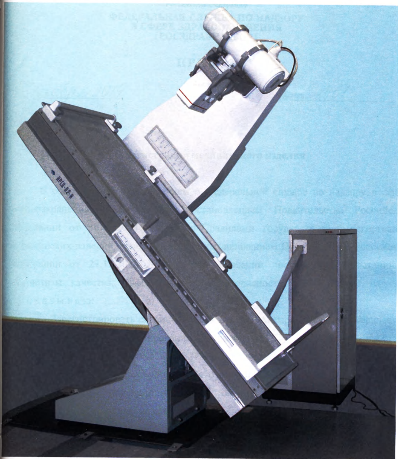
Аппарат рентгенографический линейного и углового сканирования цифровой APCQ-02-Н” ТУ 9442-002-07501706-2003
