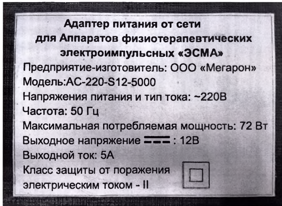
Рис. 18. Фотографическое изображение маркировки (этикетки) адаптера питания аппаратов «ЭСМА»
