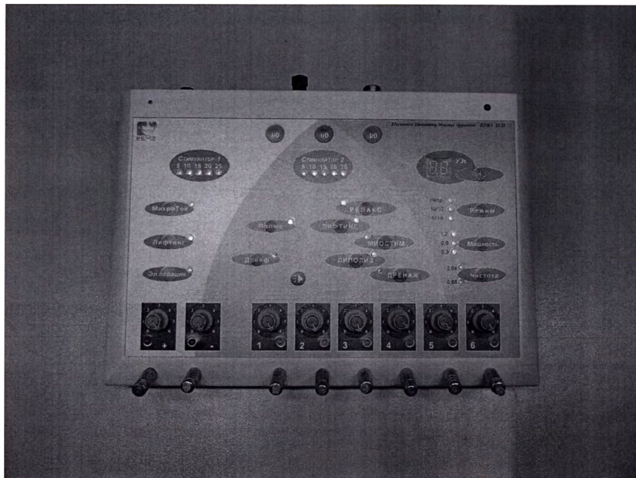
Рис.3 Аппарат «ЭСМА 12.50»
