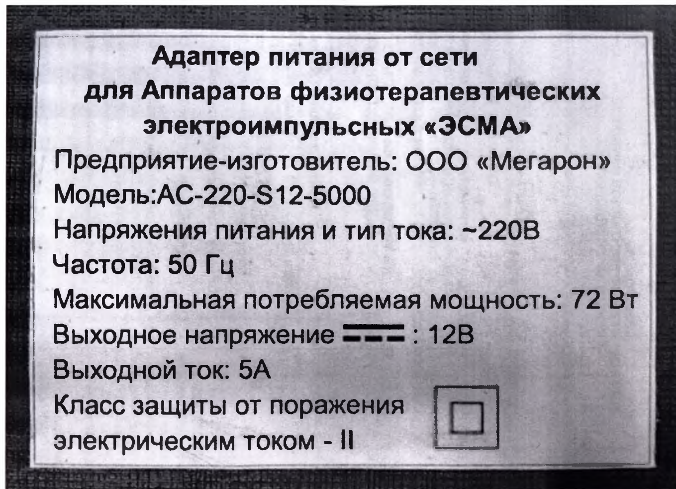
Рис. 12 Фотографическое изображение маркировки (этикетки) адаптера питания аппаратов «ЭСМА»:
