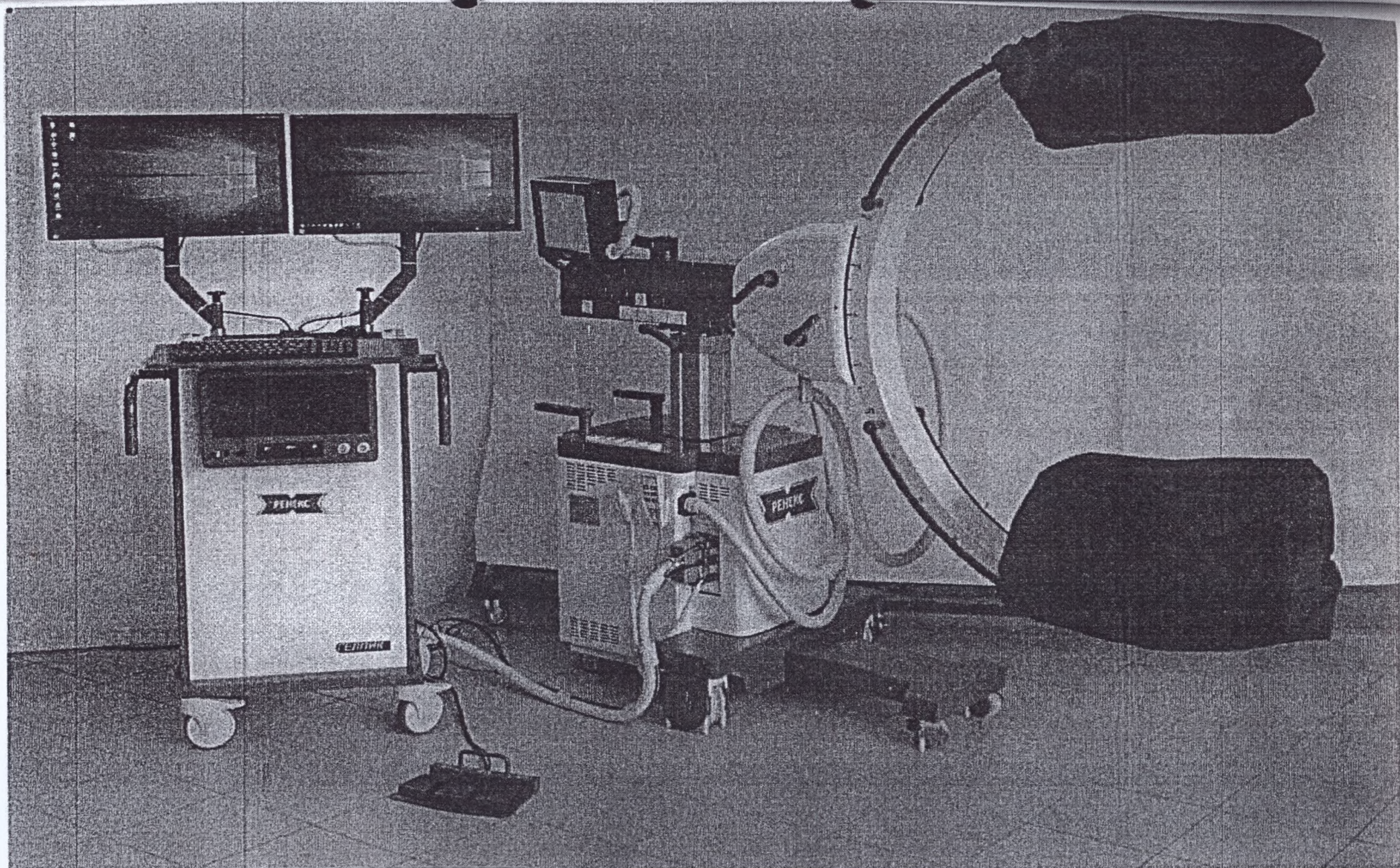
Общий вид с принадлежностями «Передвижной (мобильный) цифровой рентгенохирургический аппарат на базе штатива типа С-дуга» по ЛЖКМ.941211.001 ТУ
