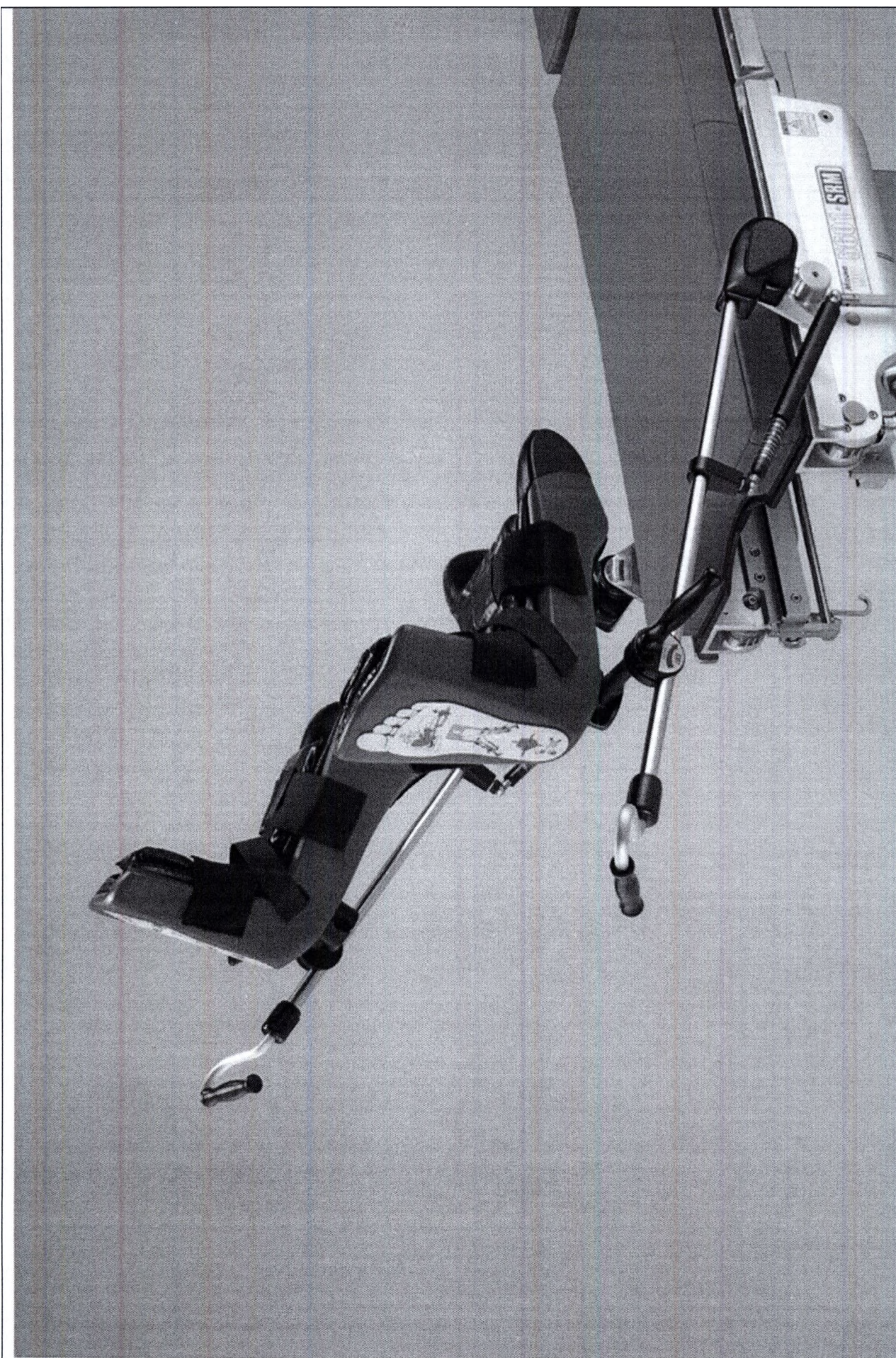
Опора для ног типа "поднятые стремяна", с креплением
