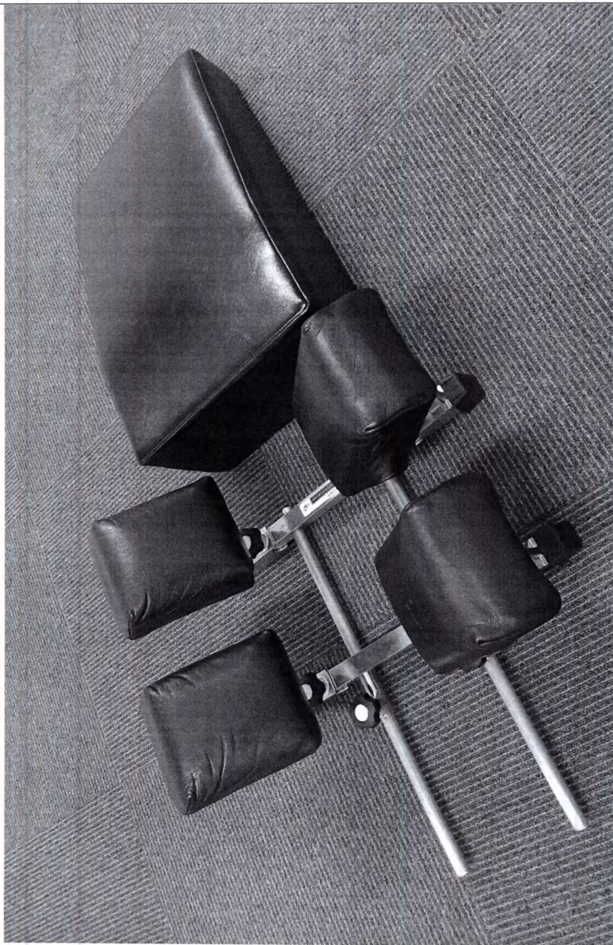
Четырехточечная рама для спинальных операций
