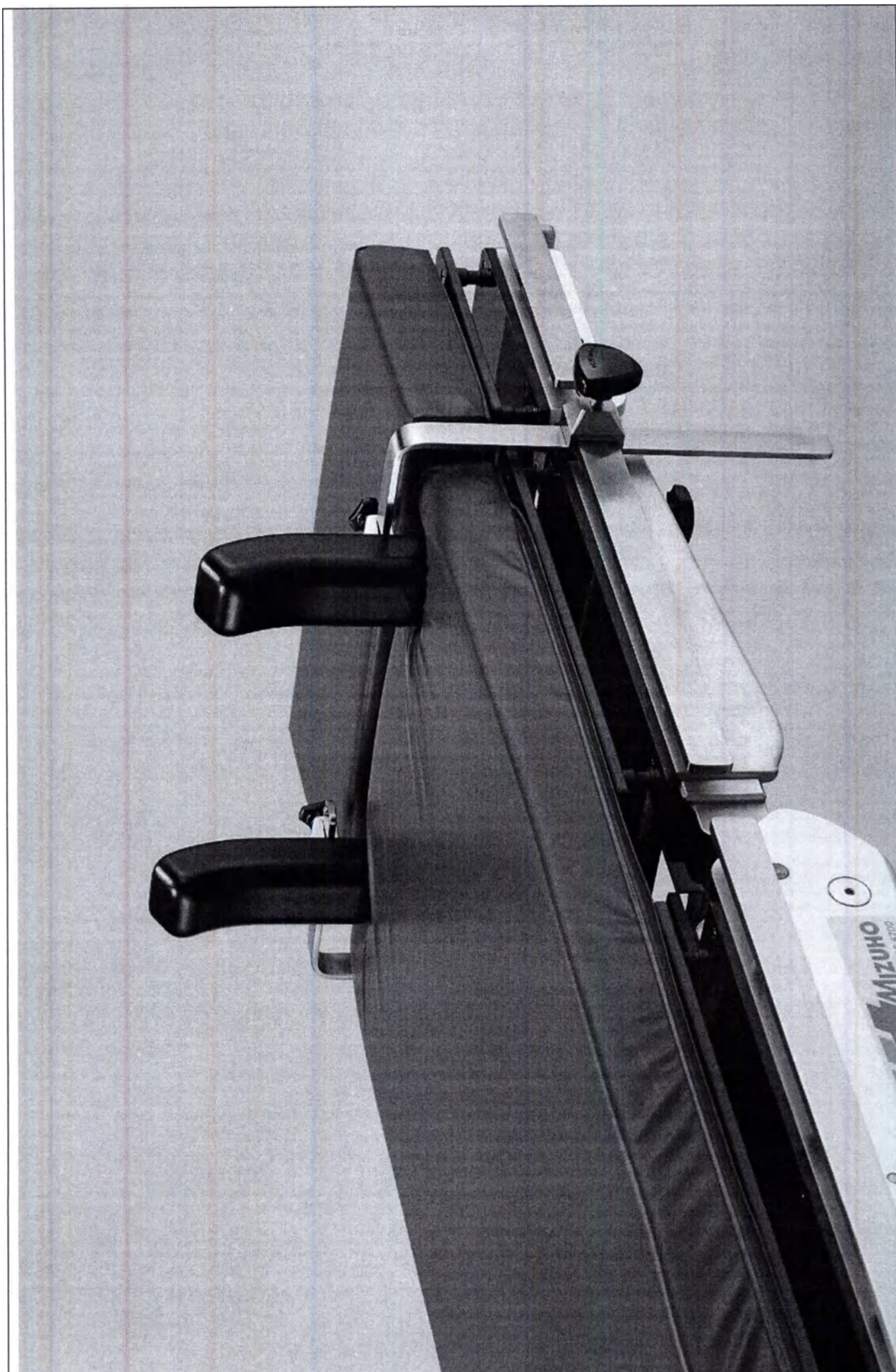
Плечевой упор, с креплением
