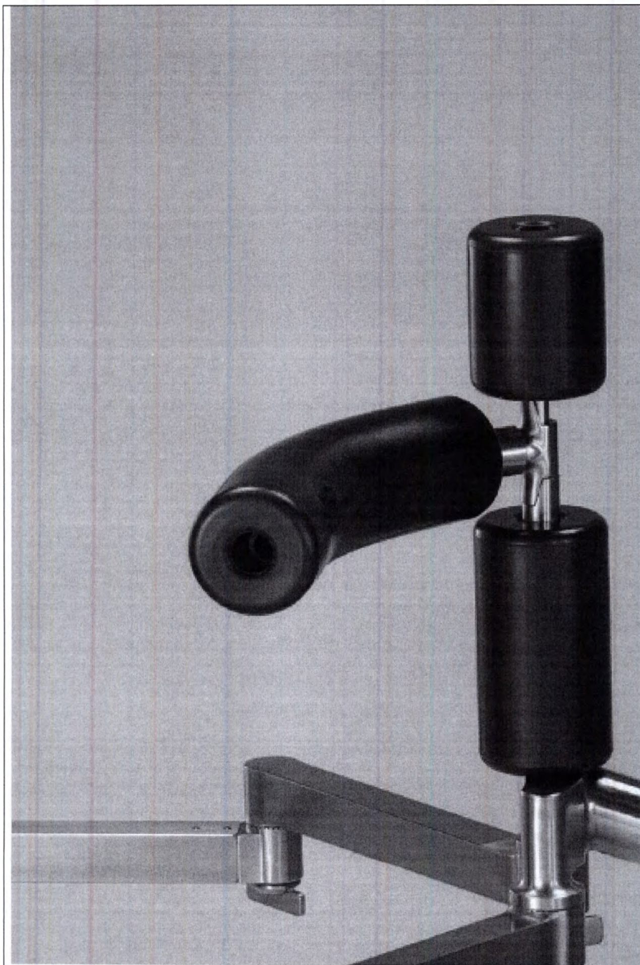
Внутренняя опора бедра для тракции в боковой позиции
