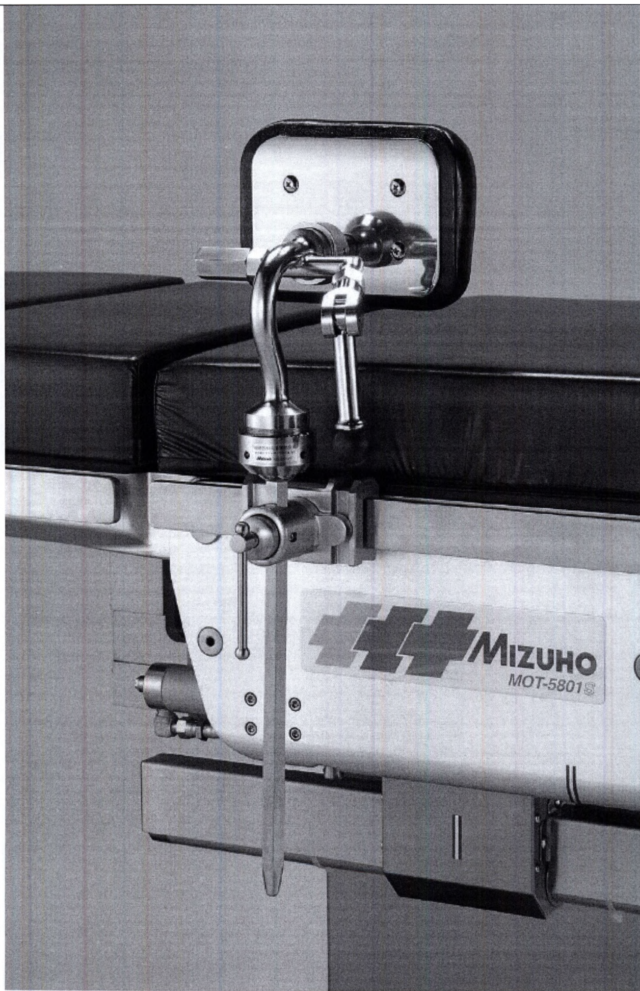
Регулируемая поддержка туловища, с креплением
