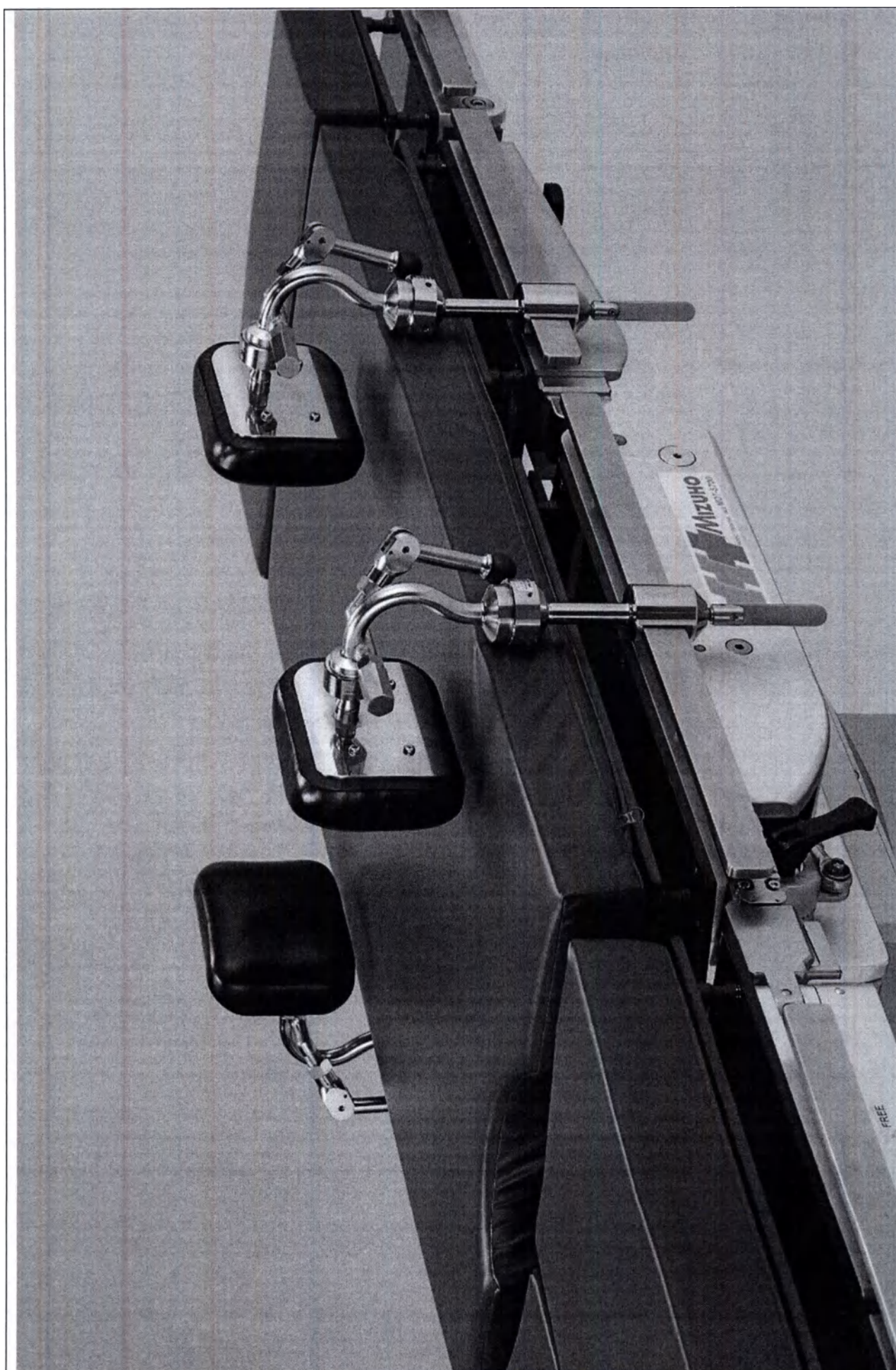
Легко регулируемая поддержка туловища, с креплением
