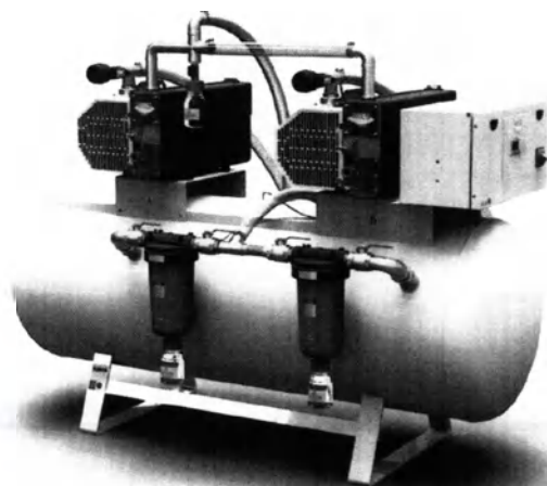
Установка медицинская вакуумная Вариант исполнения: Hospivac 2 E65
