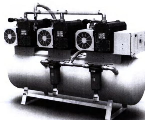
Установка медицинская вакуумная Вариант исполнения: Hospivac 3 E150
