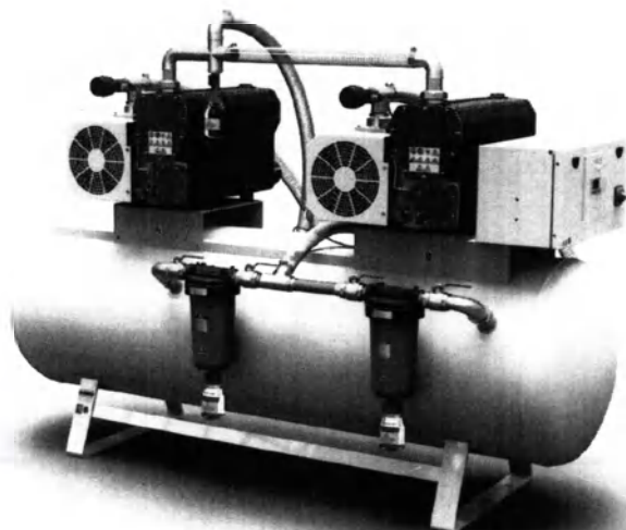
Установка медицинская вакуумная Вариант исполнения: Hospivac 2 E150
