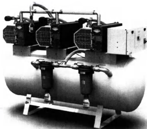
Установка медицинская вакуумная Вариант исполнения: Hospivac 3 E100
