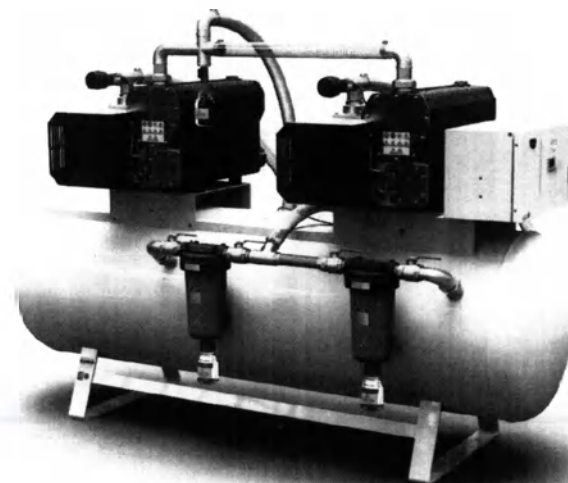
Установка медицинская вакуумная Вариант исполнения: Hospivac 2 E200
