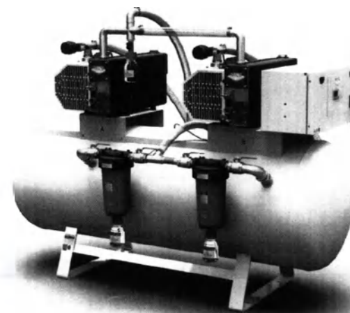
Установка медицинская вакуумная Вариант исполнения: Hospivac 2 E100
