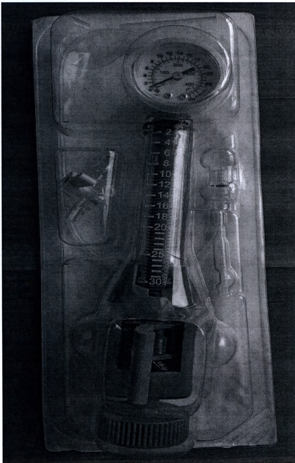
Общий вид Раздувающего устройства для ЧТКА Flute-S в упаковке
