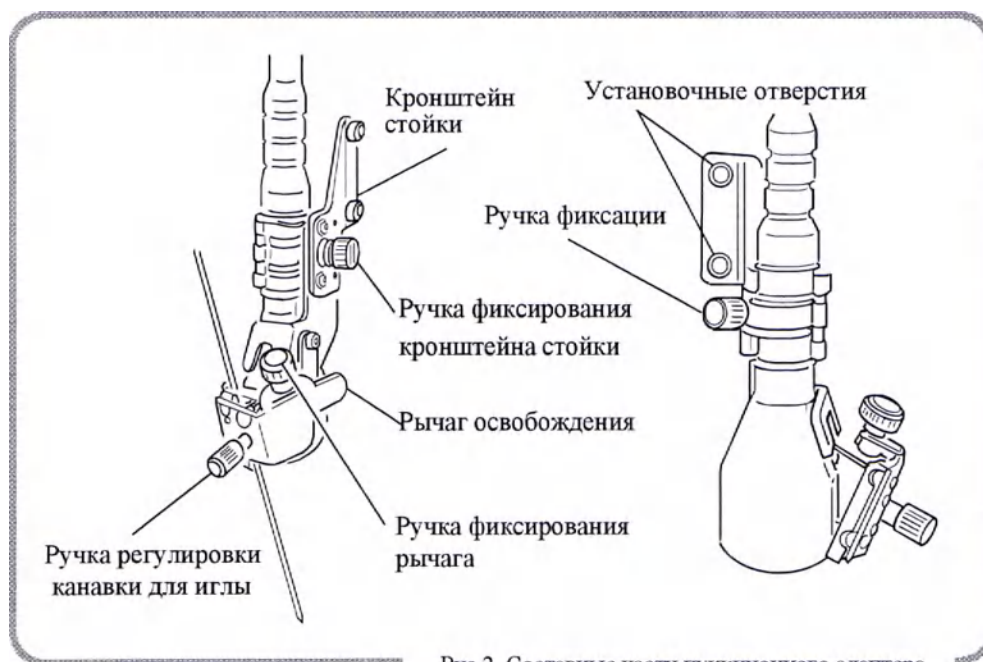
Рис.2. Составные части пункционного адаптера
