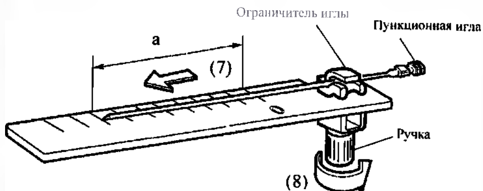
Рис. 14 Фиксирование ограничителя иглы
