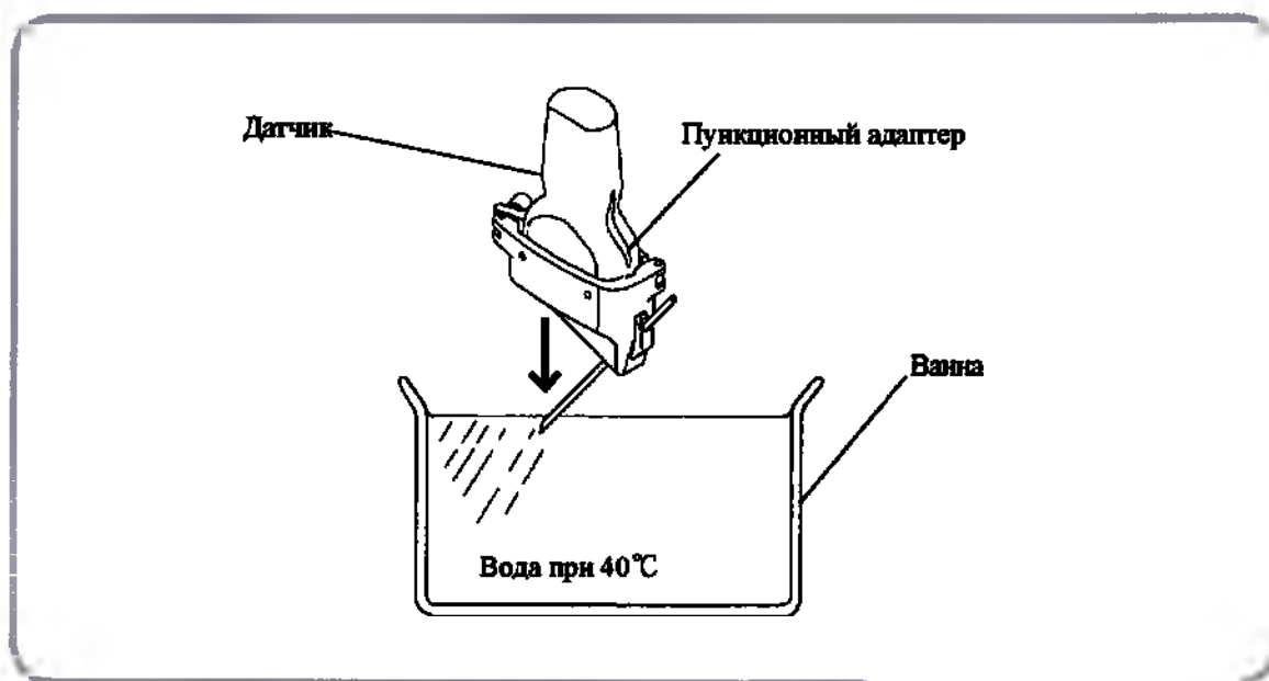
Рис. 3 Проверка эхо-сигнала от иглы 1
