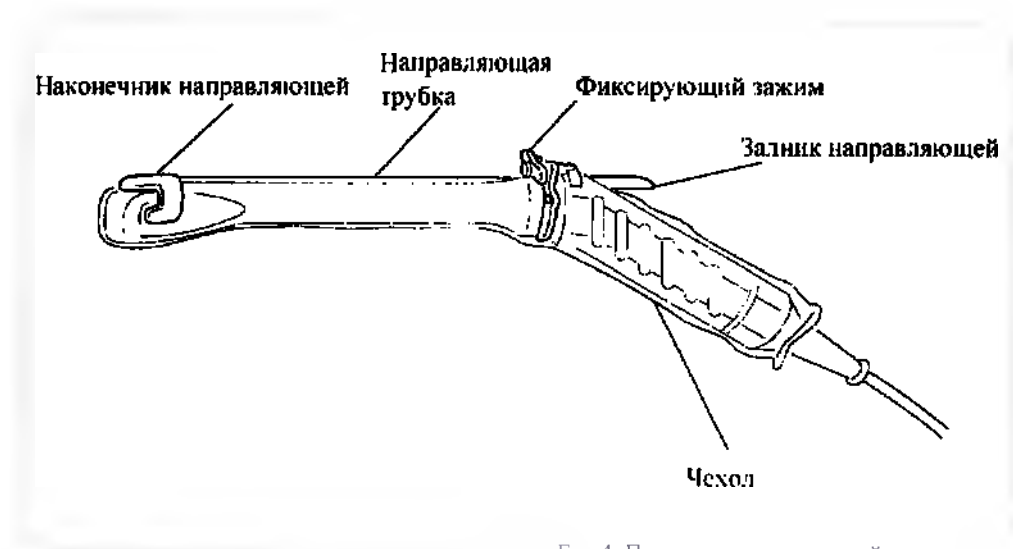
Fig 4. Проверка направляющей пункции
