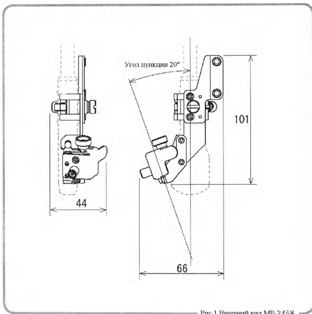
Рис.1 Внешний вид MP-2458
