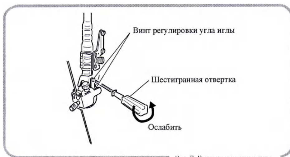
Рис. 7 Регулировка угла иглы
