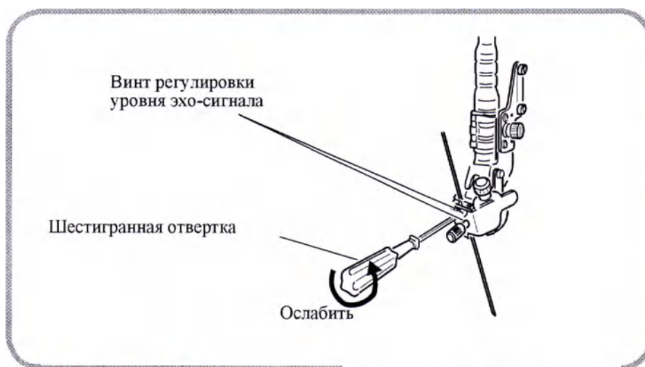
Рис. 8 Регулировка уровня эхо-сигнала от иглы.
