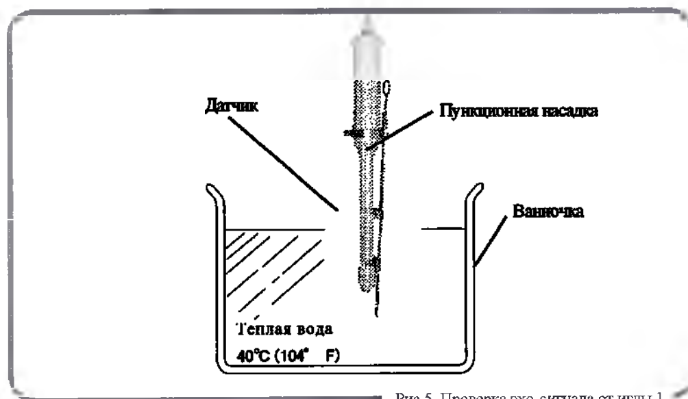
Рис.5. Проверка эхо-сигнала от иглы 1
