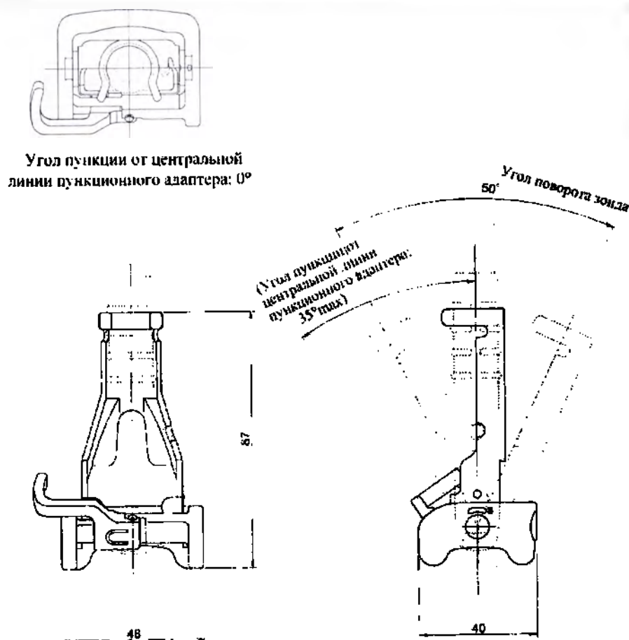
Рис.1 Внешний вид MP-2783
