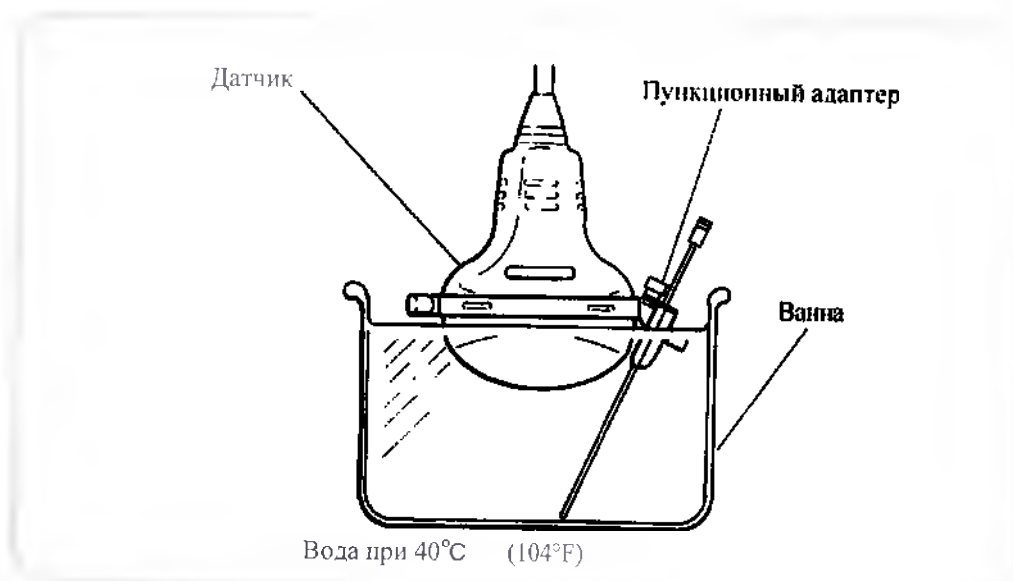
Рис. 5 Проверка эхо-сигнала от иглы 1
