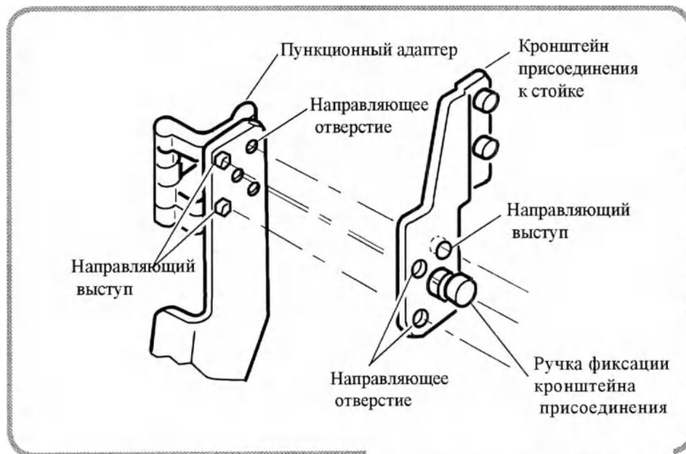
Рис.15 Фиксация кронштейна присоединения к стойке.
