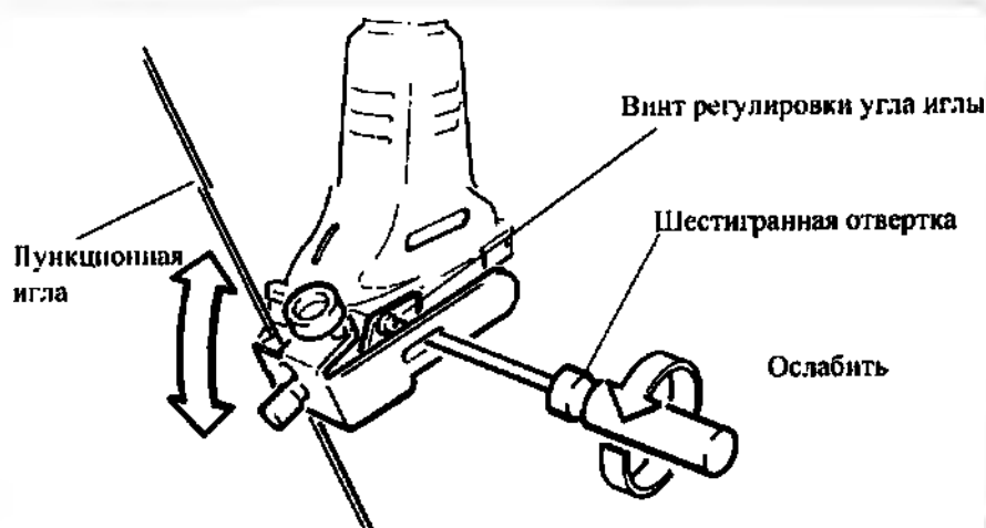
Рис. 7 Регулировка угла иглы
