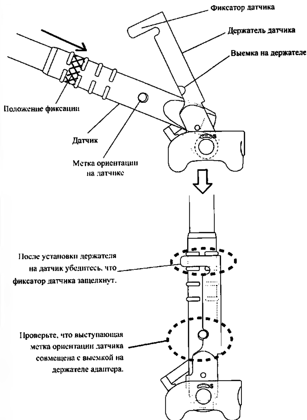
Рис.9. Сборка и крепление функционального адаптера
