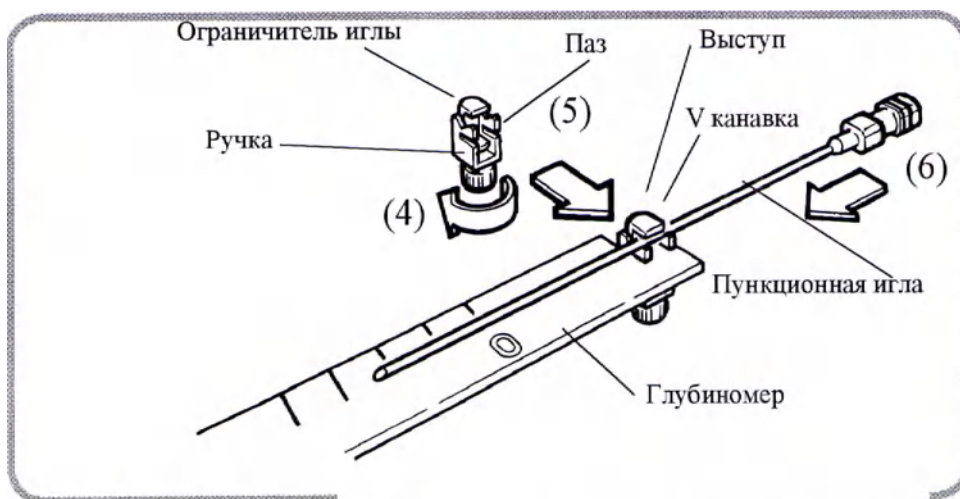
Рис. 12 Присоединение пункционной иглы к ограничителю иглы
