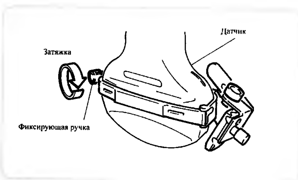
Рис.11 Присоединение и фиксация пункционного адаптера
