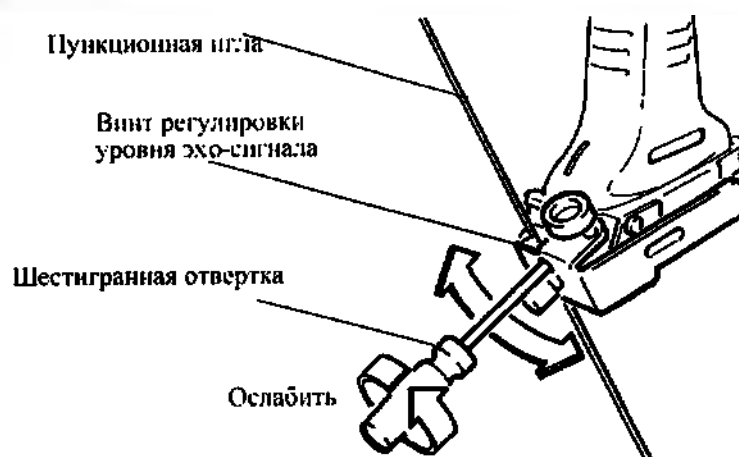
Рис. 8 Регулировка уровня эхо-сигнала от иглы.
