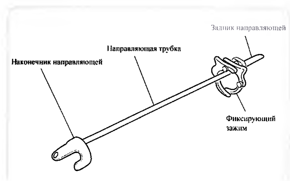
Рис. 2. Название составных частей пункционной направляющей
