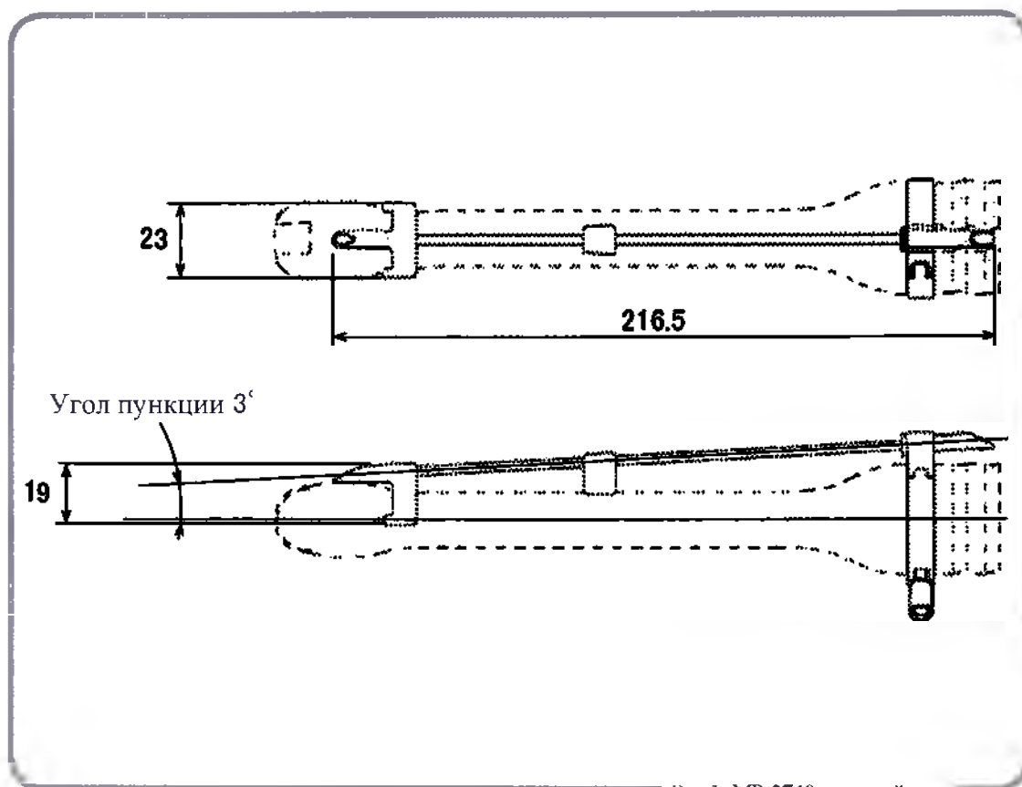
Рис.1. MP-2748 внешний вид
