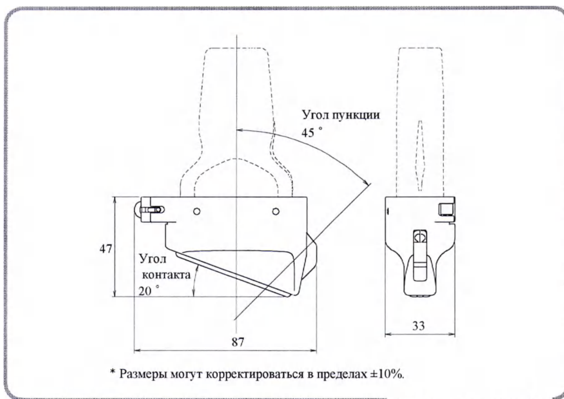
Рис.1 Внешний вид ECM-16
