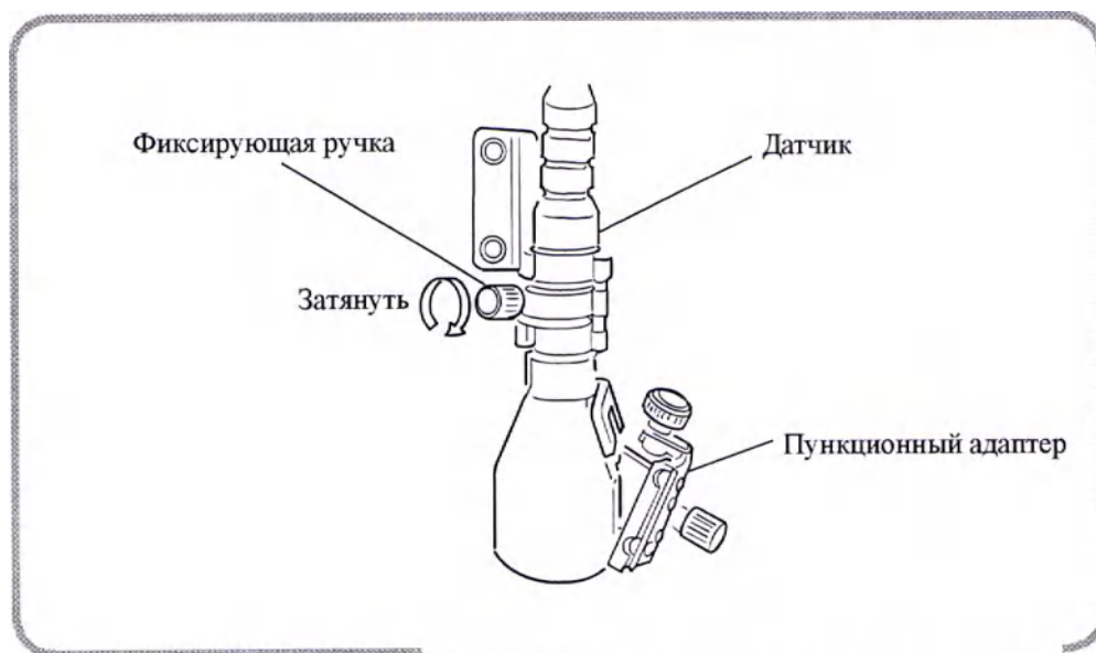
Рис.10 Присоединение и фиксация пункционного адаптера
