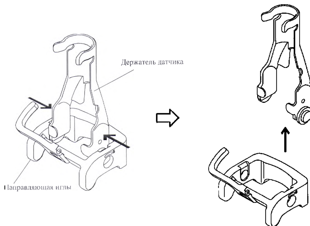
Рис.13. Разборка пункционного адаптера
