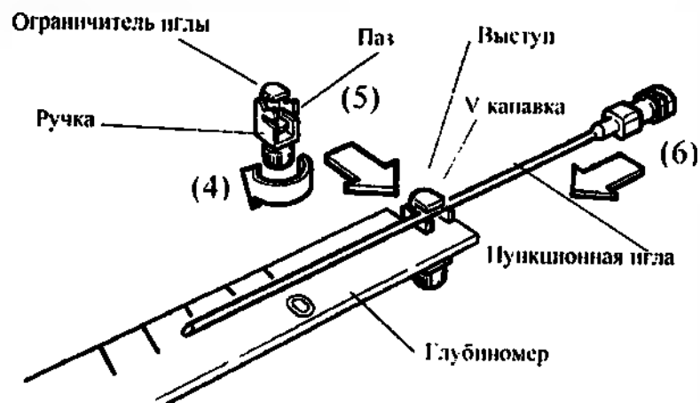
Рис. 13 Присоединение пункционной иглы к ограничителю иглы
