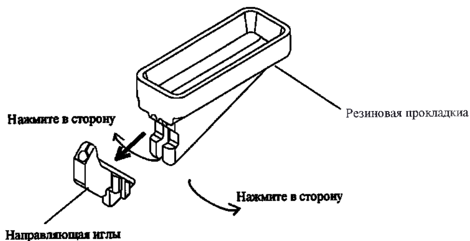
Рис.9. Удаление резиновой прокладки
