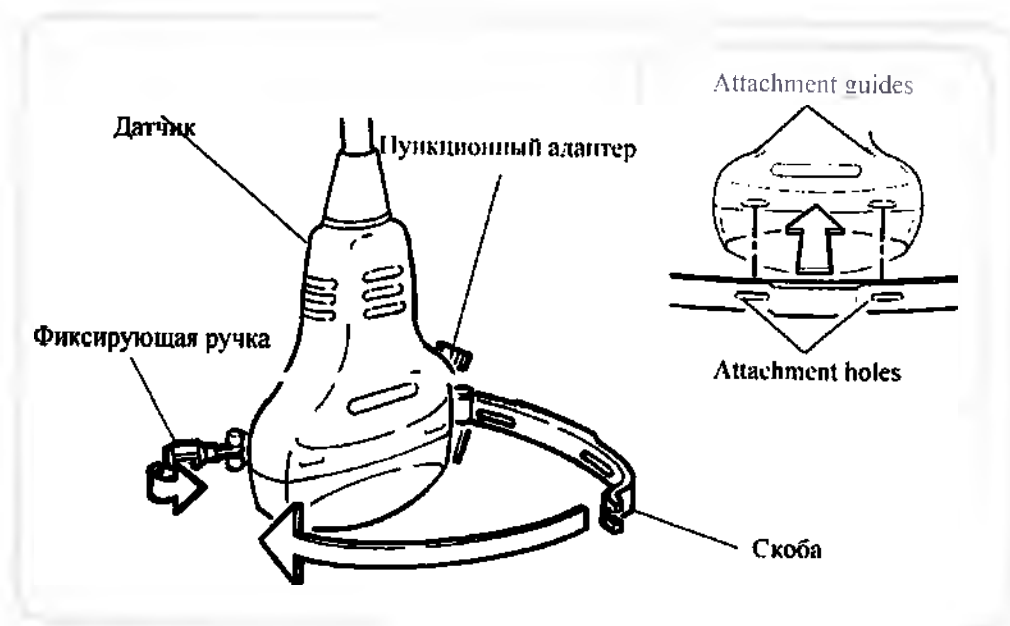
Рис.10 Присоединение и фиксация пункционного адаптера
