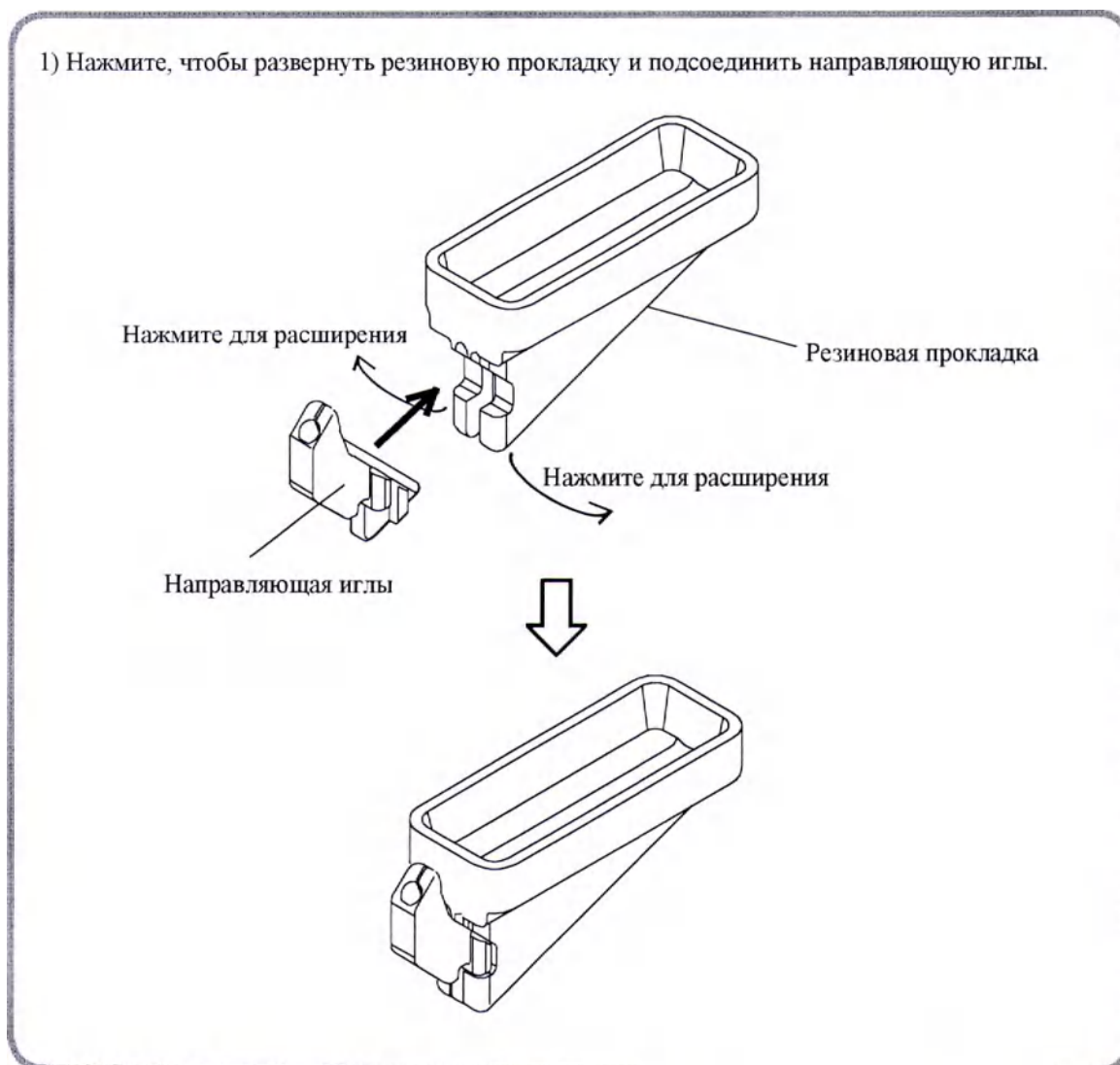
Рис. 5. Сборка пункционного адаптера 1
