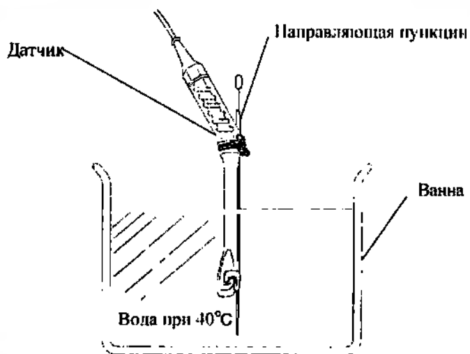
Рис. 5 Проверка эхо-сигнала от иглы
