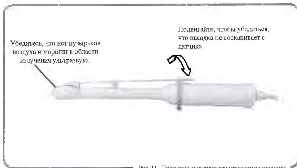
Рис.11. Проверка надежности крепления насадки
