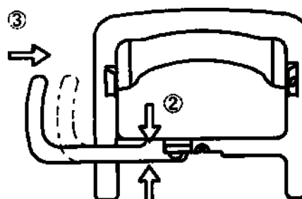
Рис.7. Сборка и крепление пункционного адаптера
