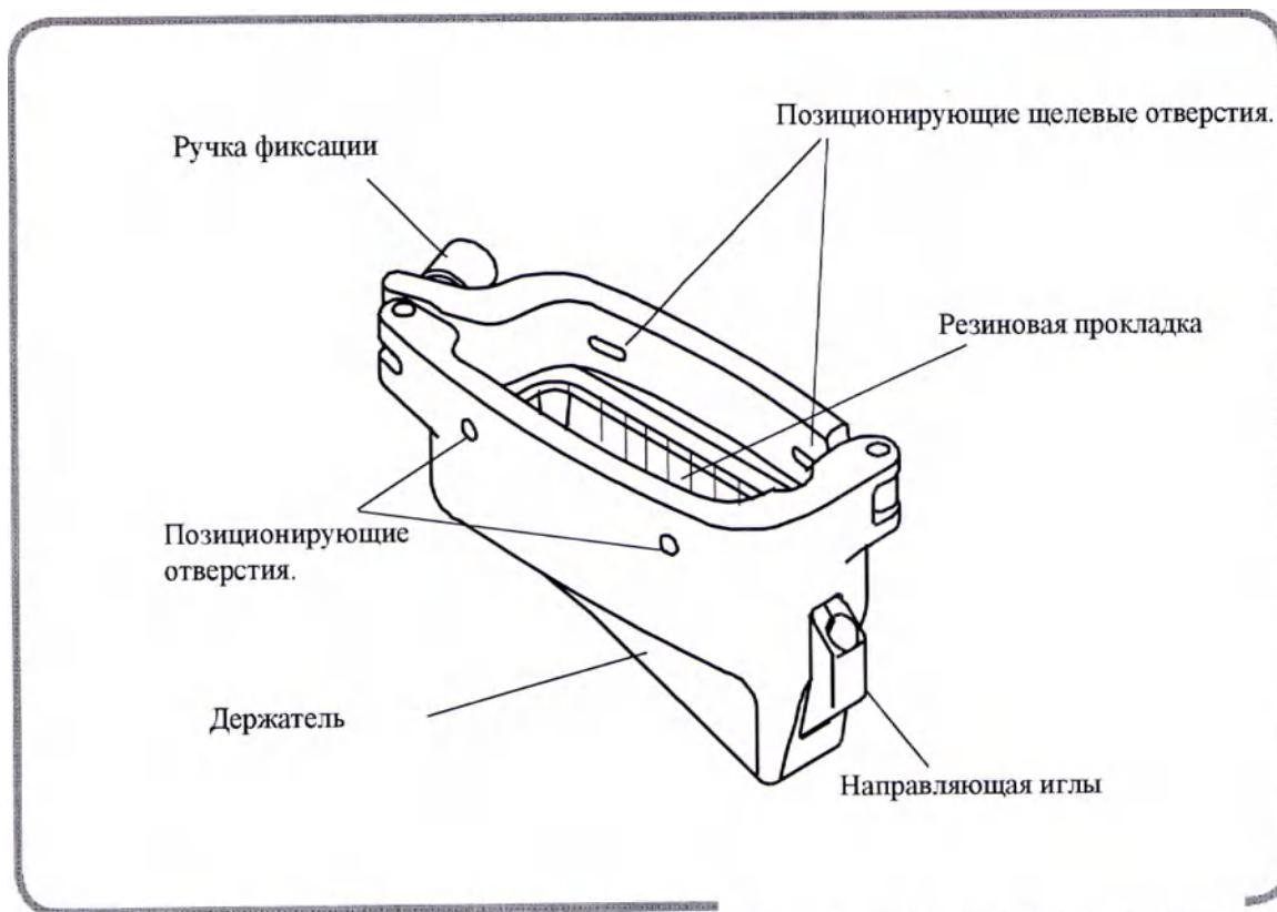
Рис.2. Составные части пункционного адаптера
