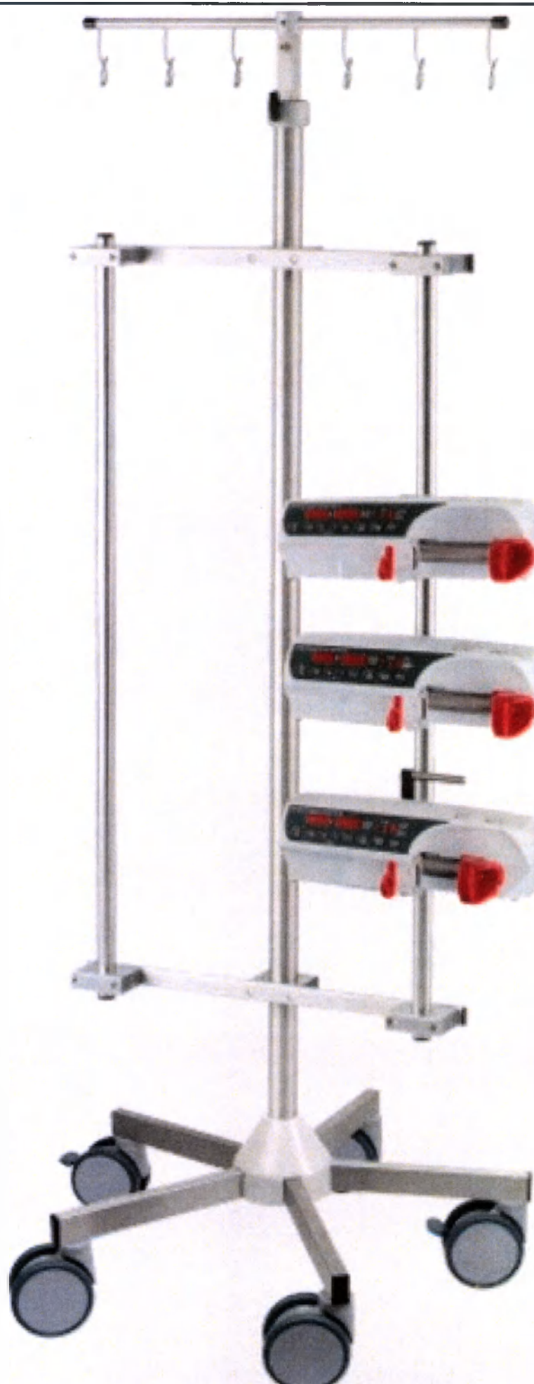
Рис 1.142. Стойка инфузионная provita передвижная «ISP-Unit»: I-PB2226
