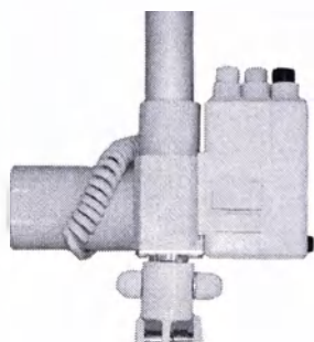
Рис.2 Исполнительный механизм Med-i-Drive 6/5-24 и блок управления Med-i-Drive 24/12М (Китай)
