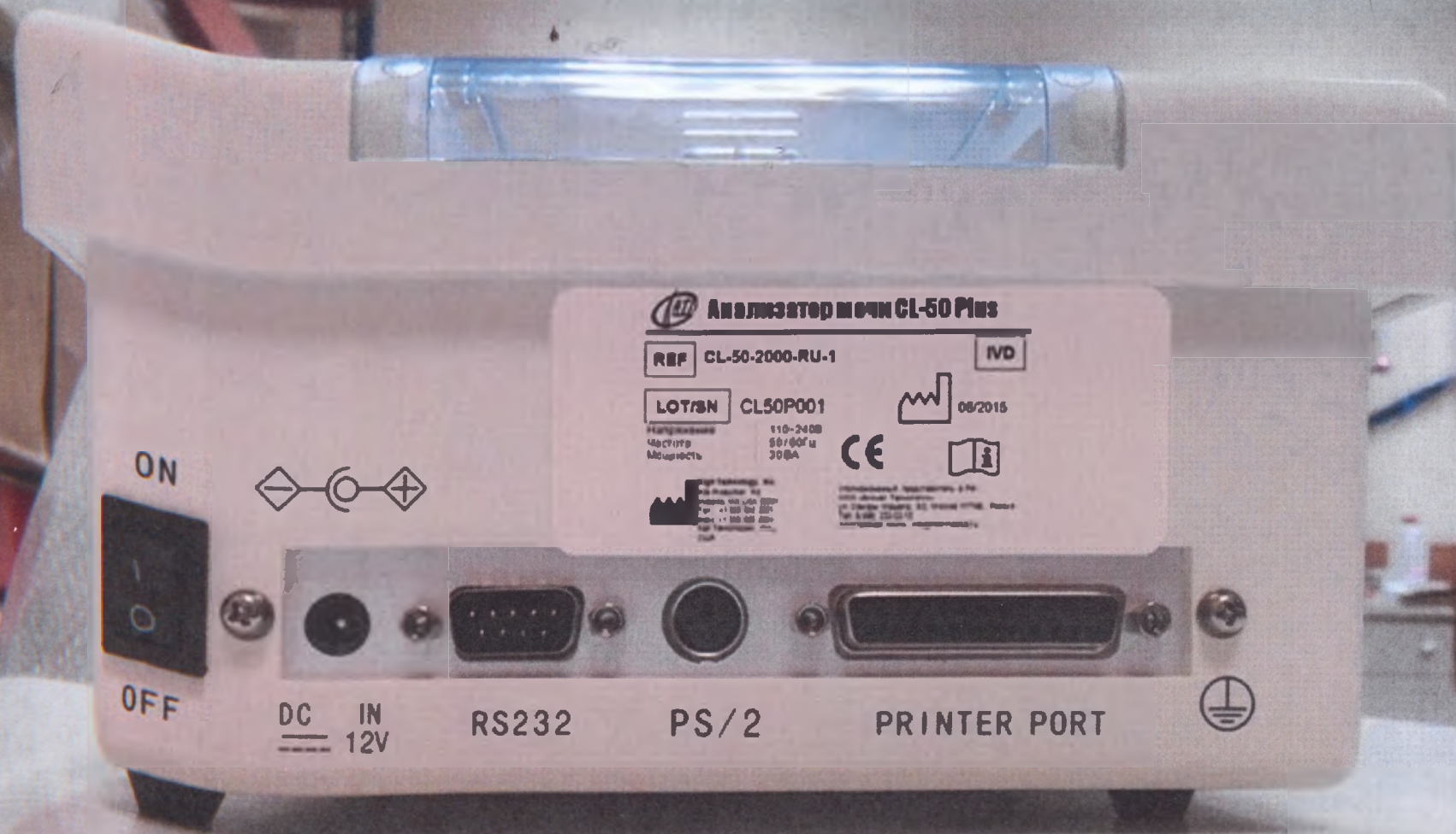
Анализатор мочи CL-50 Plus (вид сзади)
