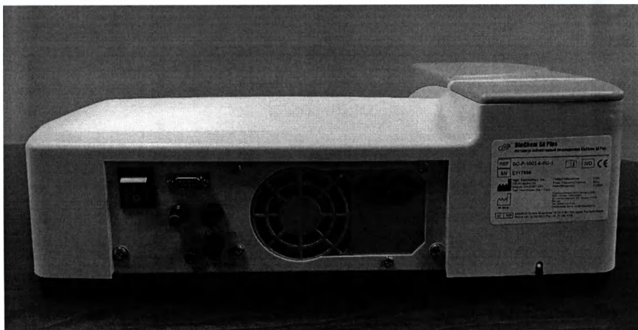
Фото 2. Анализатор биохимический автоматический BioChem модели . Вид сзади
