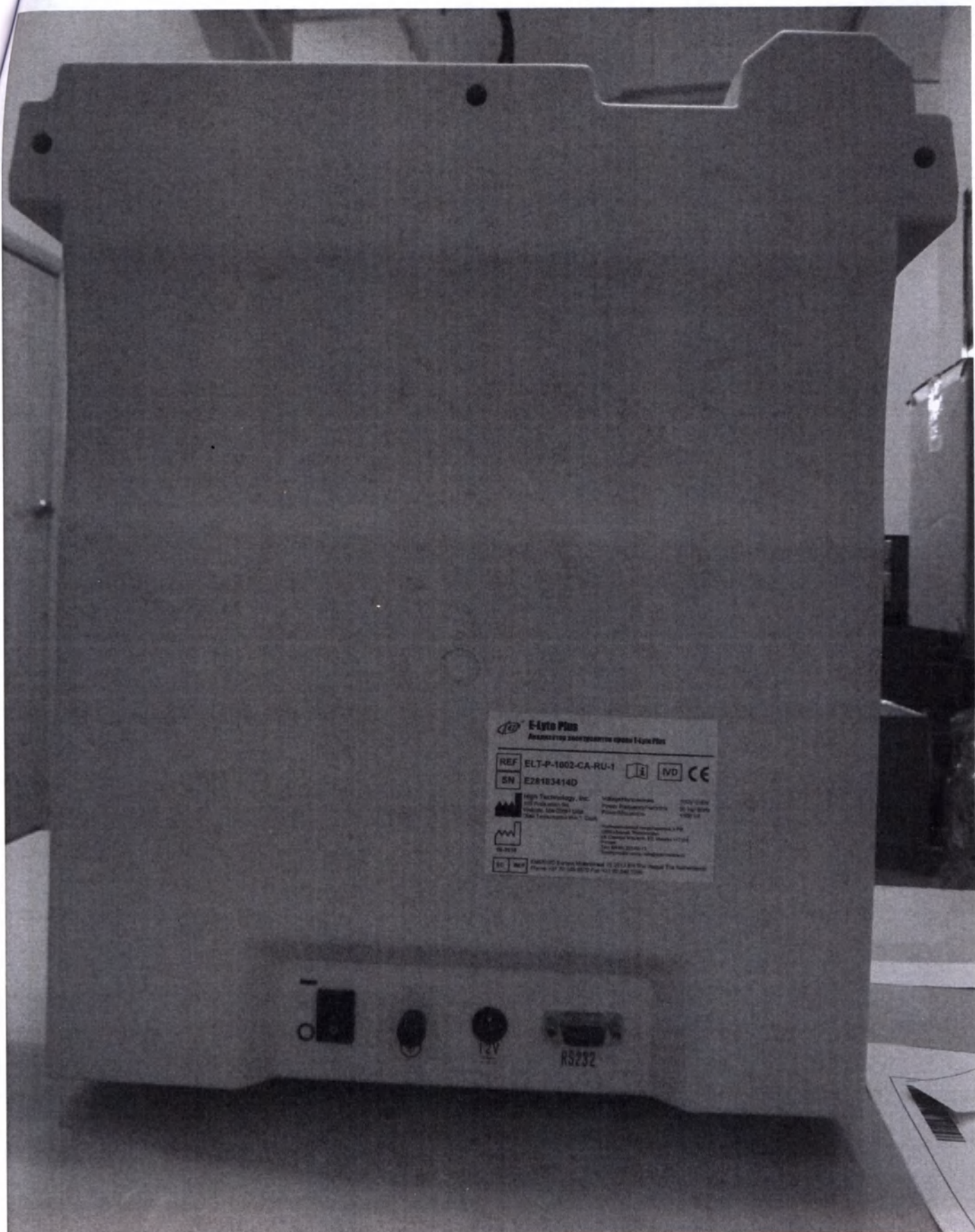
Фото 2. Анализатор электролитов крови E-Lyte Plus. Вид сзади.
