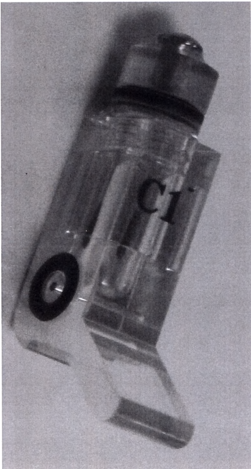
Фото 9. Электрод, Cl
