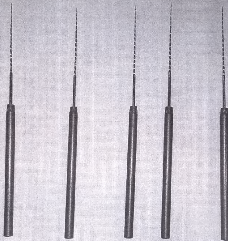
Каналорасширители зубные КрЗ - "КМИЗ", тип К для прямого наконечника
