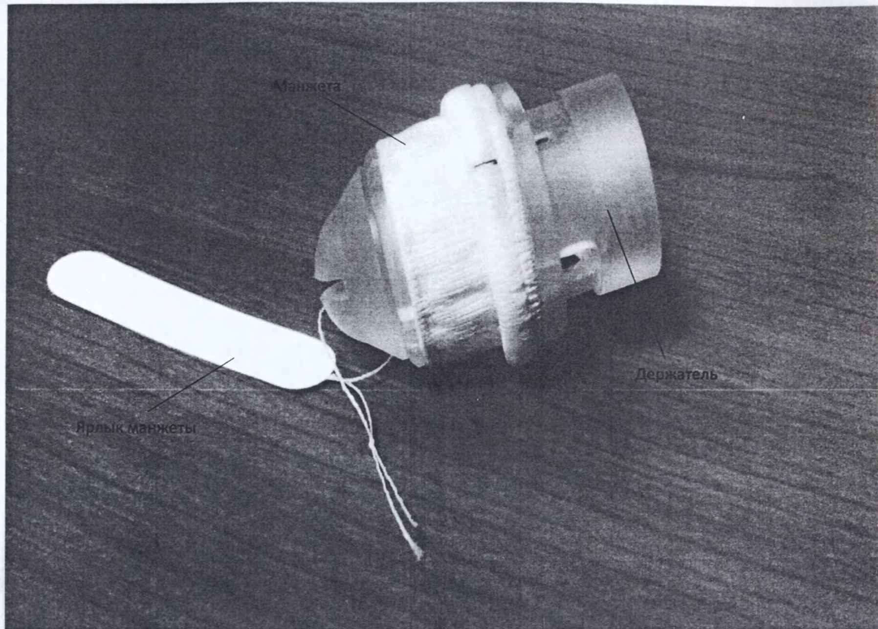
Присоединяемая манжета протеза клапана сердца с бесшовной фиксацией «МЕДИНЖ» ТУ 9444-023-27771122-2016: Общий вид изделия, манжета, закрепленная на держателе
