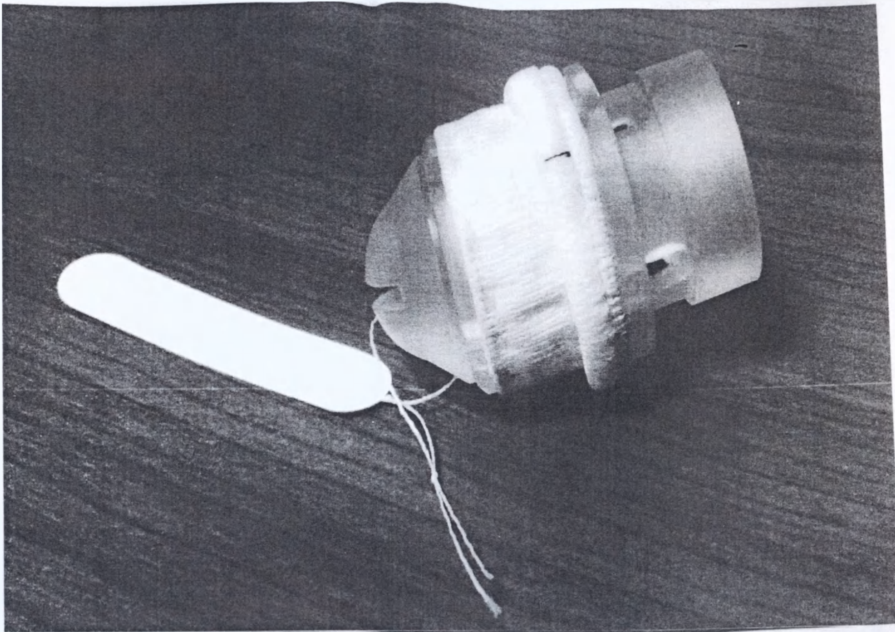
Присоединяемая манжета протеза клапана сердца с бесшовной фиксацией «МЕДИНЖ» ТУ 9444-023-27771122-2016. Общий вид изделия, манжета модели аортальная, формы интрасупрааннулярная
