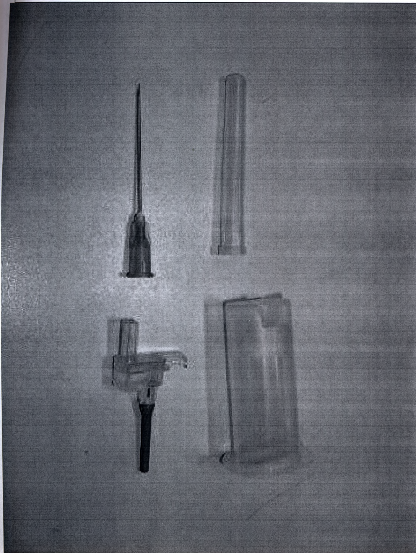
Z-образная игла (игла со смещенным центром и присоединенным держателем Improvacuter) (Off-center collection set Improvacuter)
