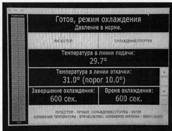
Панель управления
