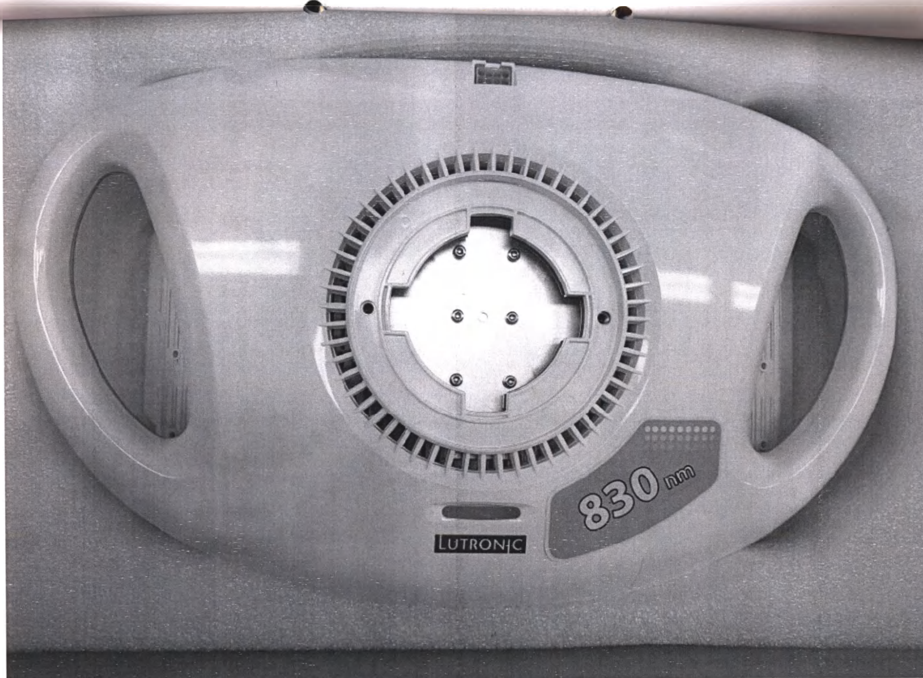
Аппарат фототерапевтический HEALITE II: Блок-лампа на 830/590 нм
