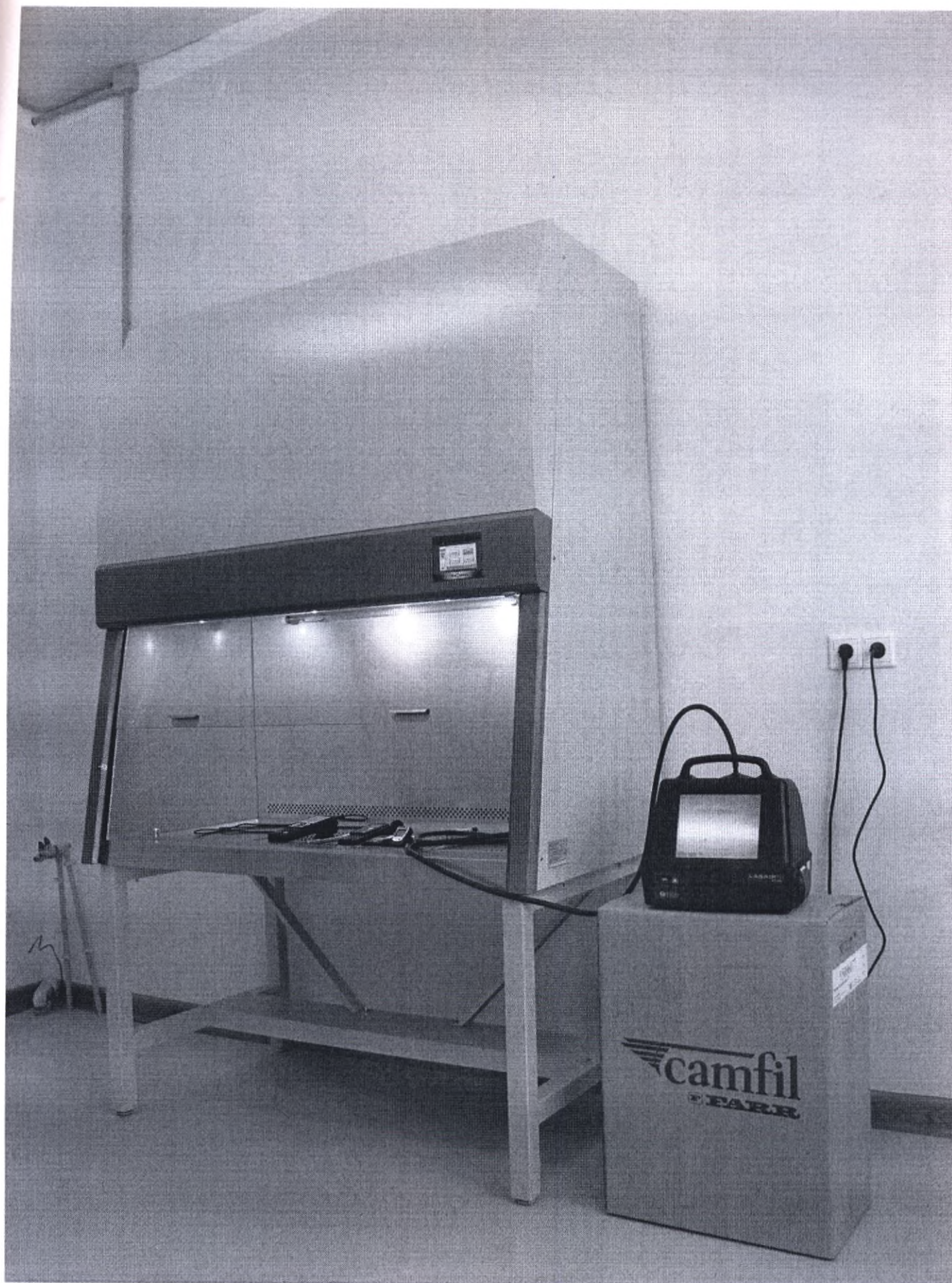
Фото 3 - Шкаф ламинарный серии BA-safe, вариант исполнения BA-safe 1,5
