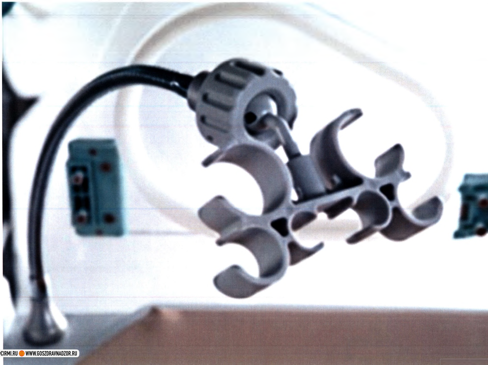
6. Держатель шлангов внутри инкубатора.
