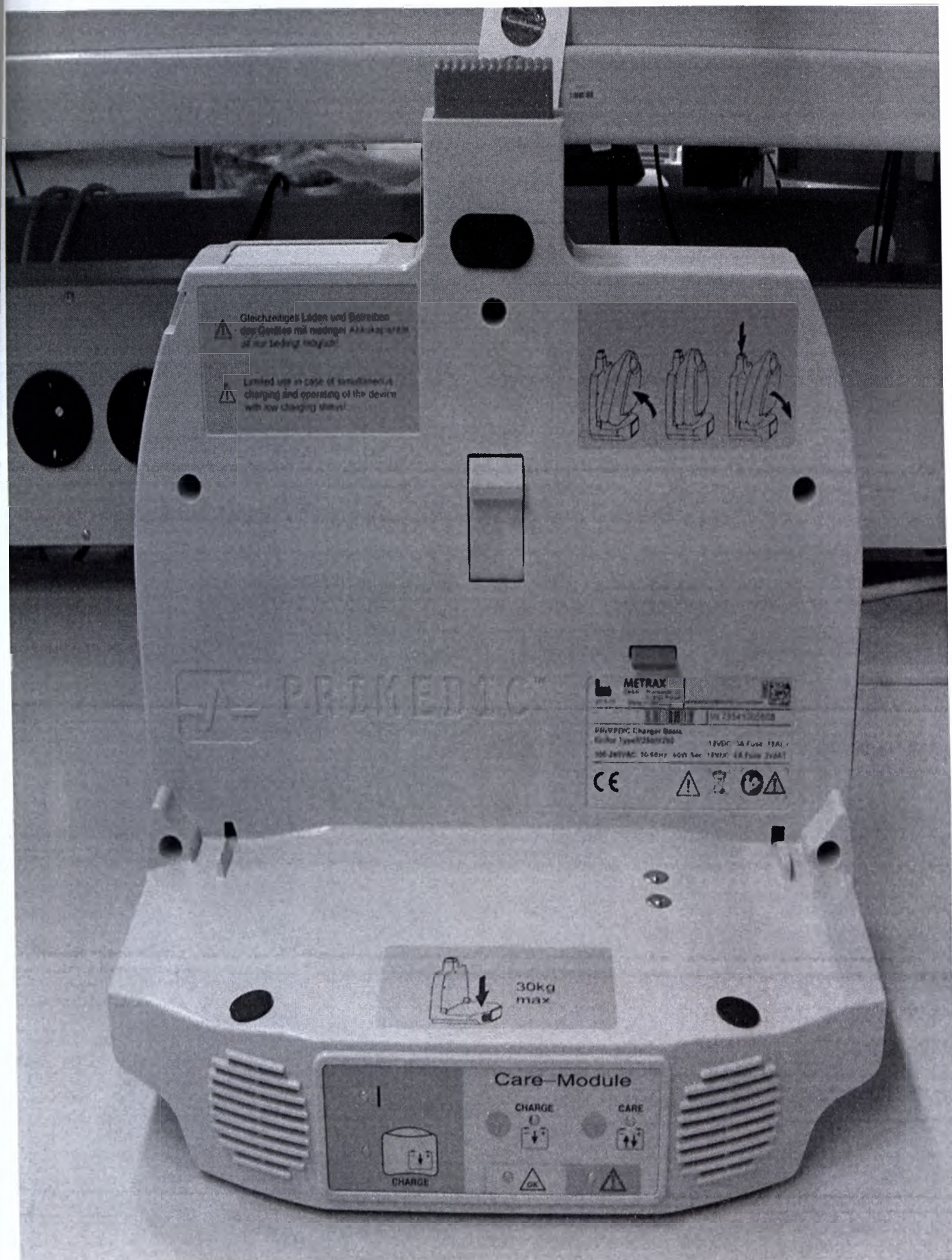
Зарядная консоль PRIMEDIC Charger Basis
