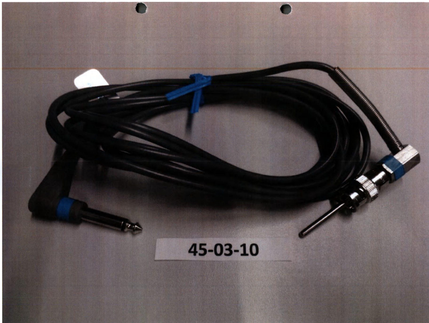
Датчик температурный для прямого измерения температуры крови в оксигенаторах
