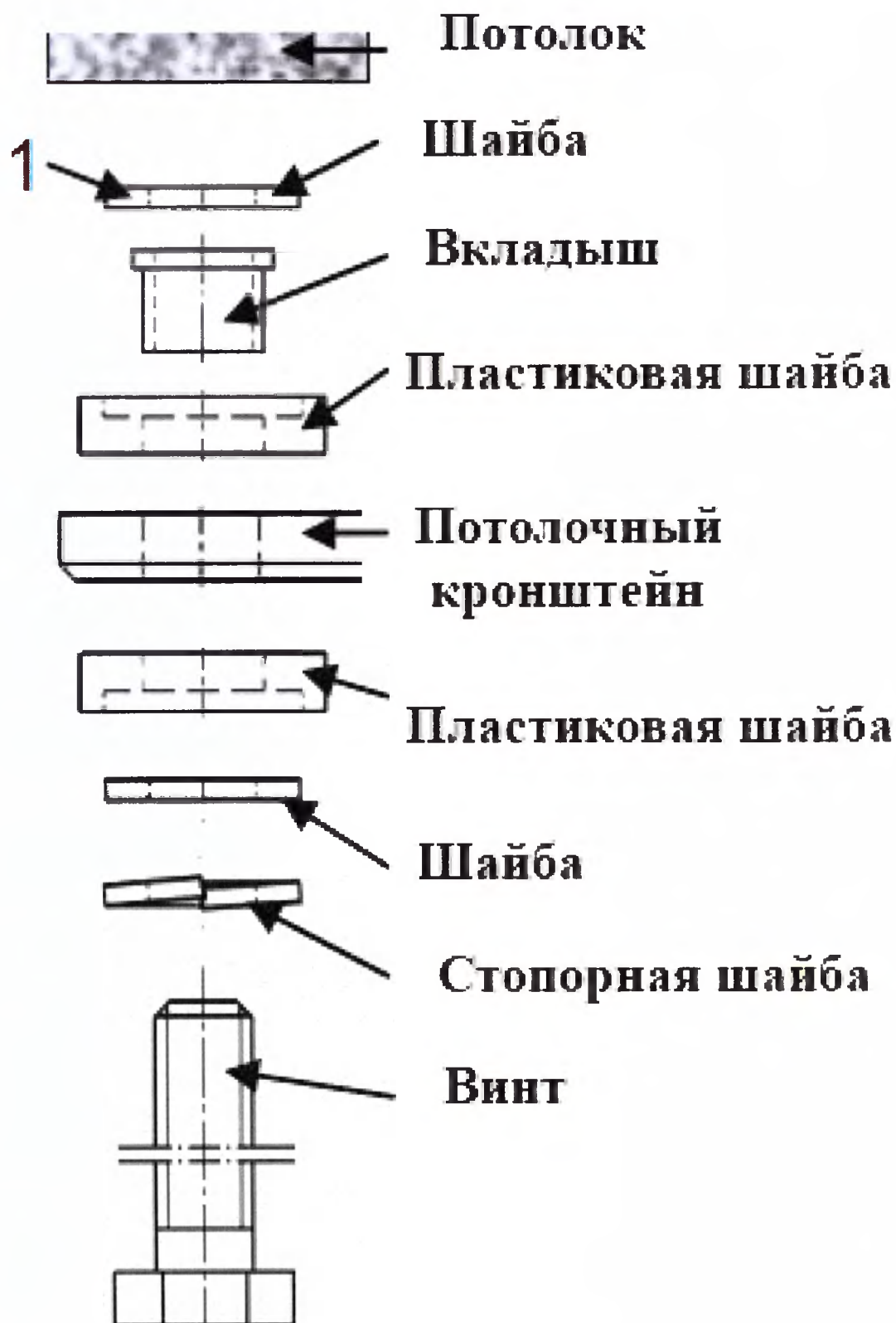
Рисунок 7 - Комплект крепежный: потолочный, настенный
