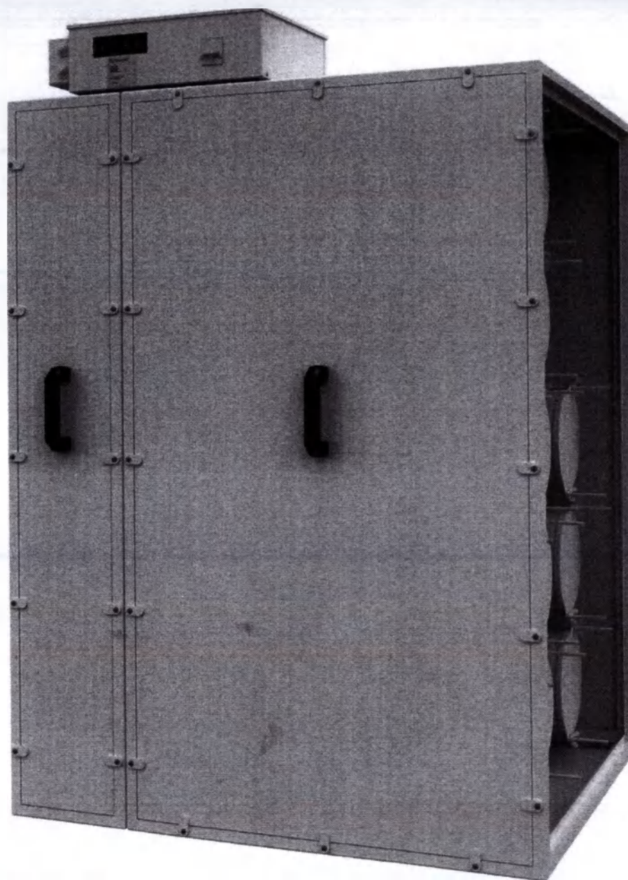
Обеззараживатель-очиститель воздуха «Тион В150х1950»
