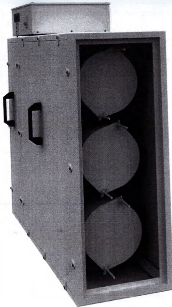
Обеззараживатель-очиститель воздуха «Тион В150х450»
