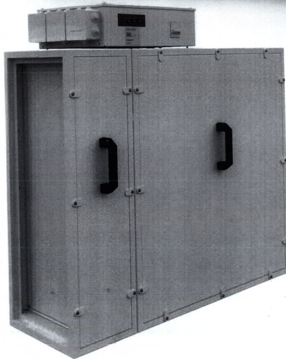
Обеззараживатель-очиститель воздуха «Тион В150х450»
