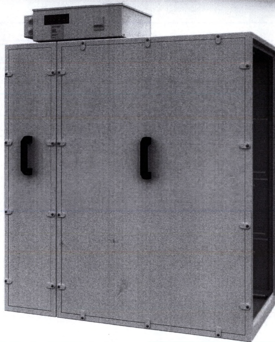
Обеззараживатель-очиститель воздуха «Тион В150х1050»
