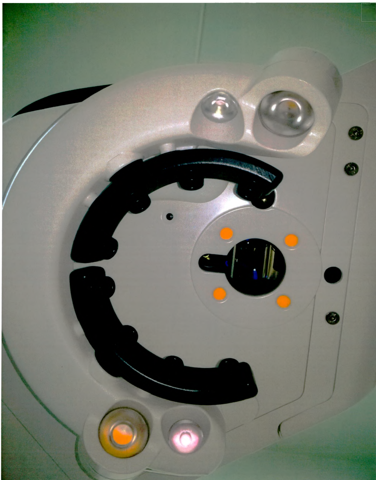
Осветительный блок, крышка кольцевого освещения, иллюминация монтажной пластины, инфракрасный индикатор оптического фокуса, левое и правое впускные сопла шлейфа (№ п/п 90, 91, 92, 94, 134, 135)
