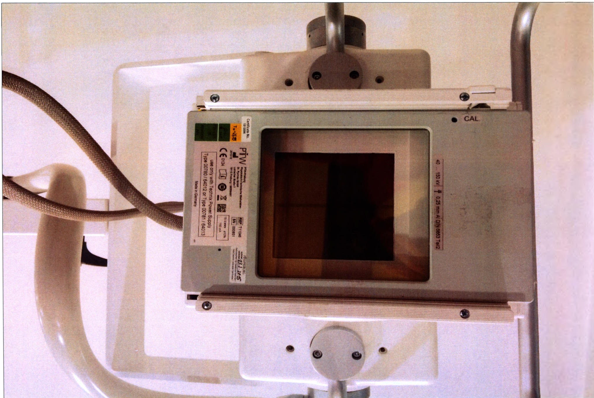
3. Дозиметр DAP.
