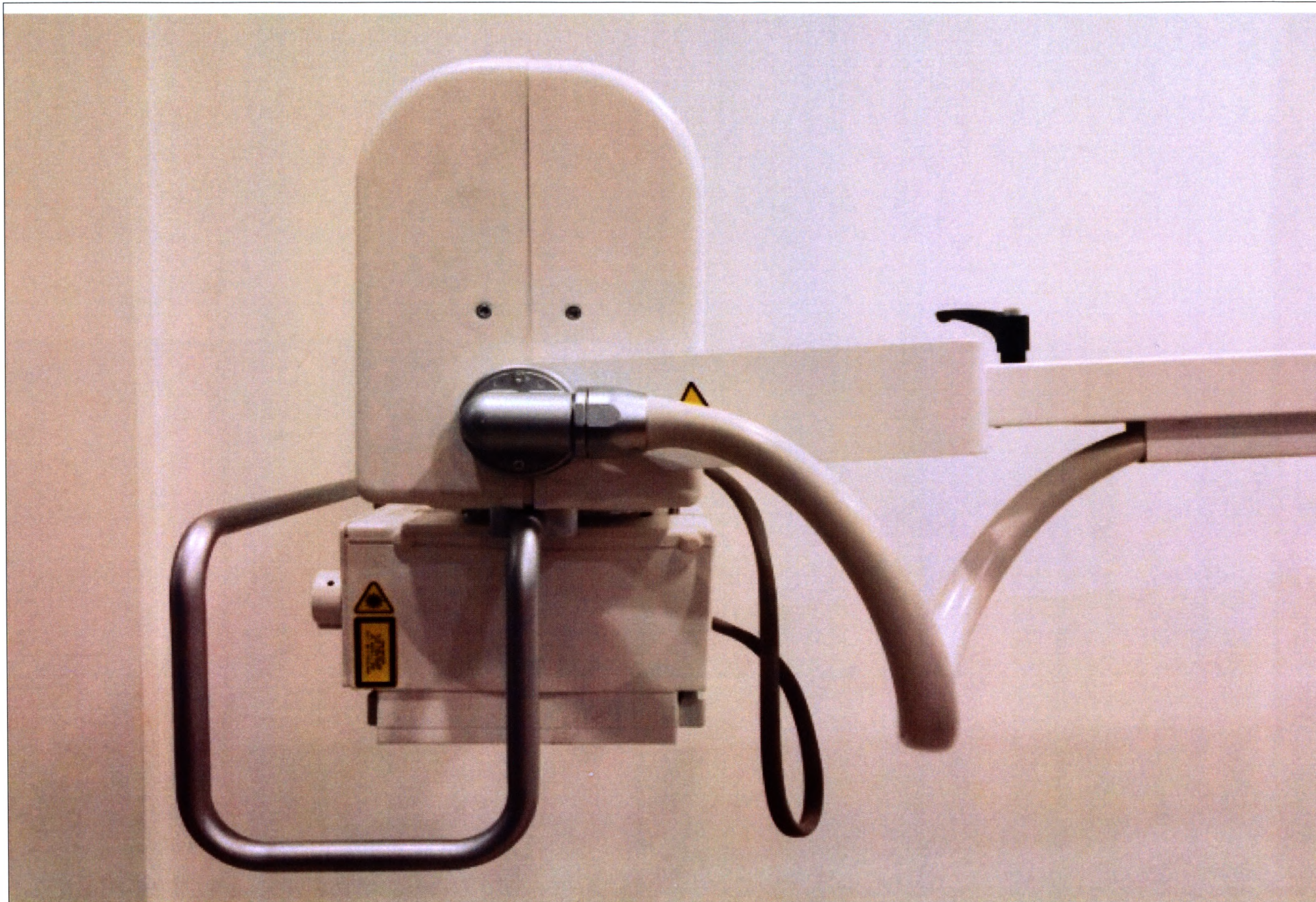
1б. Моноблок: 1.1 Рентгеновская трубка; 1.2 Генератор 16кВт/32 кВт; 1.3 Кронштейн трубки.
