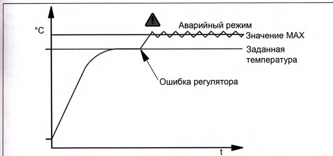
Рис. 17 Схематическое изображение процесса контроля температуры с помощью TWW
