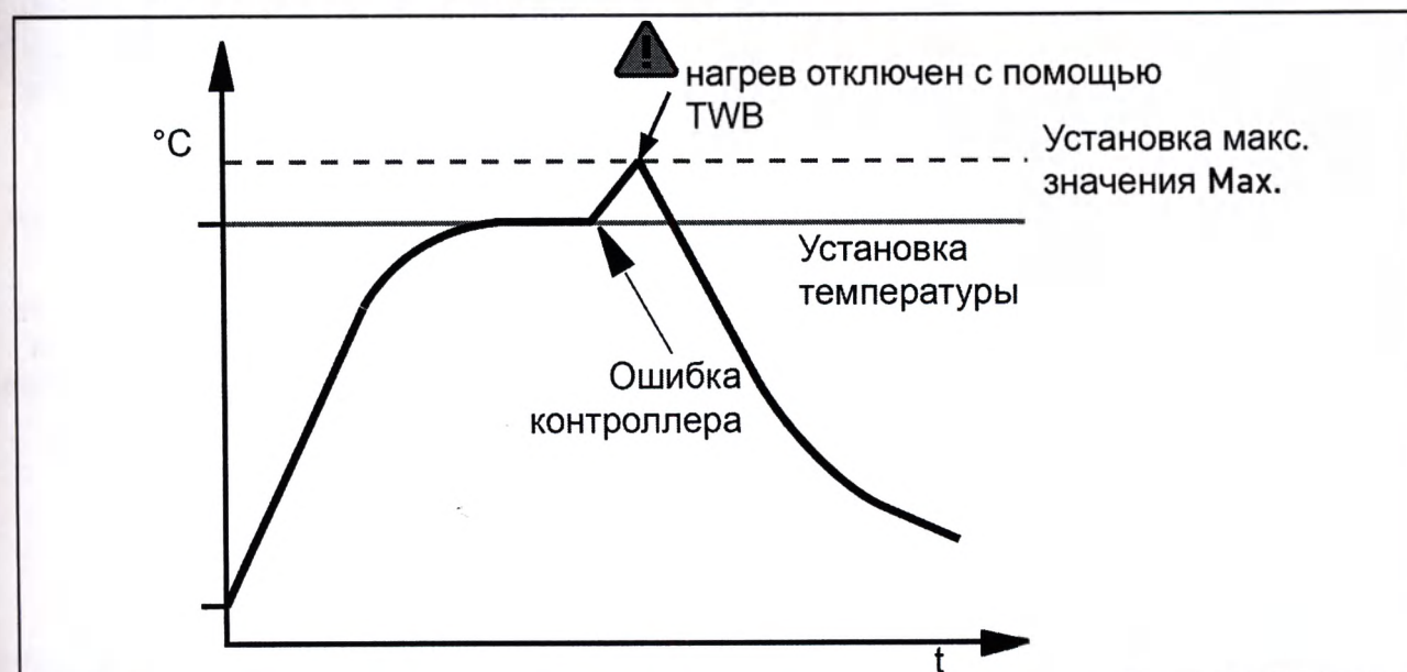
Рис. 18 Схематическое изображение процесса контроля температуры с помощью TWB
