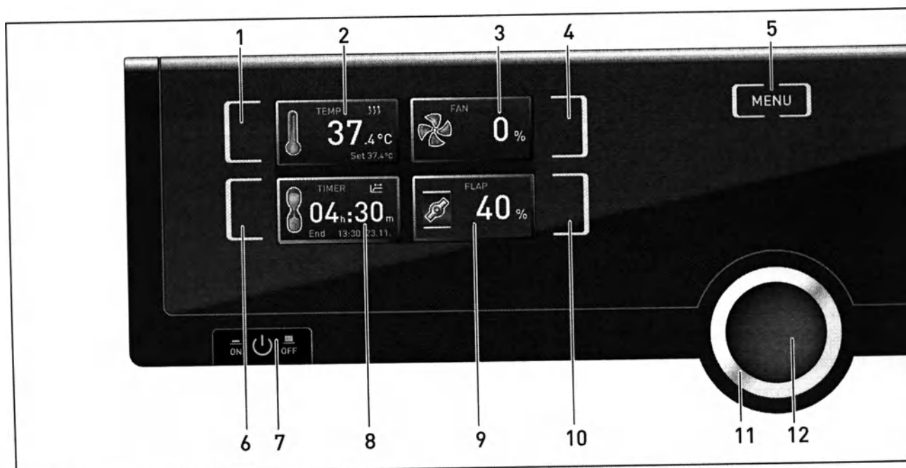
Рис. 14 Панель ControlCOCKPIT устройств IFxx в режиме эксплуатации
