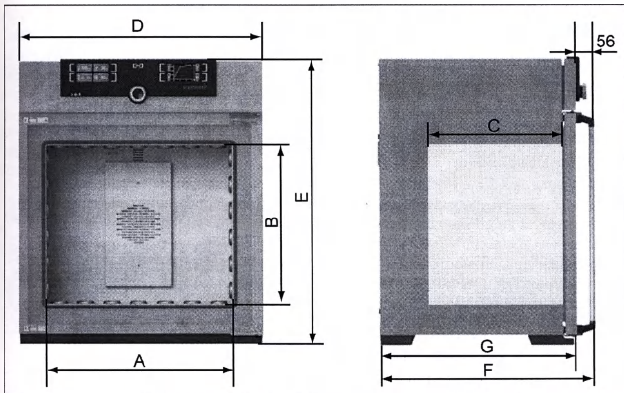
Рис. 7 Размеры
