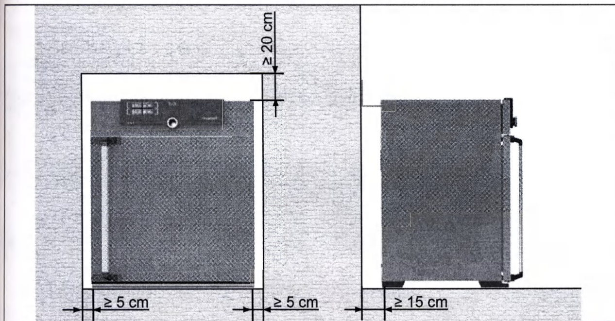
Рис. 8 Минимальные расстояния для стен и потолка
