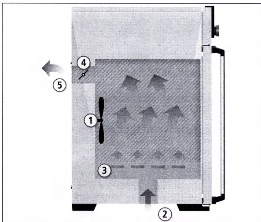
Рис. 3 Принципы работы
