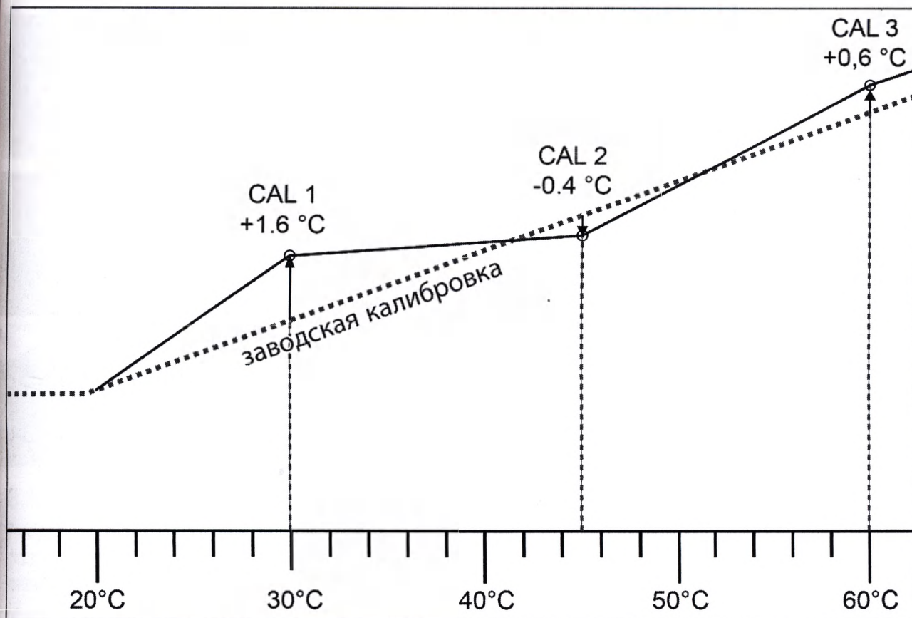
Рис. 23 Схематический пример точной настройки температуры
