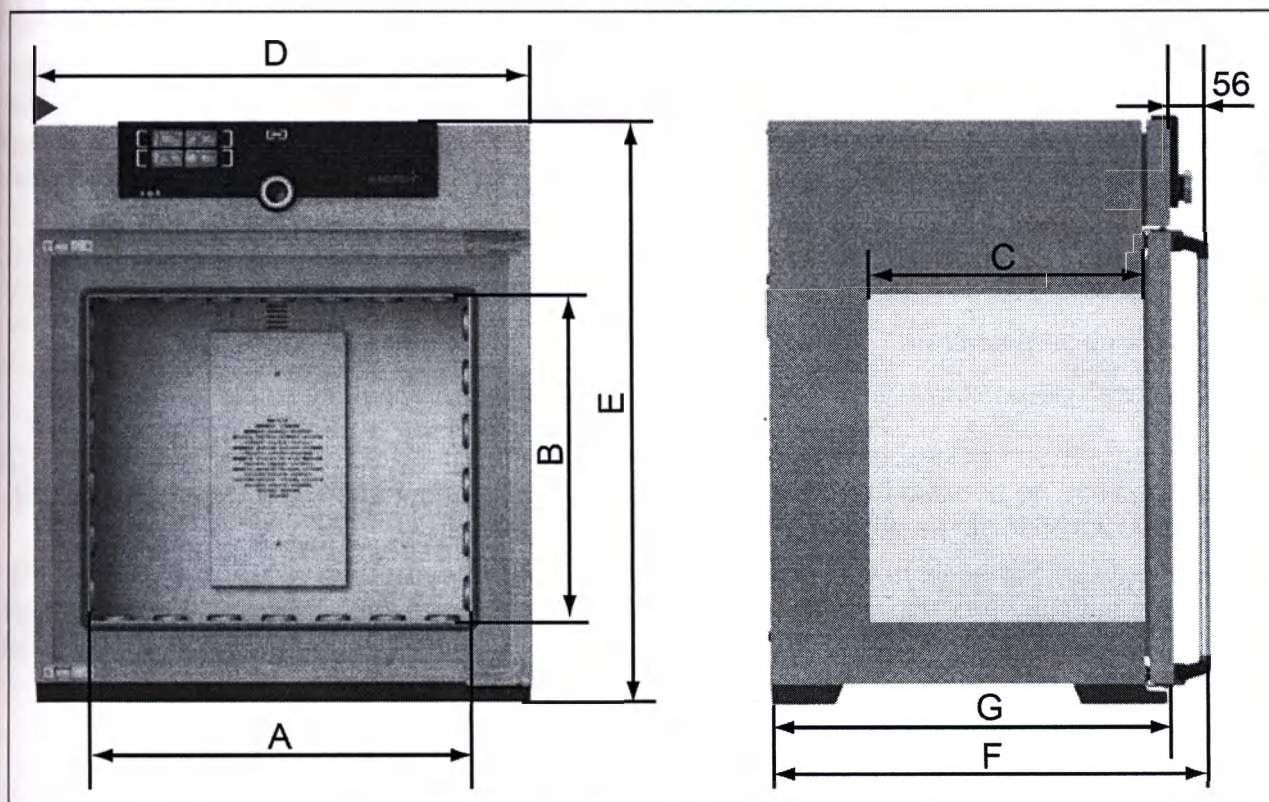
Рис. 6 Размеры
