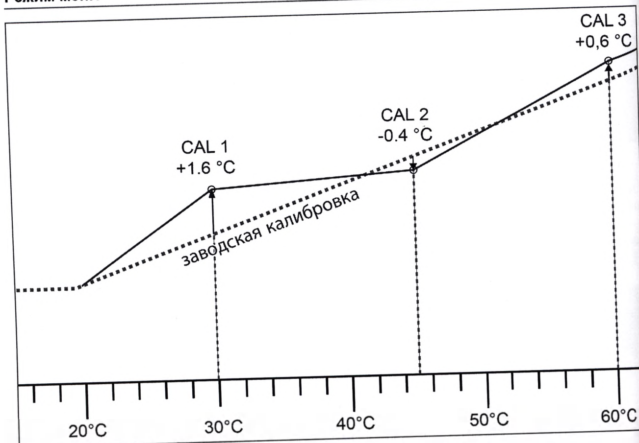
Рис. 25 Схематический пример точной настройки температуры
