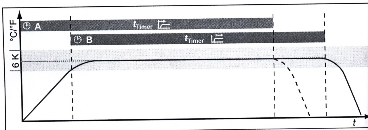
Рис. 23 Режим таймера
