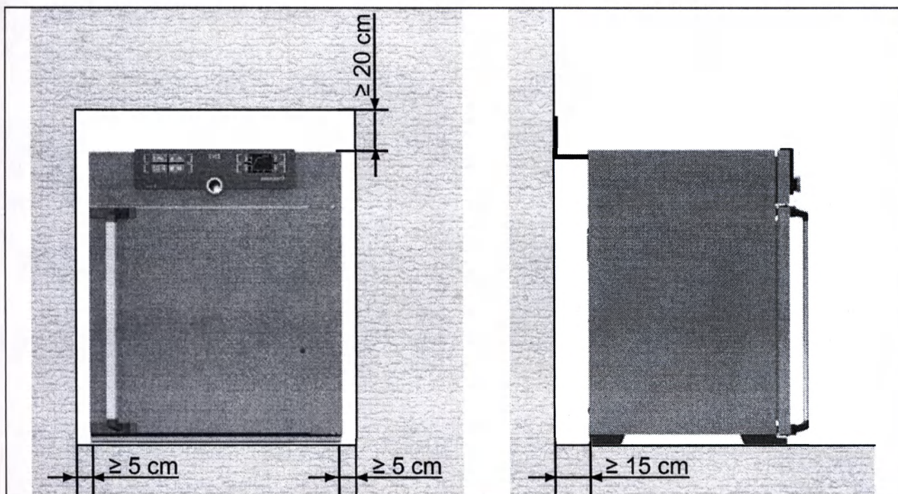
Рис. 8 Минимальные расстояния для стен и потолка
