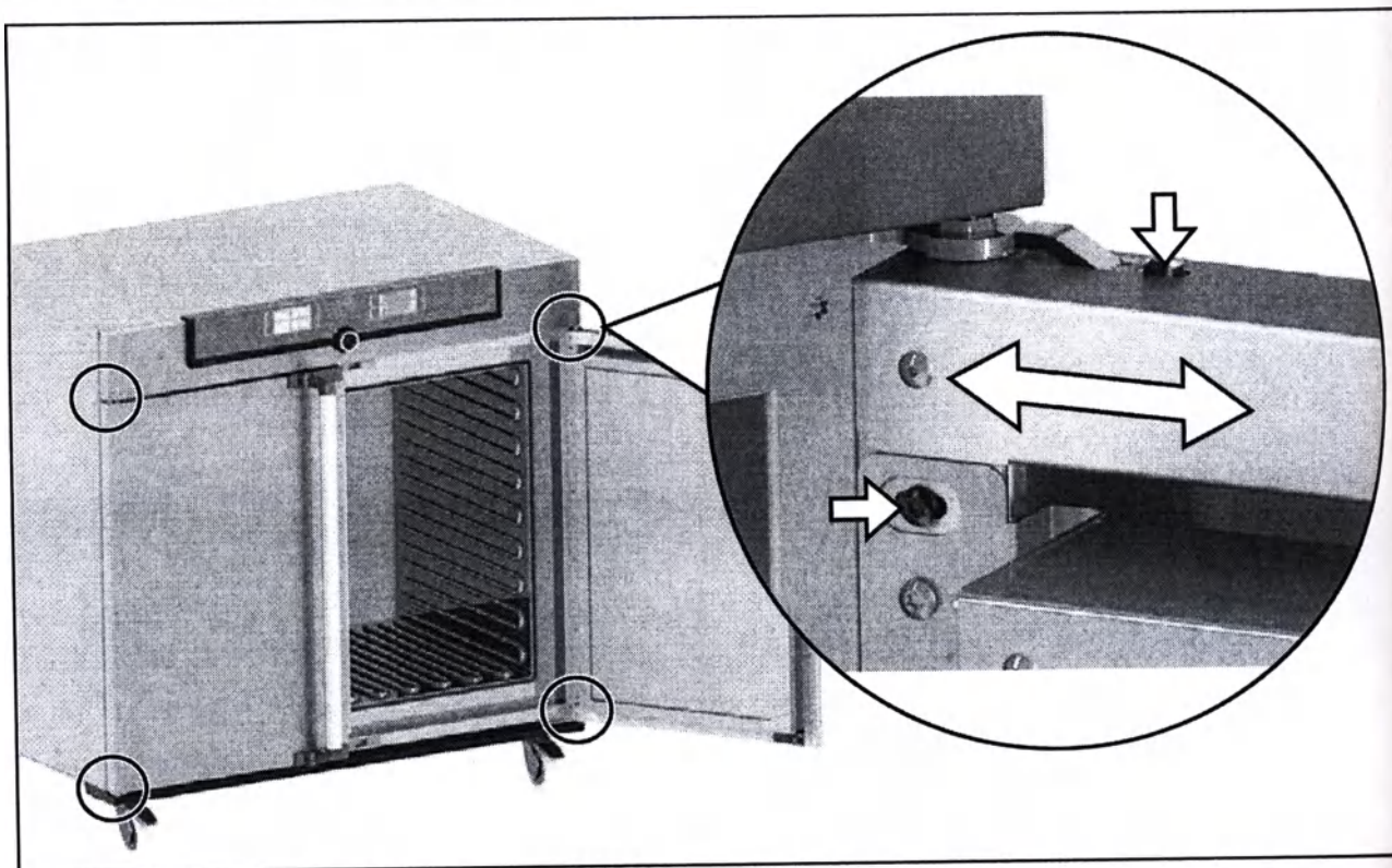
Рис. 9 Регулировка дверцы
