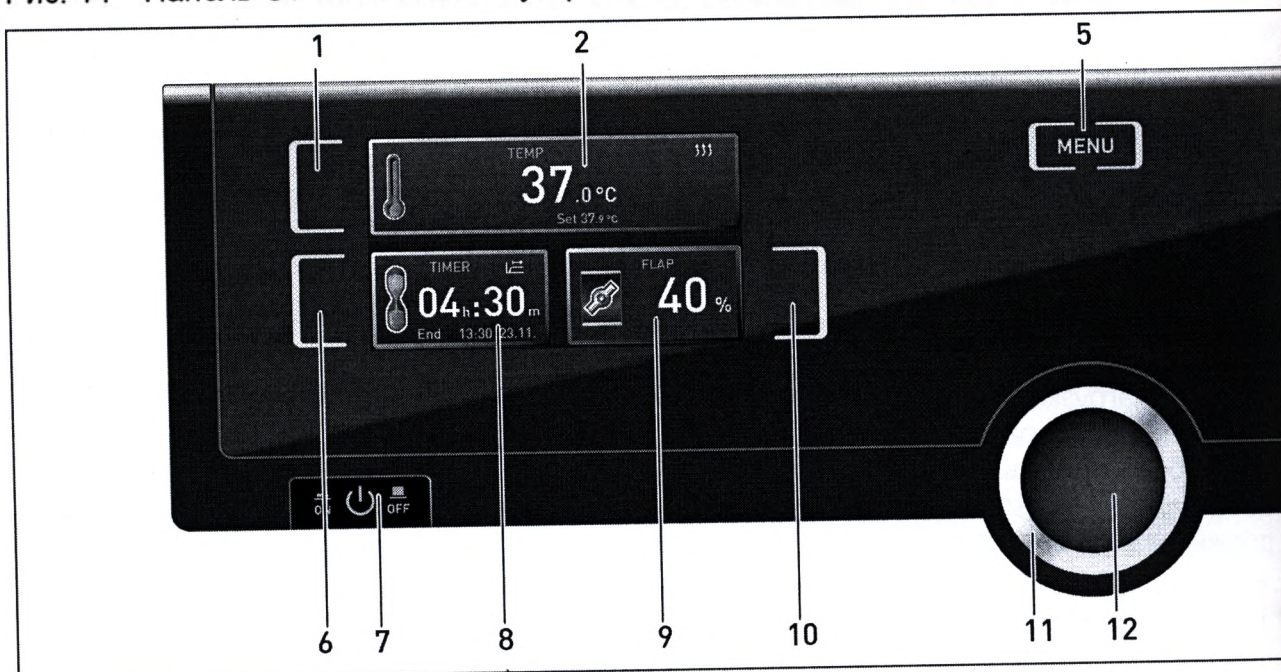
Рис. 15 Панель ControlCOCKPIT устройств INxx в режиме эксплуатации
