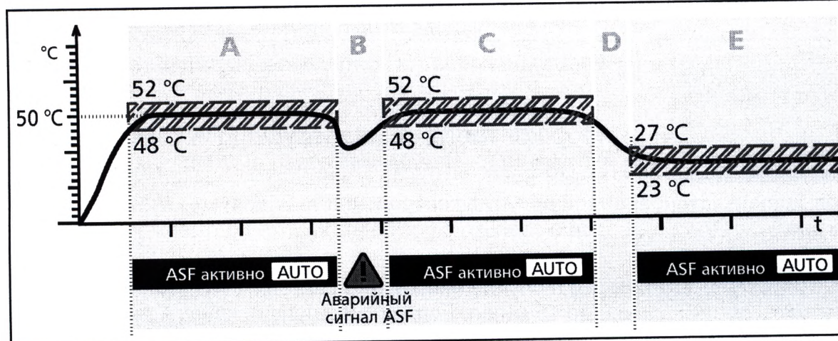
Рис. 19 Схематическое изображение процесса контроля температуры с помощью ASF
