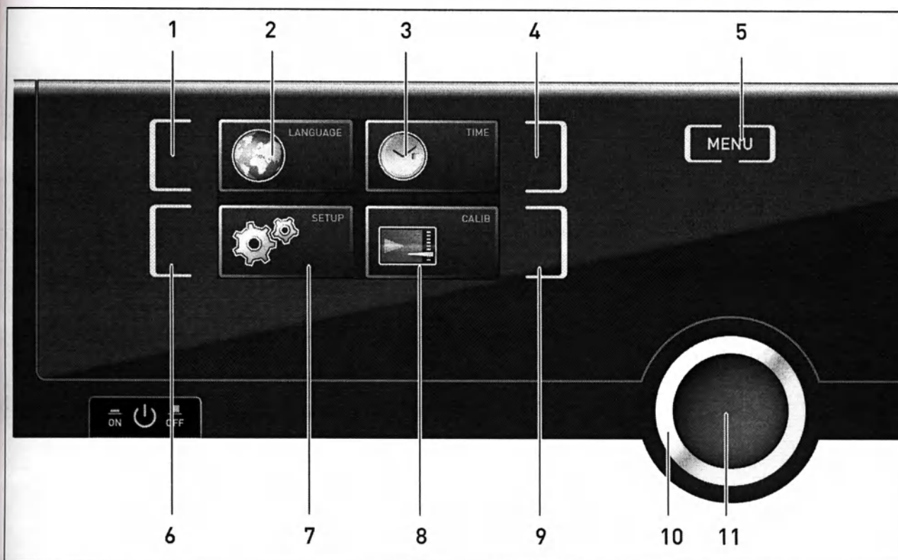
Рис. 20 ControlCOCKPIT в режиме меню
