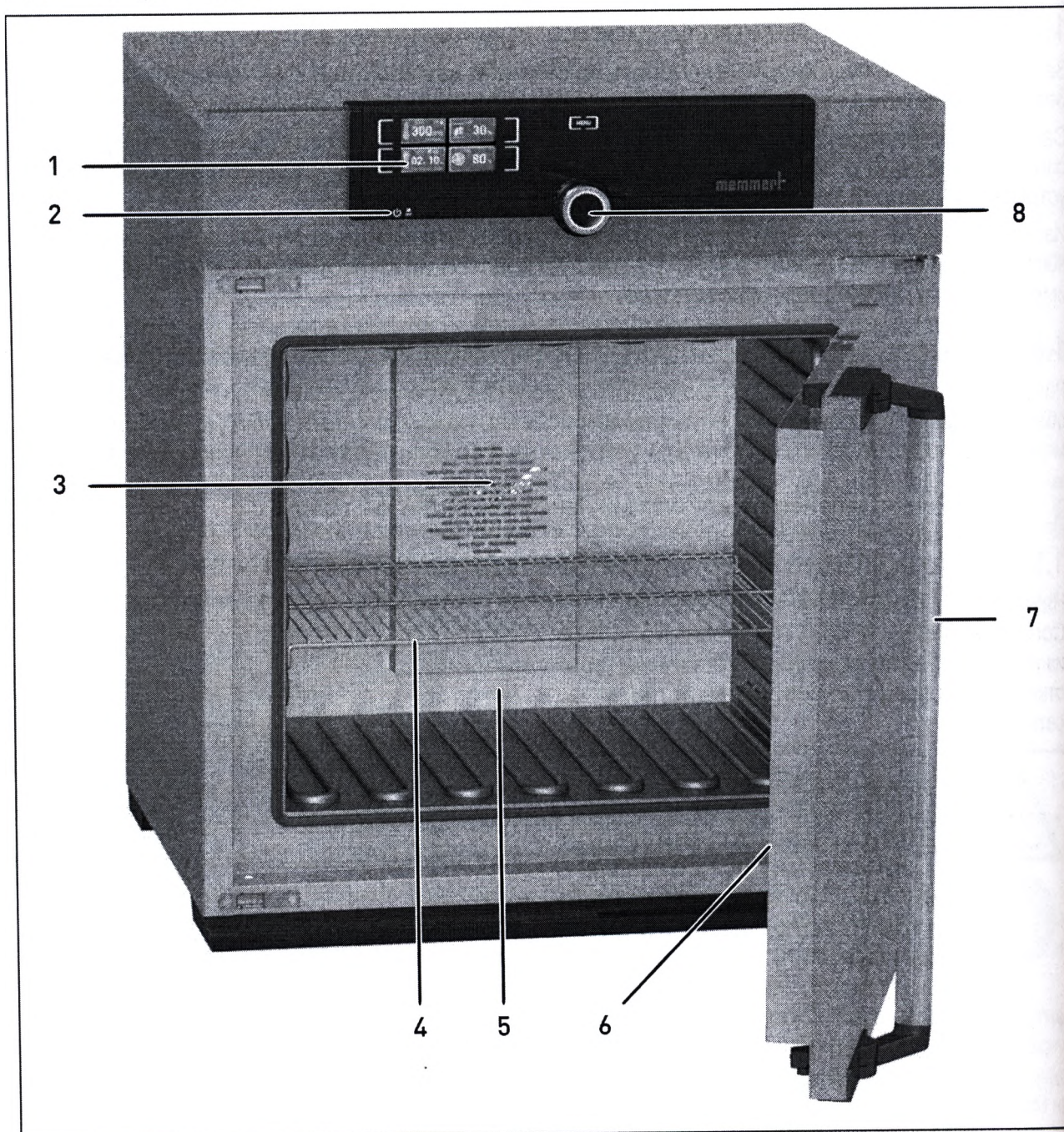
Рис. 2 Устройство
