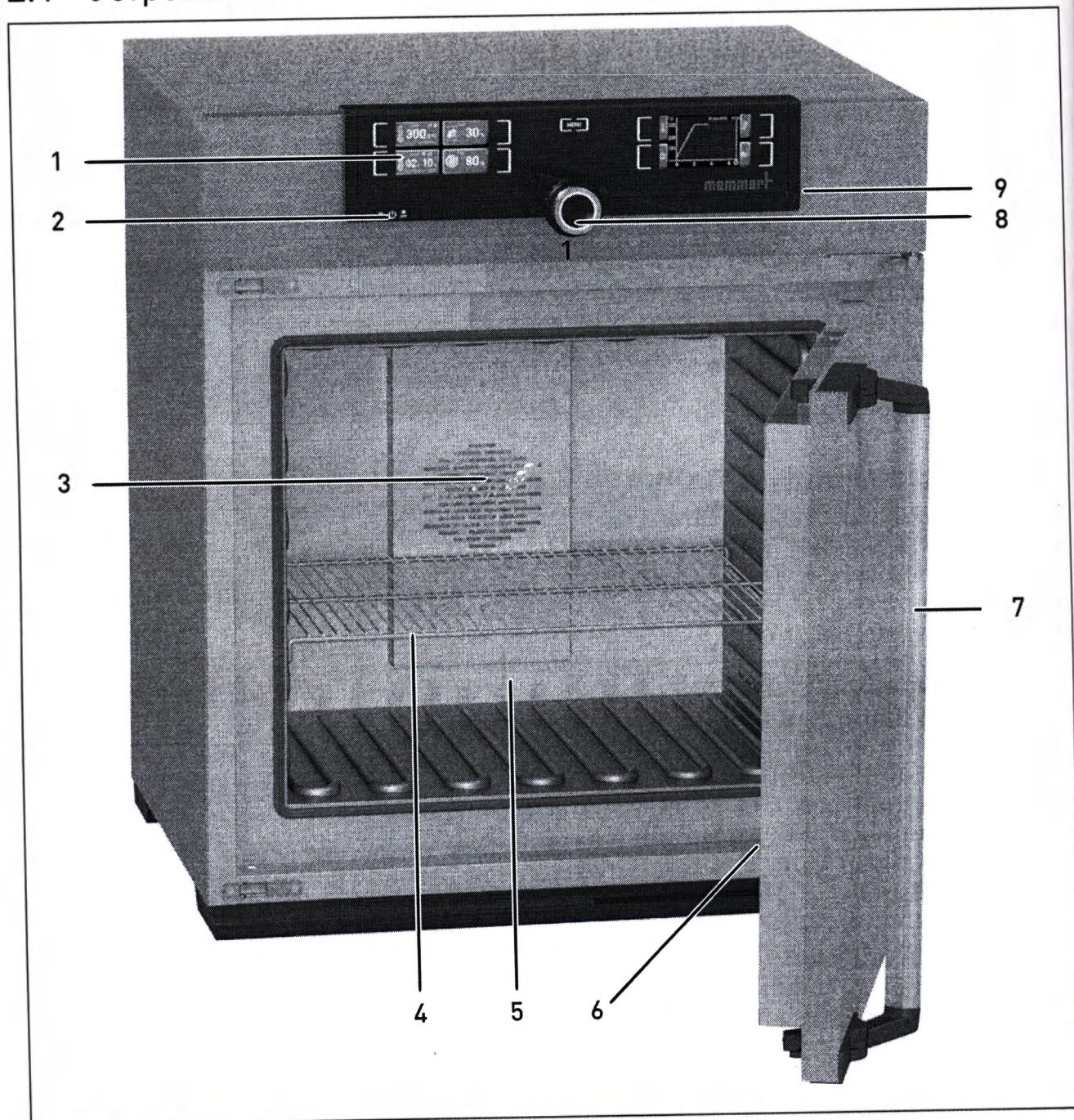
Рис. 2 Устройство
