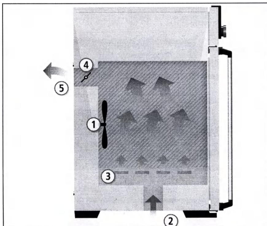
Рис. 3 Принципы работы
