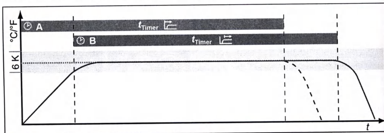
Рис. 22 Режим таймера
