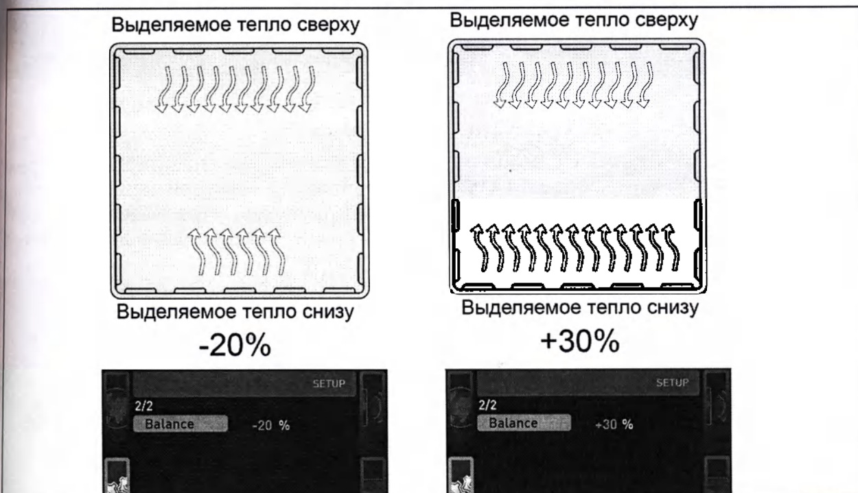
Рис. 24 Распределение теплопроизводительности (пример): при настройке -20\% (слева) теплопроизводительность нижней группы нагревателей на 20\% ниже, чем верхней. При настройке +30\% (справа) теплопроизводительность нижней группы нагревателей на 30\% выше, чем верхней. Настройка 0\% восстанавливает заводские настройки теплопроизводительности.
