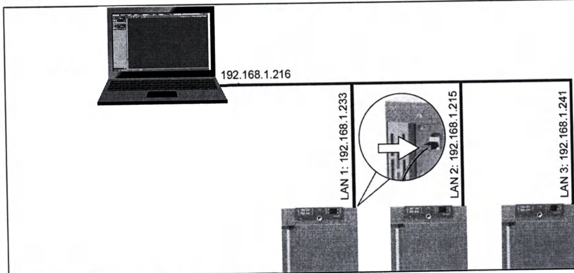
Рис. 22 Эксплуатация нескольких устройств в одной сети (схематический пример)
