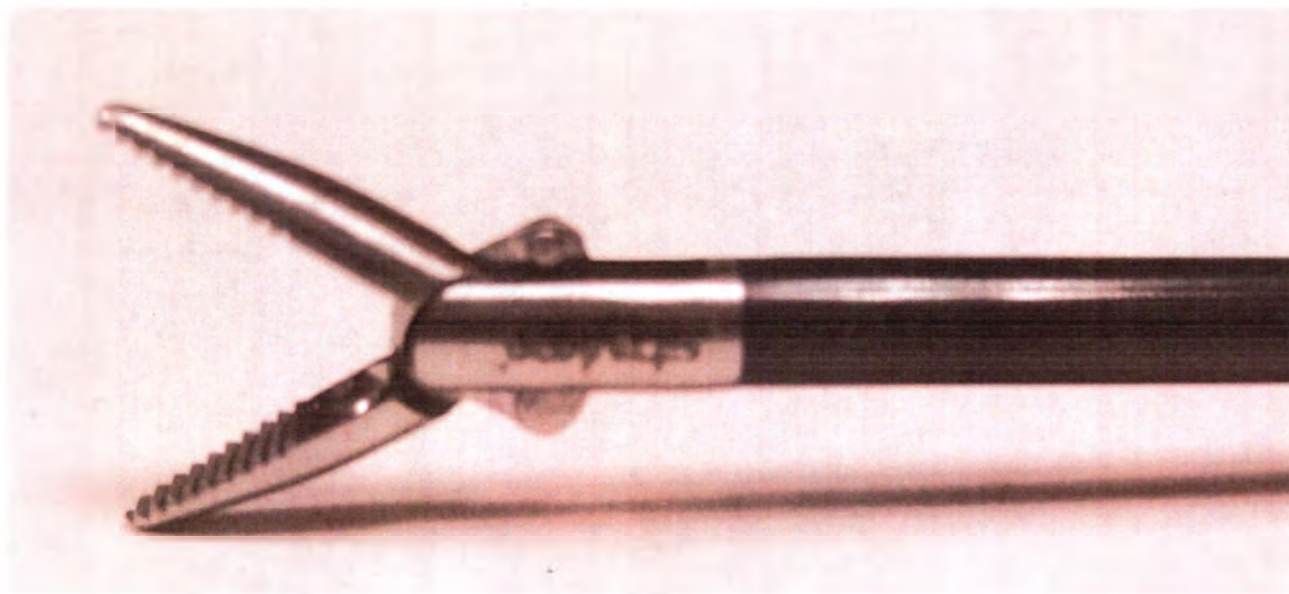
Вставка «щипцы-диссектор» пулевые, диаметр 3 мм, длина 29 см
