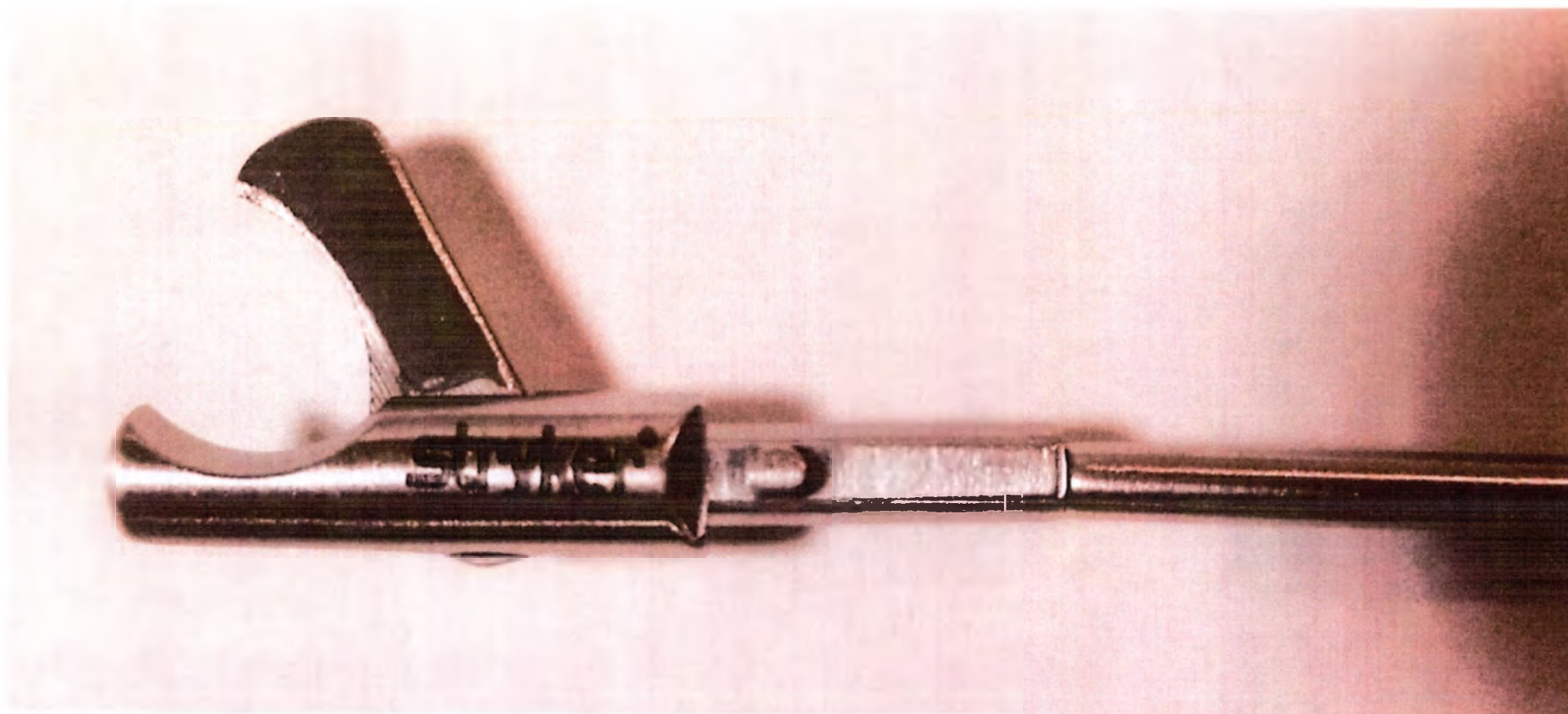
Вставка «ножницы», крючковидные, диаметр 5 мм, длина 33см Вставка «ножницы», крючковидные, диаметр 5 мм, длина 45см
