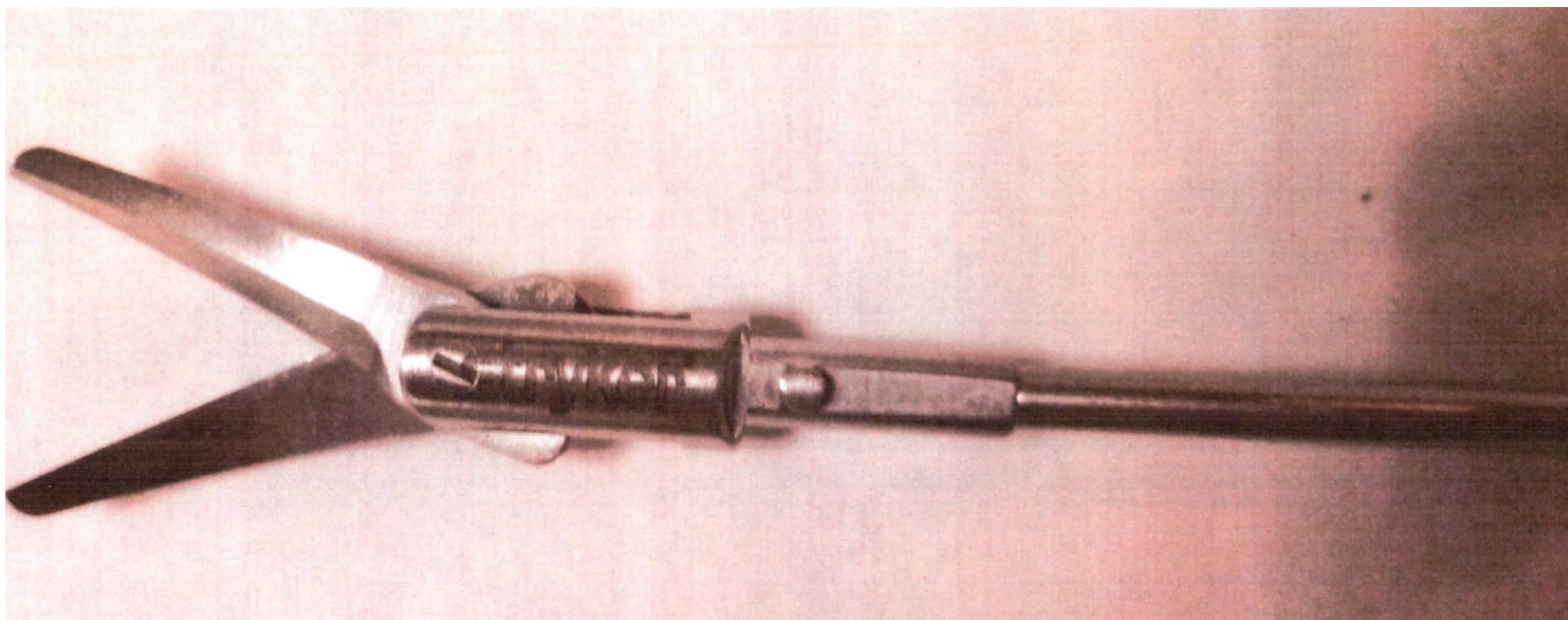
Вставка «ножницы» по Метценбаум, изогнутые, диаметр 5мм, длина 33см Вставка «ножницы» по Метценбаум, изогнутые, диаметр 5 мм, длина 45 см
