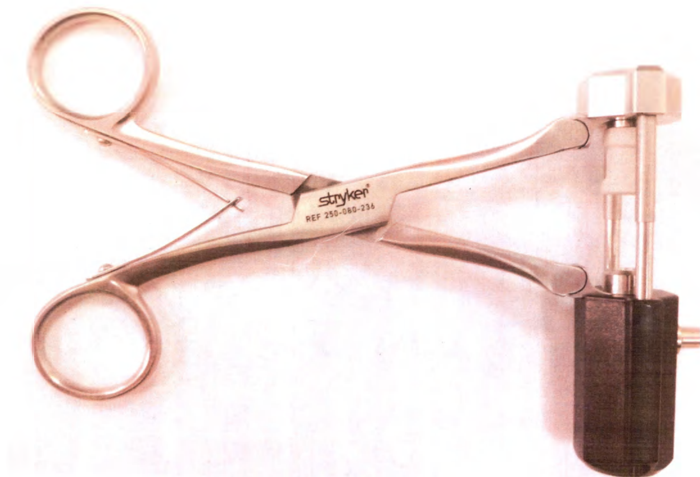
Рукоятка кольцевая биполярная, диаметр 5.0 мм
