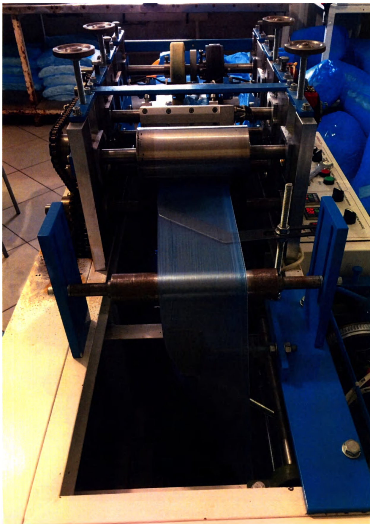
Спайка швов под резинку. Формирование заготовки
