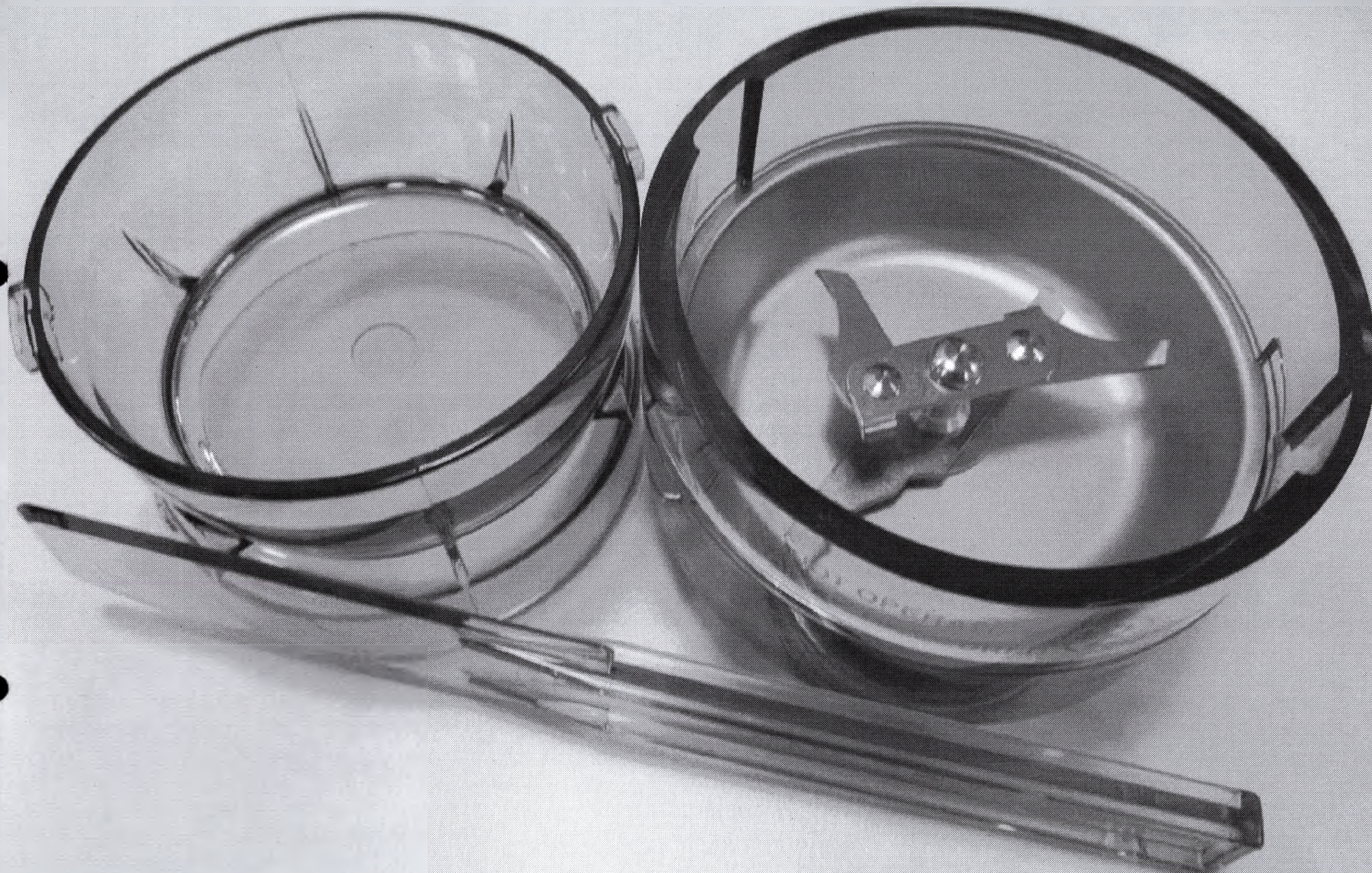
Внешний вид изделия – Лезвие костной мельницы Midas Rex, модель BM210
