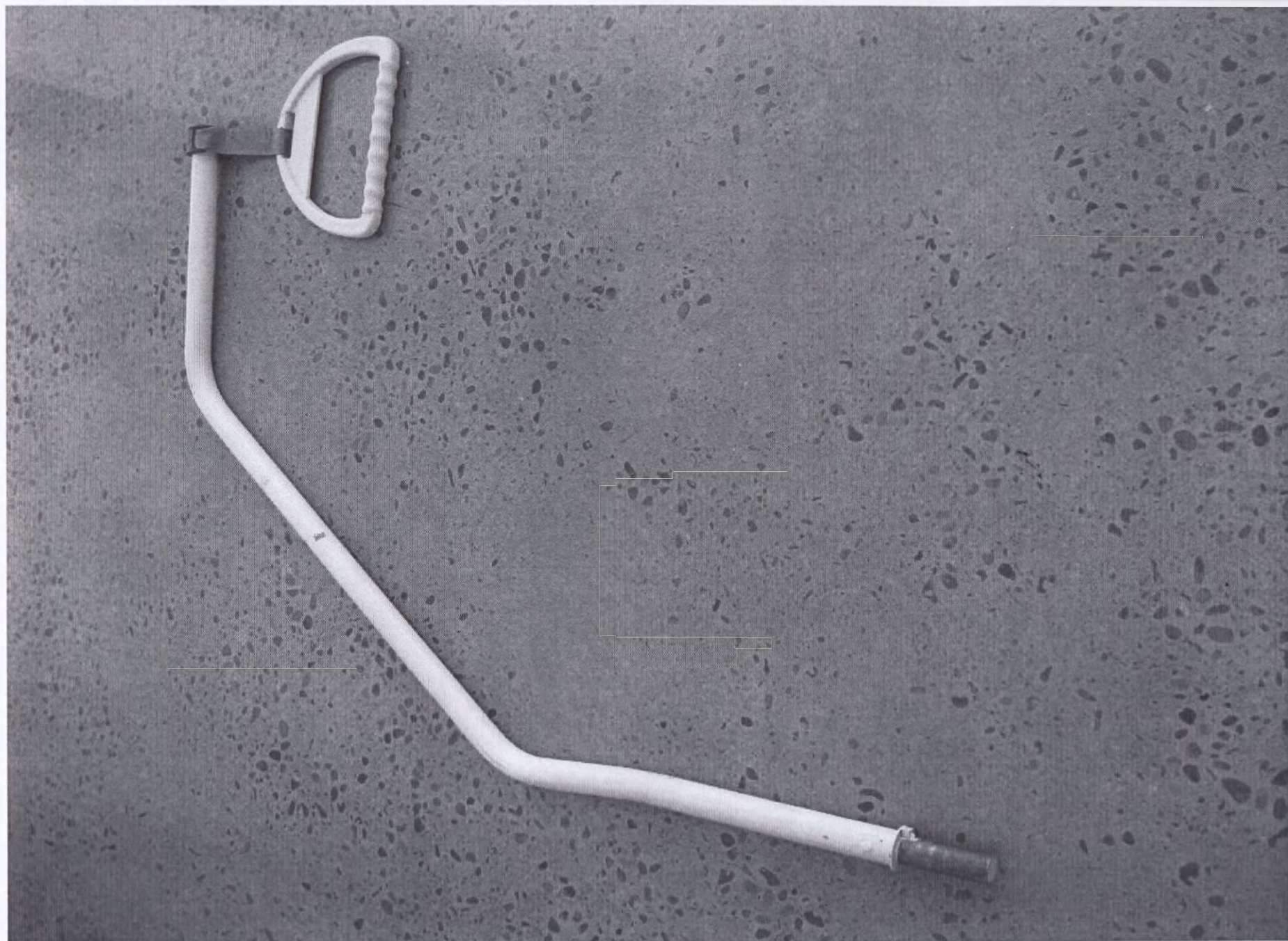
Устройство для поднятия пациента, не регулируемое (PH pole complete (FIXED handle))
