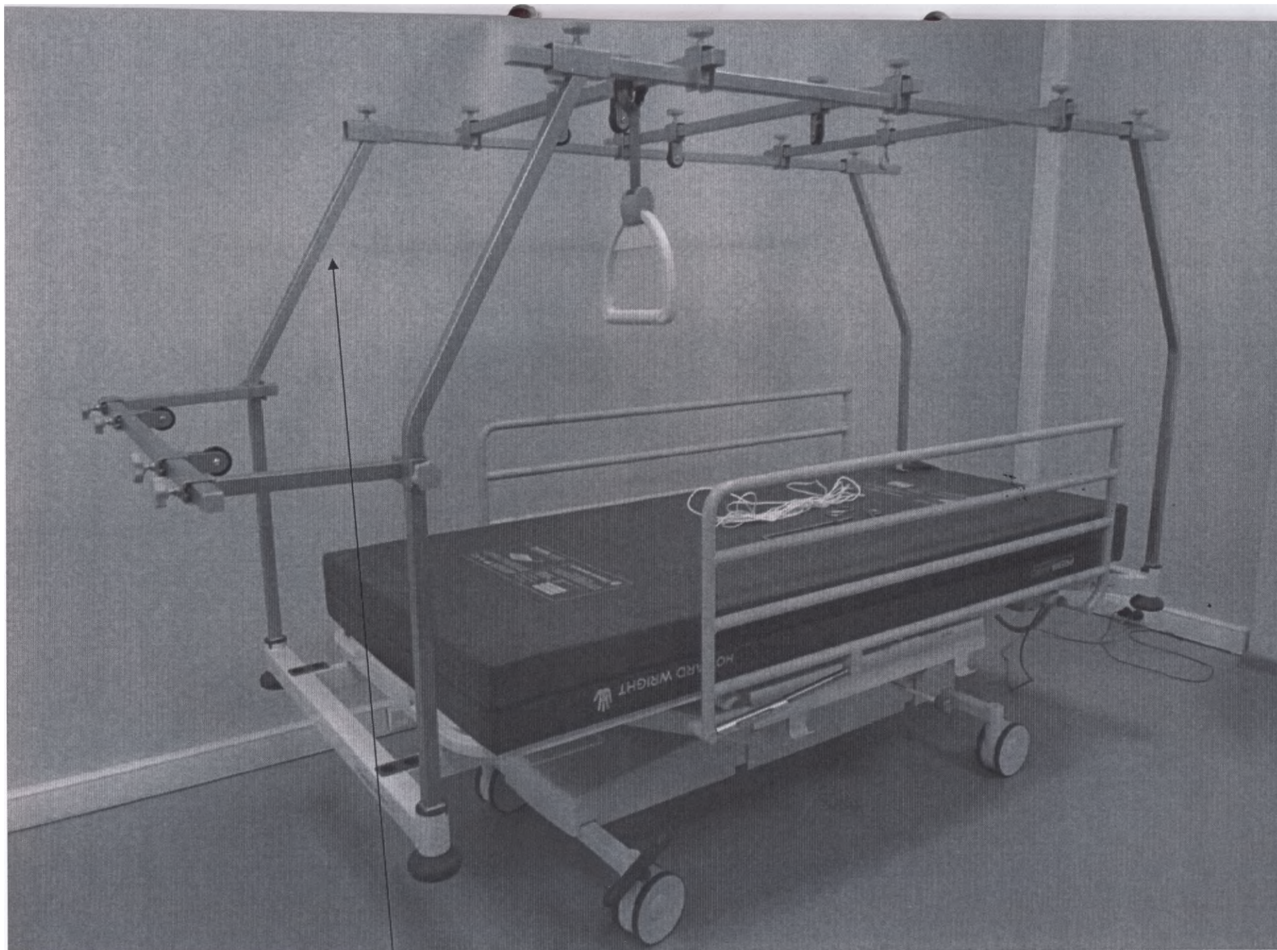
Ортопедическая рама (Orthopaedic frame)
