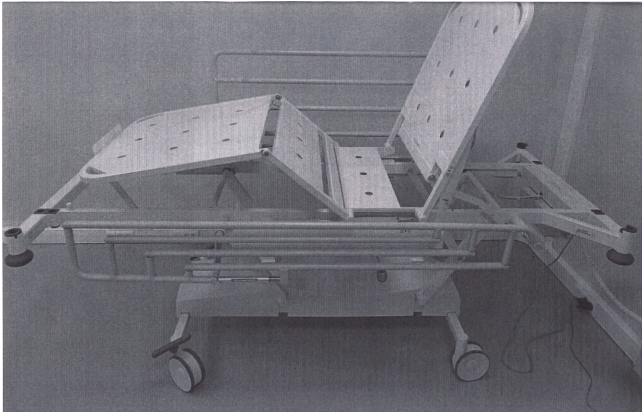
Кровать М9 общебольничная с горизонтальными боковыми ограждениями (M9 Ward Bed (Horizontal Siderails)), общий вид, без матраца
