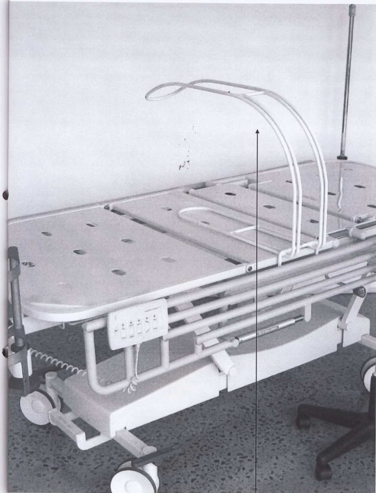
Держатель для одеяла (Blanket cradle)
