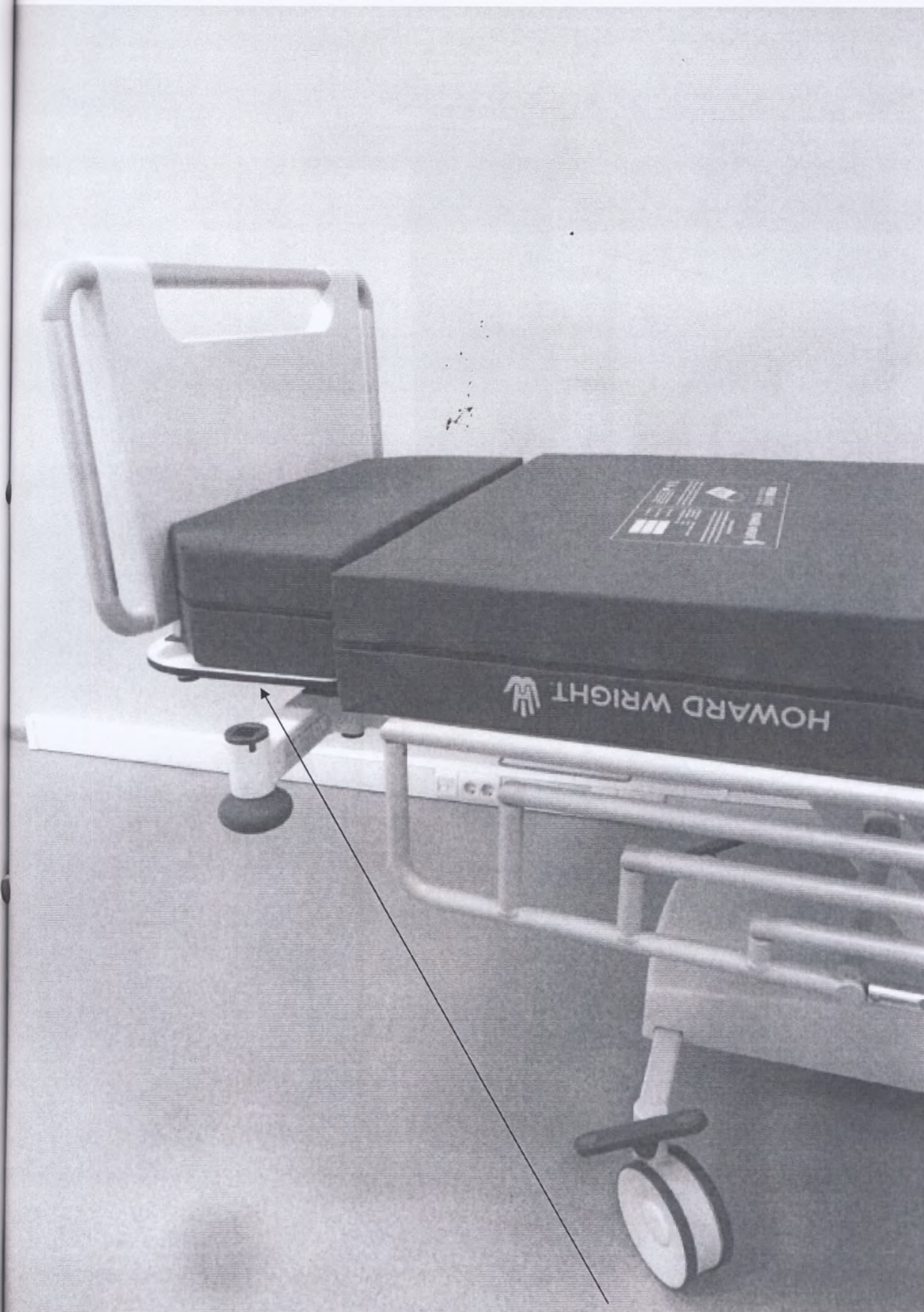
Дополнительный матрац для удлинения кровати M9 Ward (Bolster mattress for M9 Ward)
