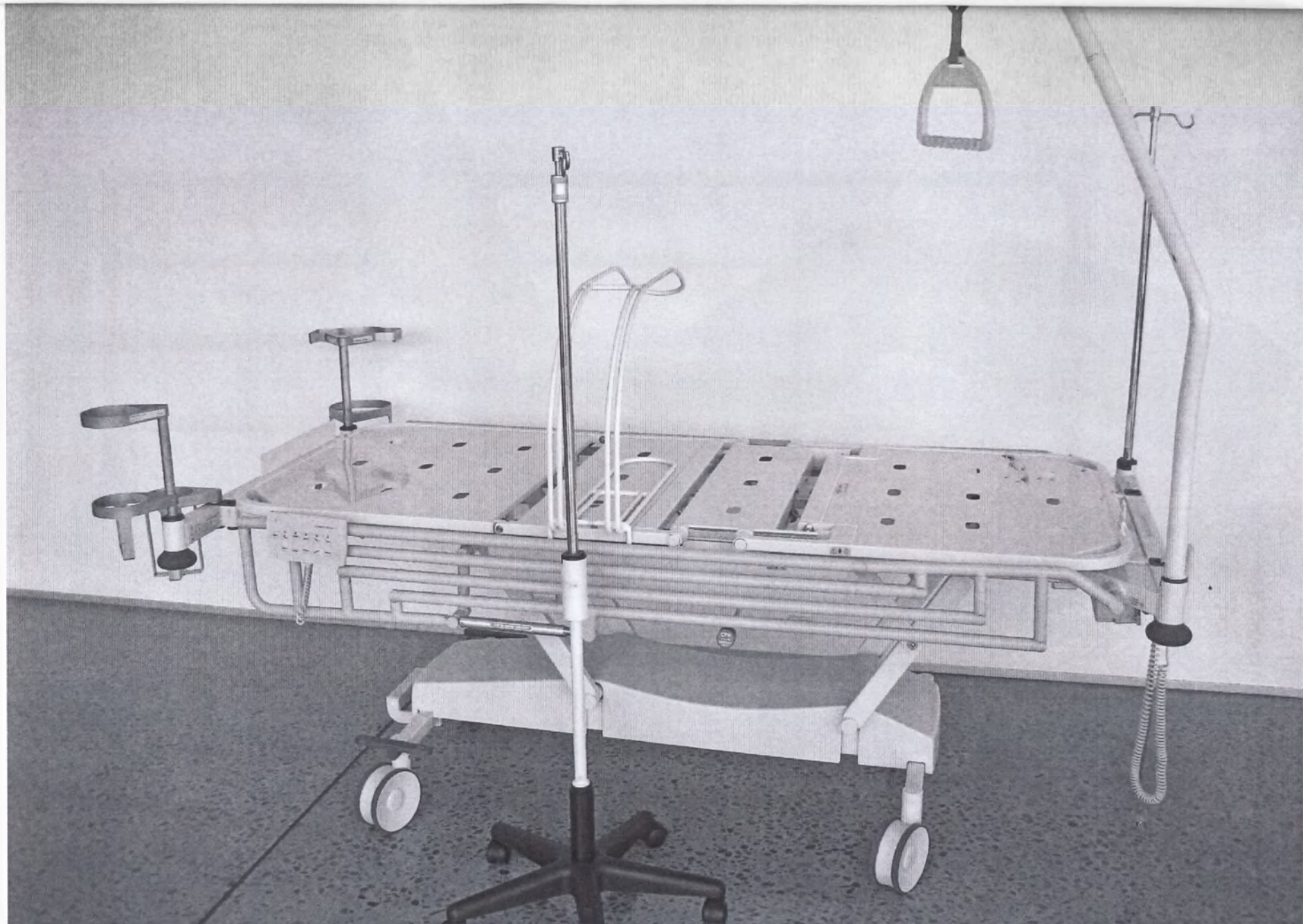
Кровать М9 общепольничная с горизонтальными боковыми ограждениями (M9 Ward Bed (Horizontal Siderails)) с принадлежностями, общий вид.
