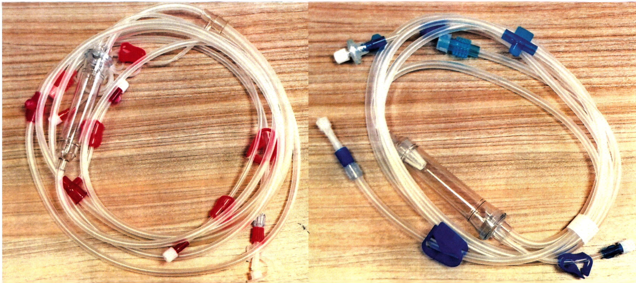
Комплект трубок для гемодиализа, BLU001E.
