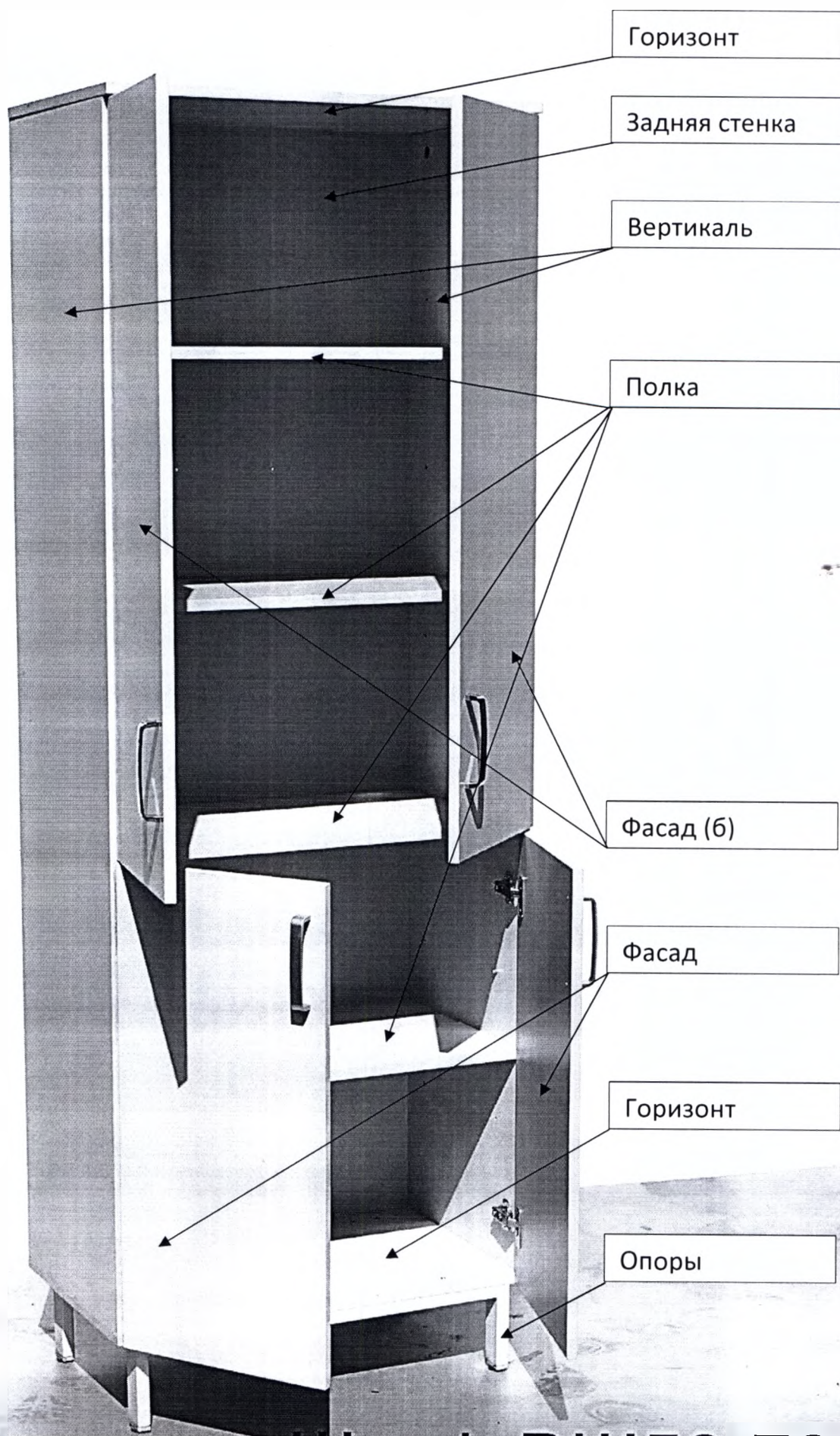
Шкаф ВШ56-70.1
