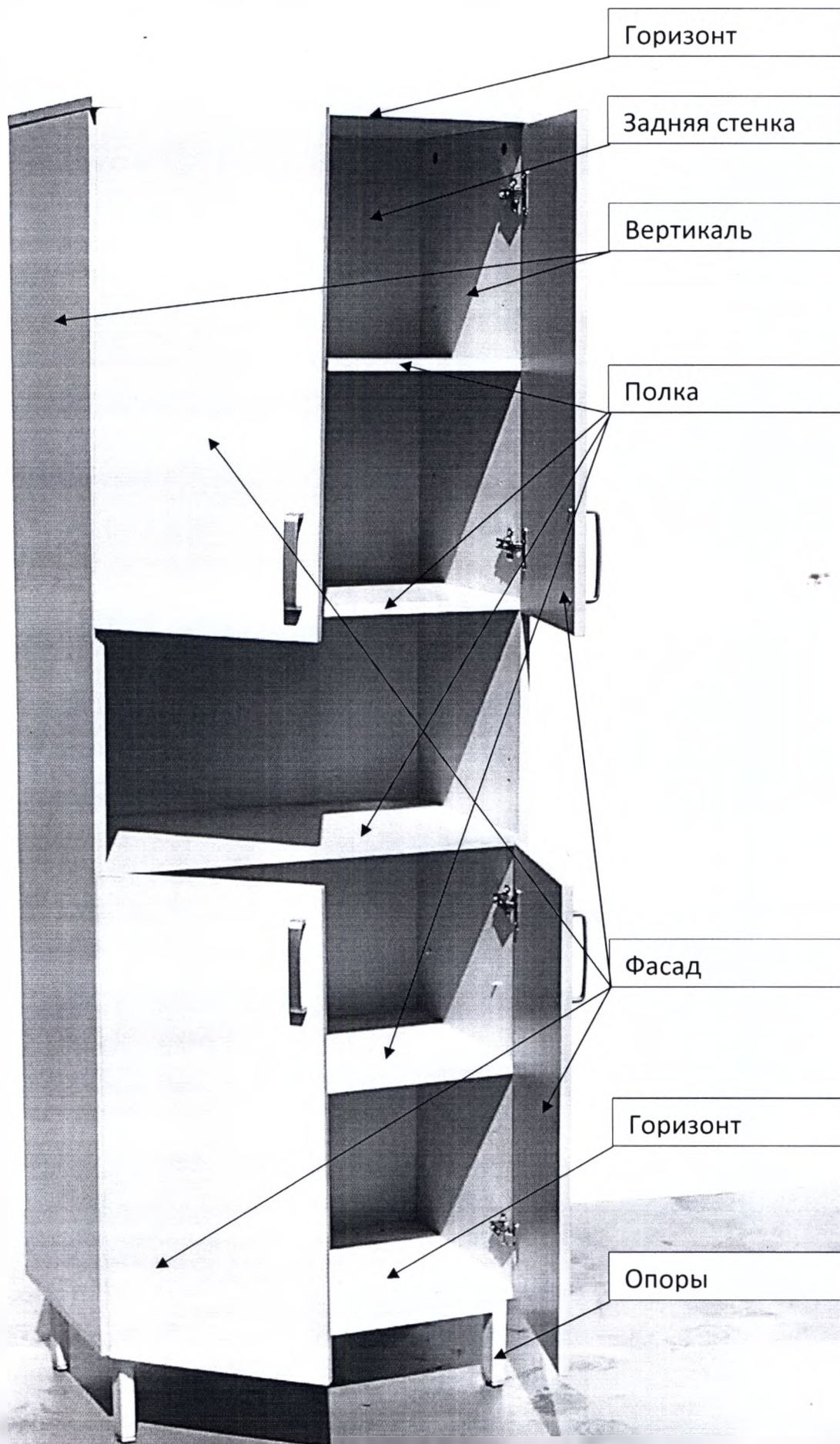
Шкаф ВШ55-70
