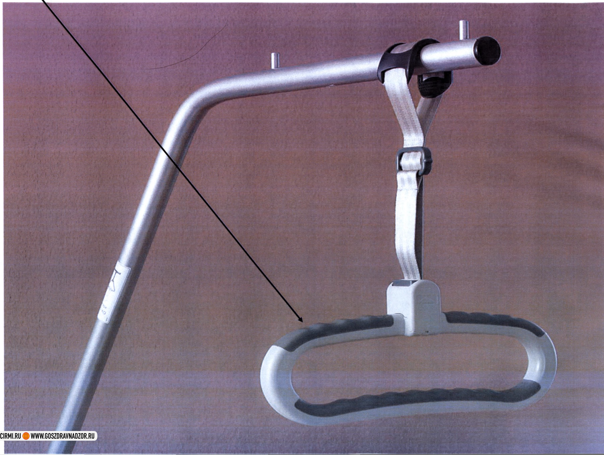
33. Рукоятка устройства для приподнятия пациента (Softtouch grab handle for patient lifting pole).
