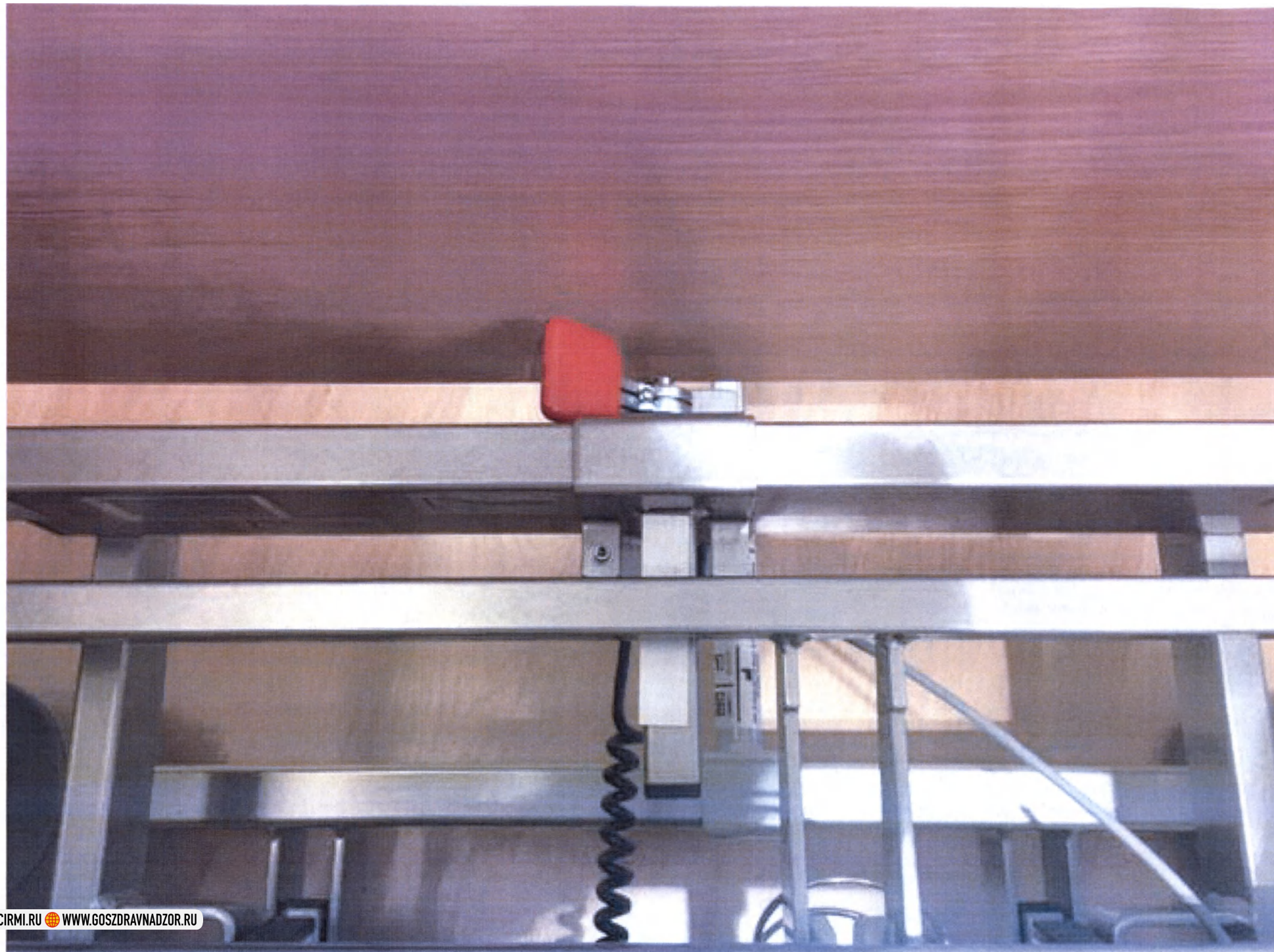
28. Устройство для экстренного опускания спинной секции (CPR on back section)
