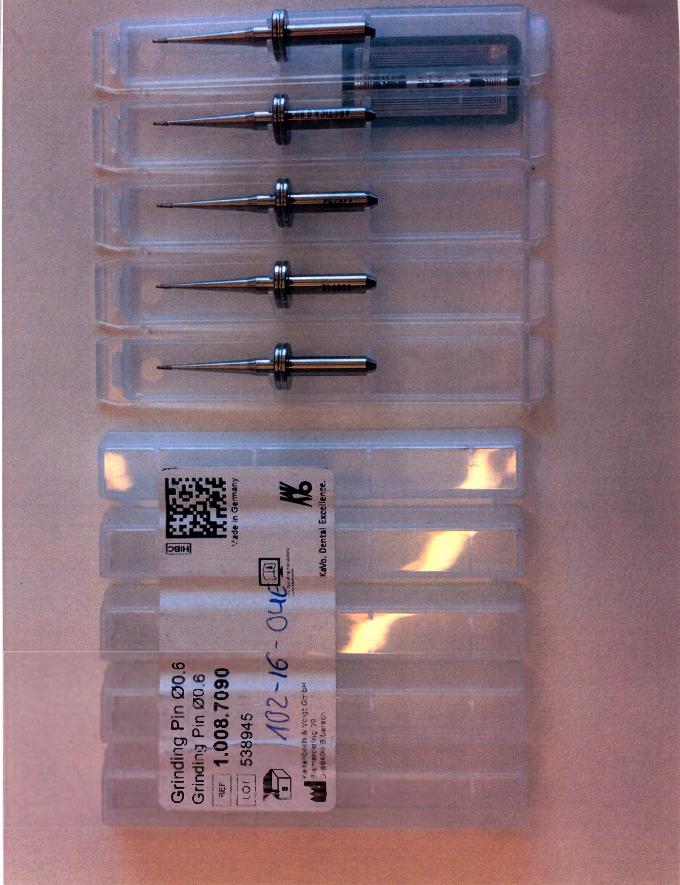
Фото 14 – Шлифовальные фрезы для заготовок из стеклокерамики KaVo ARCTICA Grinding Pin: Фреза диаметр 0,6 мм, 5 шт.
