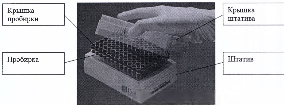
Общий вид изделия вместе со штативом.
