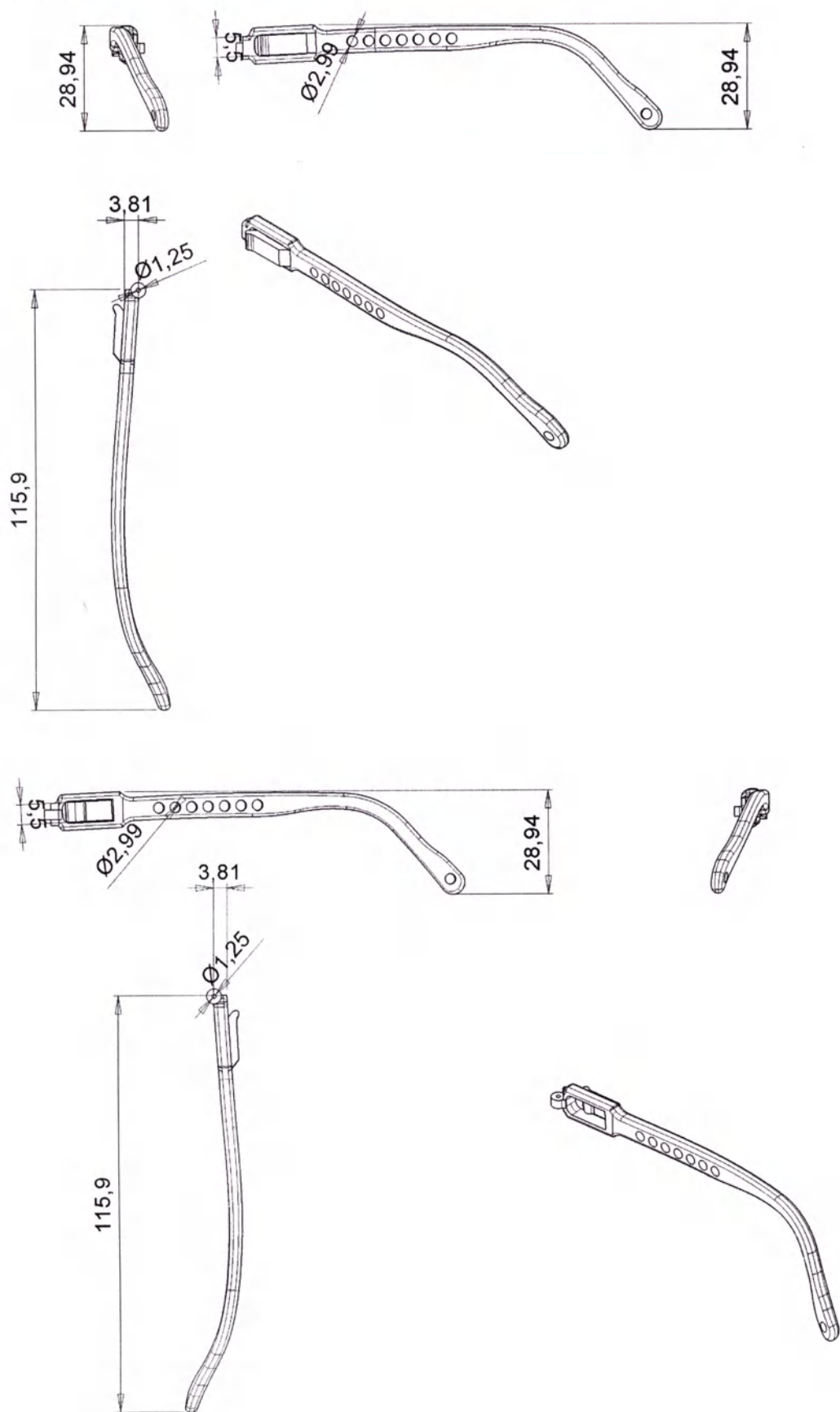
Рис. 5. Эскиз Заушины оправы
