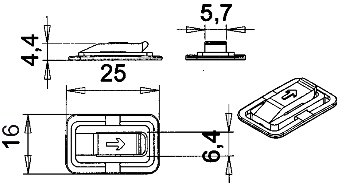
Рис. 6. Эскиз Крепление на оправу очков (клипон)
