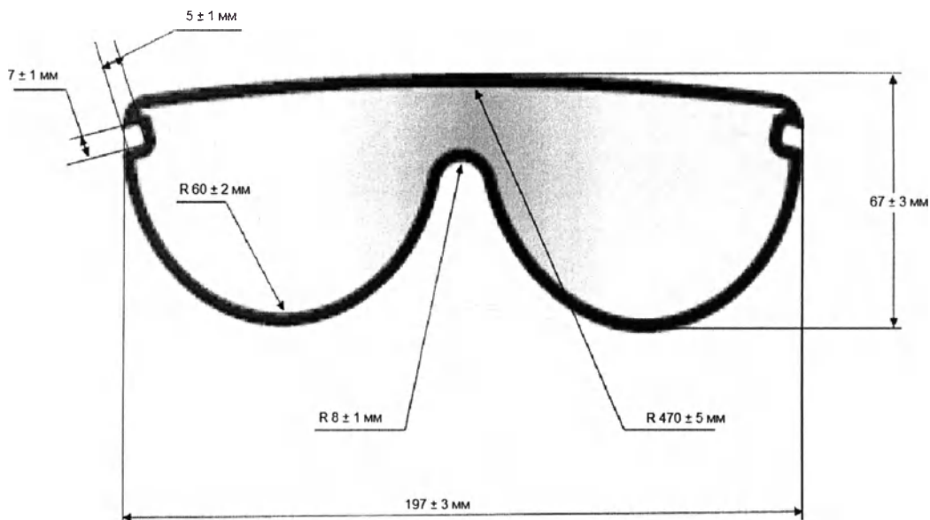
Рис. 3. Эскиз Щиток для глаз
