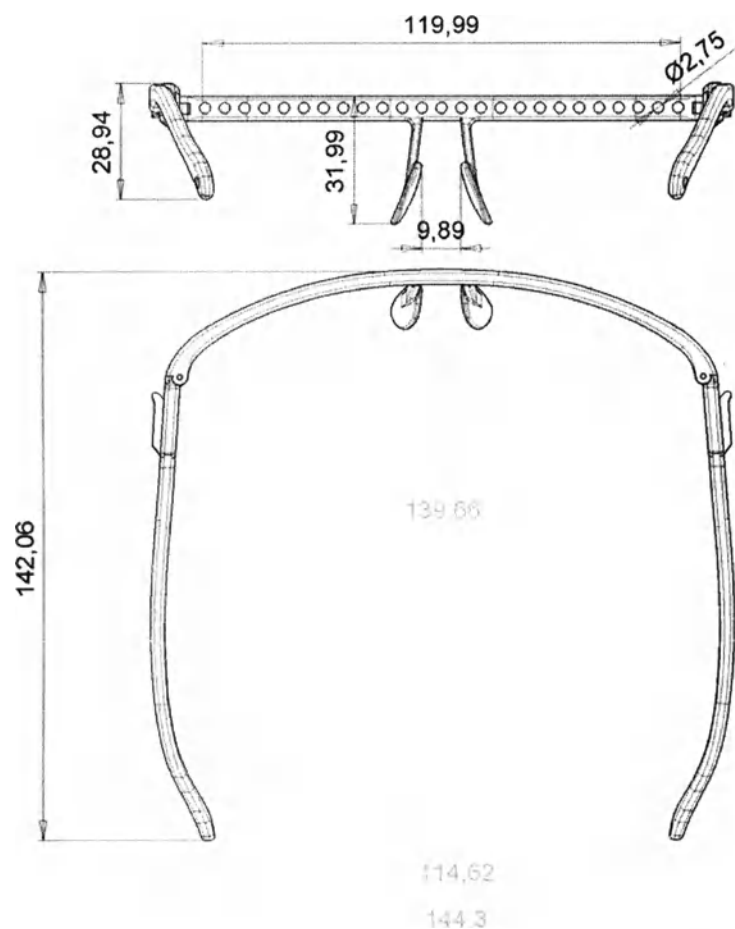
Рис. 4. Эскиз Оправа
