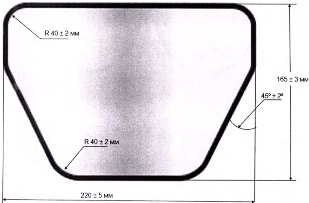
Рис. 2. Эскиз Щиток для лица типа Л
