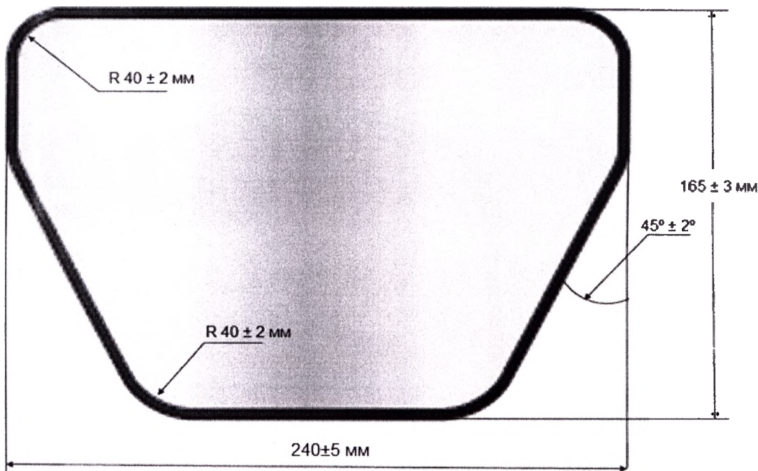
Рис. 2. Эскиз Щиток для лица типа Л
