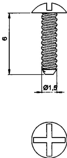
Рис. 7. Эскиз Винт самонарезающей
