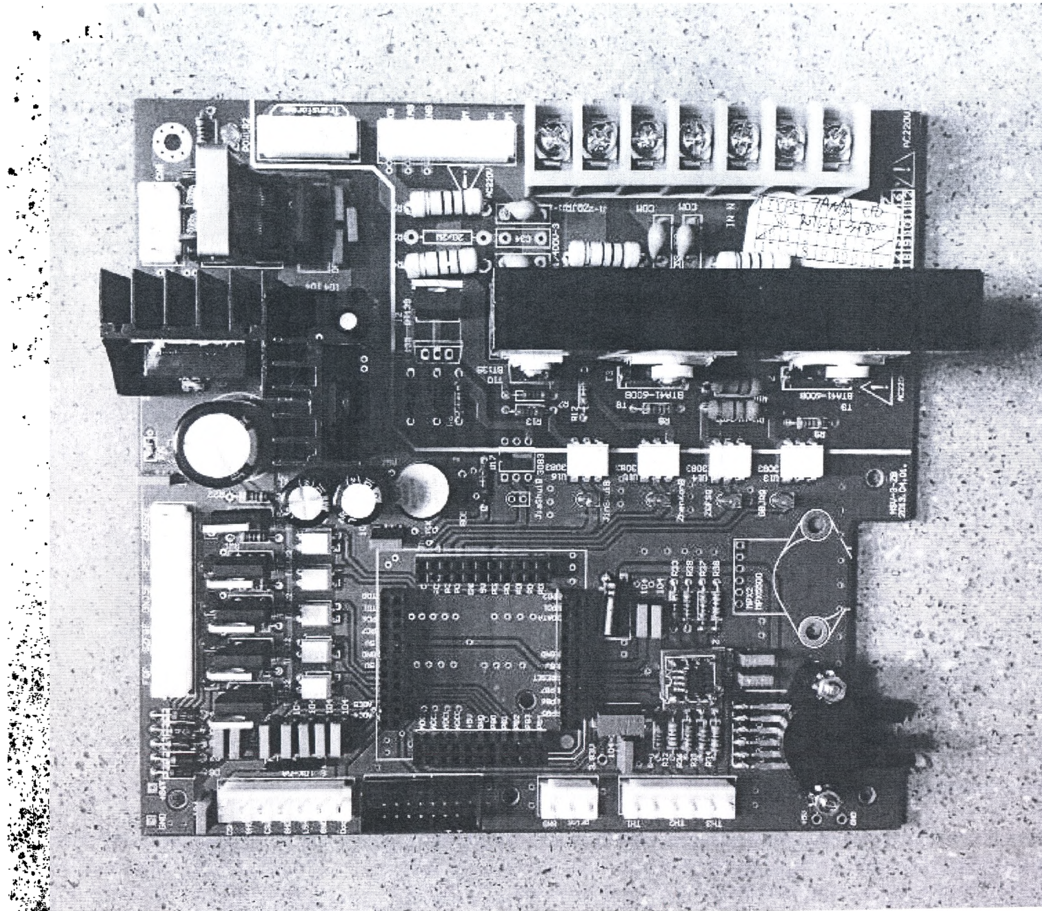
Плата управления.
