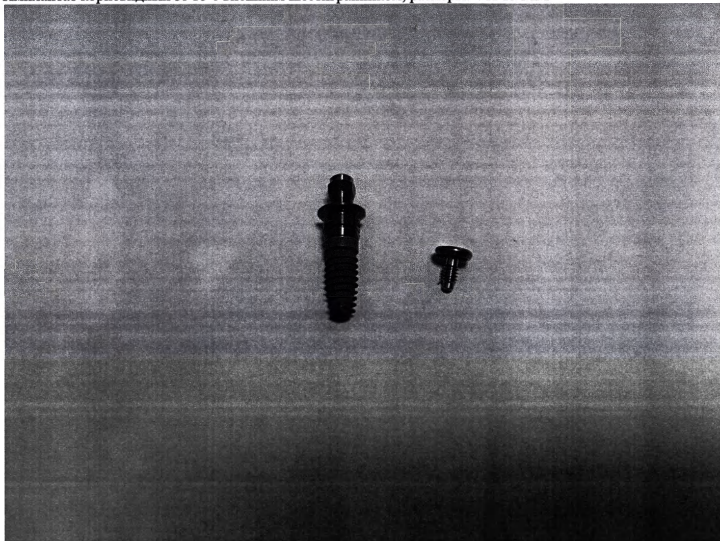
Имплантат корневидный 3i T3 с внешним шестигранником, размеры: 4 X 15 ММ
