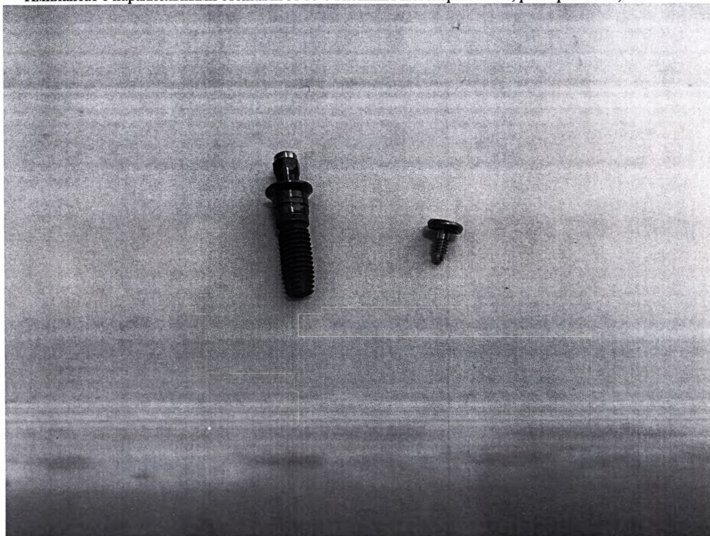
Имплантат с параллельными стенками ZrTi с внешним шестигранником, размеры: 6 X 8,5 ММ
