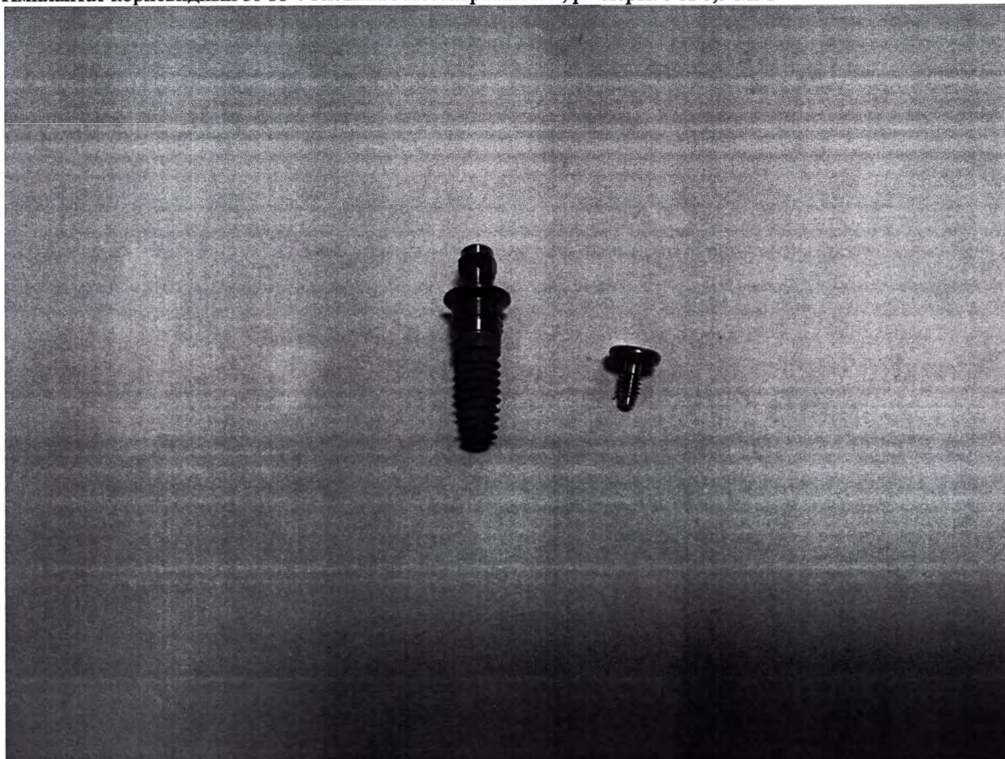
Имплантат корневидный 3i T3 с внешним шестигранником, размеры: 5 X 8,5 MM
