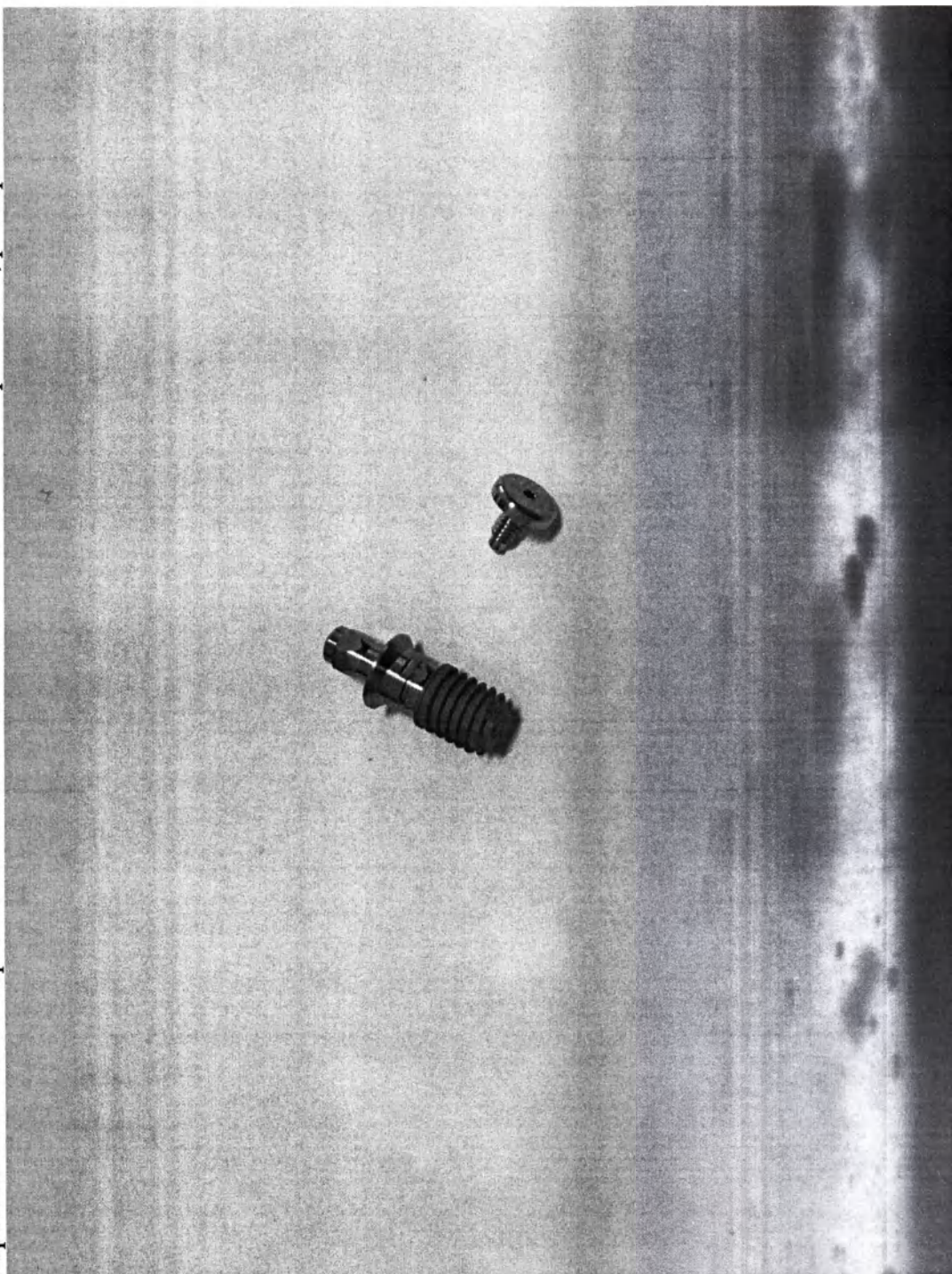
14. Короткий имплантат с параллельными стенками 3i T3 с внешним шестигранником, размеры: 5 ММ X 5 ММ
