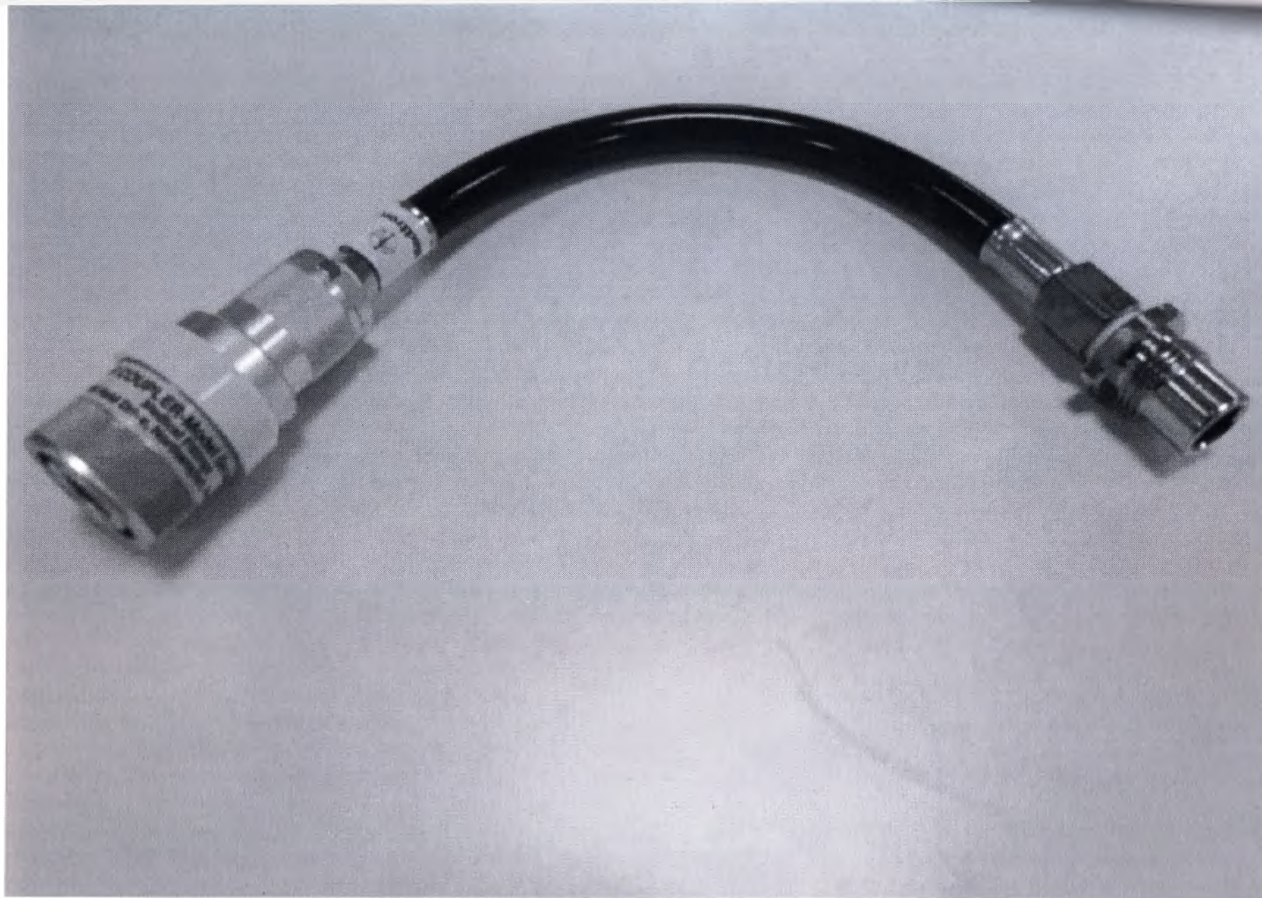
Внешний вид - Адаптеры для крепления шланга Midas Rex, модель: PC140
