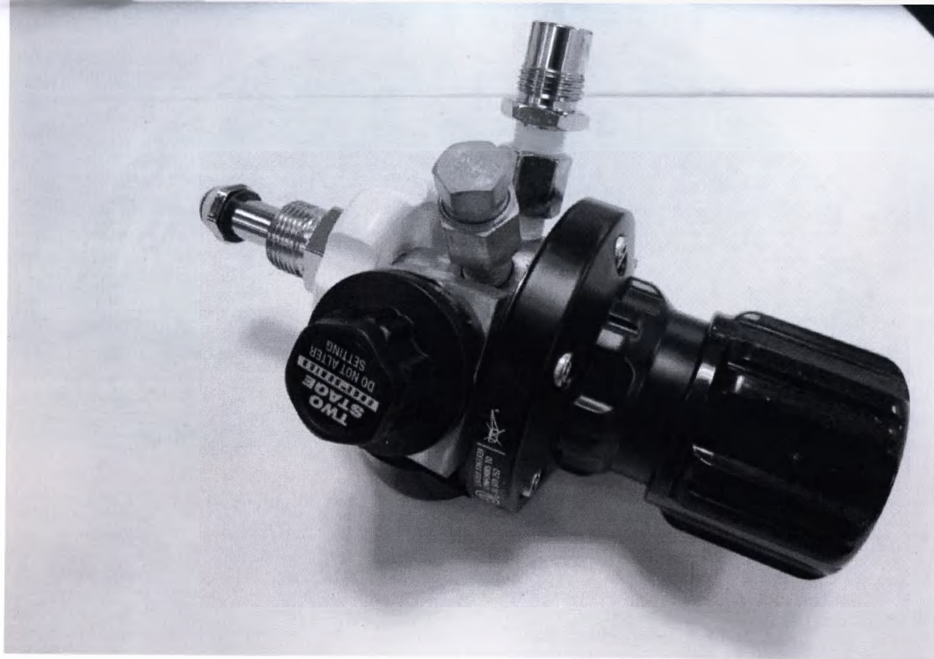
Внешний вид - Регулятор давления воздуха Midas Rex, модель: PA200
