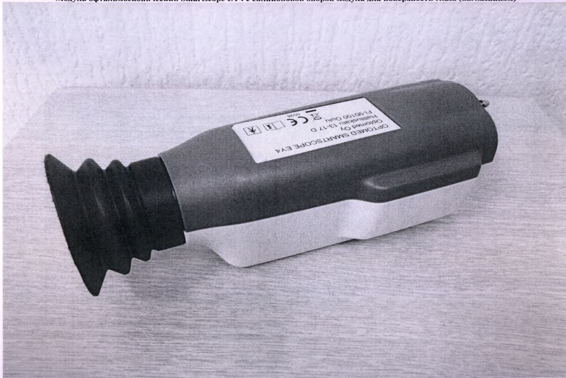
Модуль офтальмоскопический Smartscope EY4 с силиконовой опорой модуля для поверхности глаза (наглазником)
