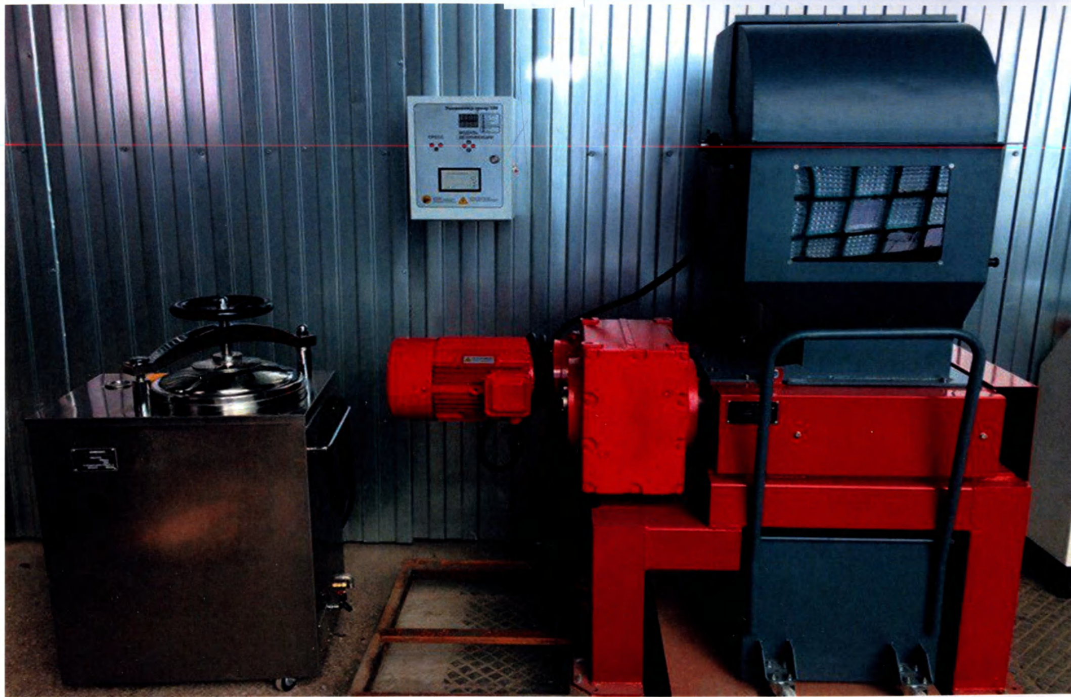
ЭЛЕКТРОННАЯ КОПИЯ ОФОРМЛЕНА ЦЕНТРОМ ИСПЫТАНИЙ И РЕГИСТРАЦИИ МЕДИЦИНСКИХ ИЗДЕЛИЙ Установка для обезвреживания и измельчения медицинских отходов «ЭЛИМИНАТОР-СУПЕР», исполнение ЭЛИМИНАТОР-СУПЕР100
